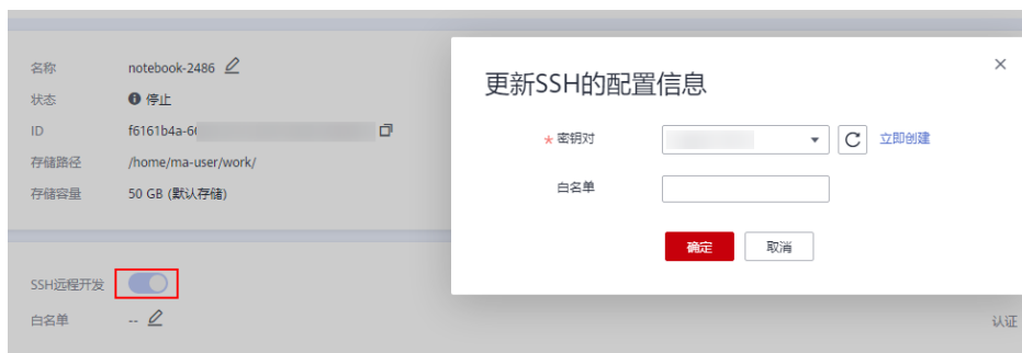
图 3-13 更新 SSH 配置信息
