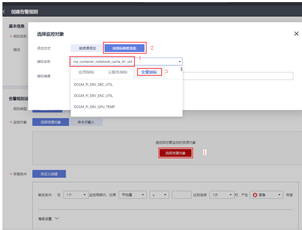
图 3-19 监控对象指标设置
