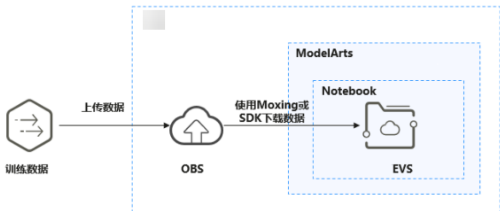
图 5-60 数据通过 OBS 中转上传到 Notebook
