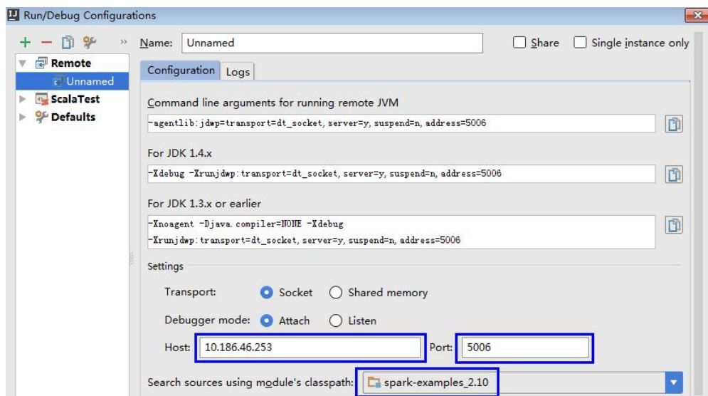
图 14-44 配置参数
