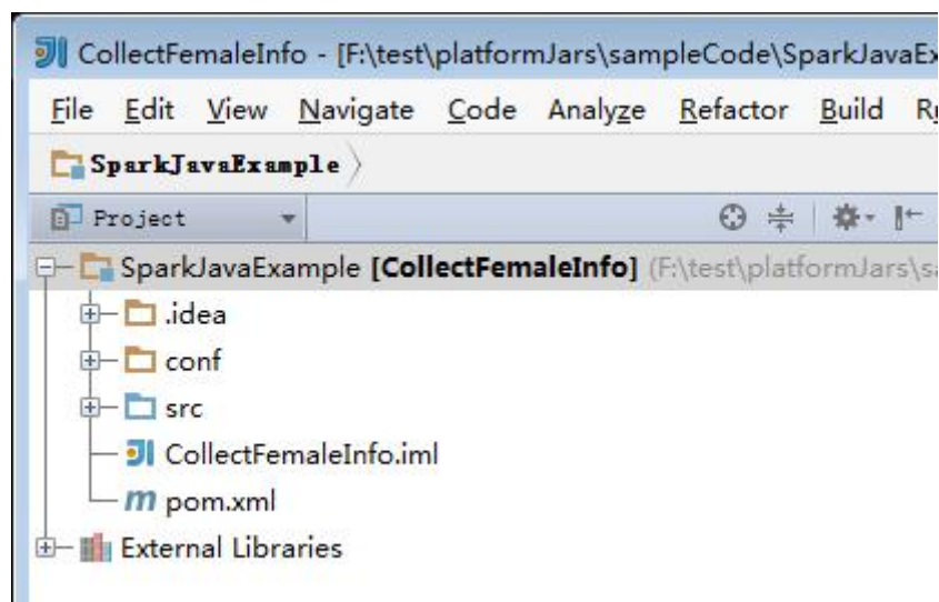
图 14-29 已导入工程
