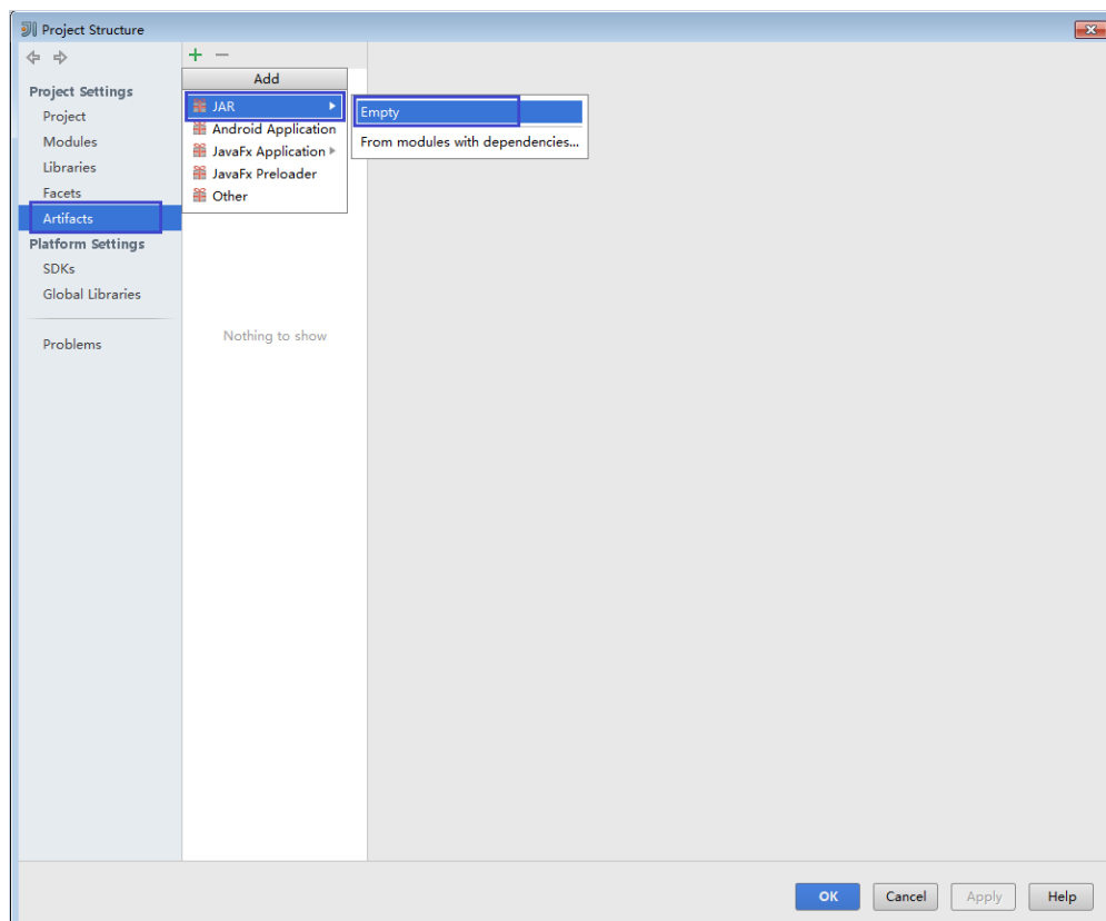
图 5-32 添加 Artifacts
