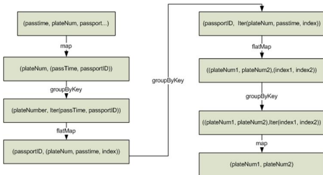
图 14-36 实现 1 逻辑
