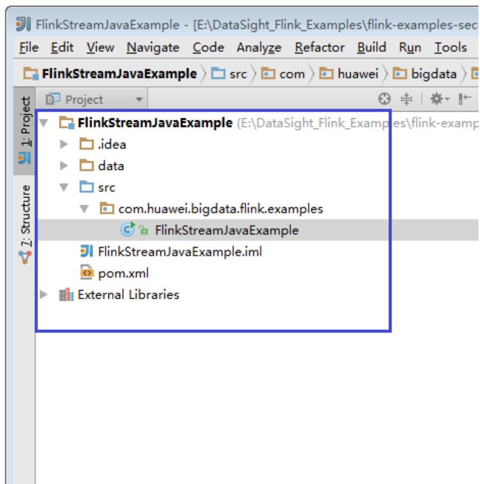
图 5-14 已导入工程
