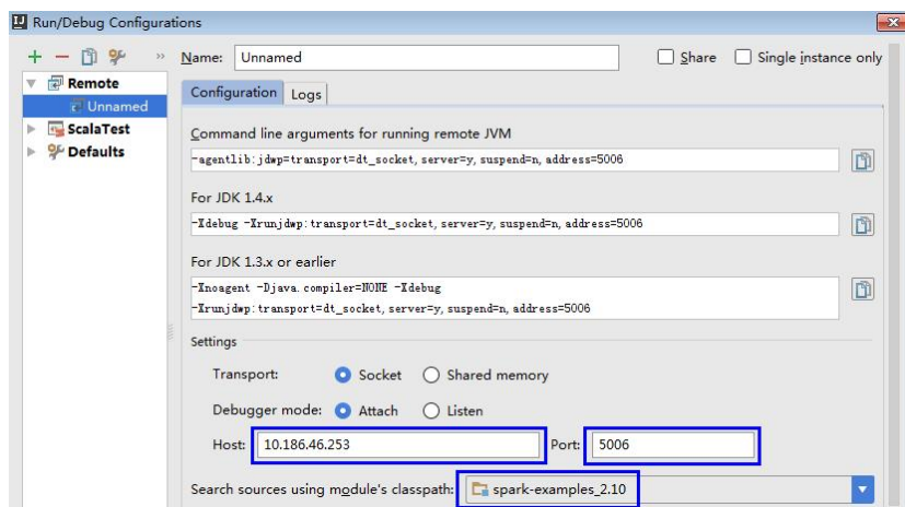
图 14-43 选择 Remote
