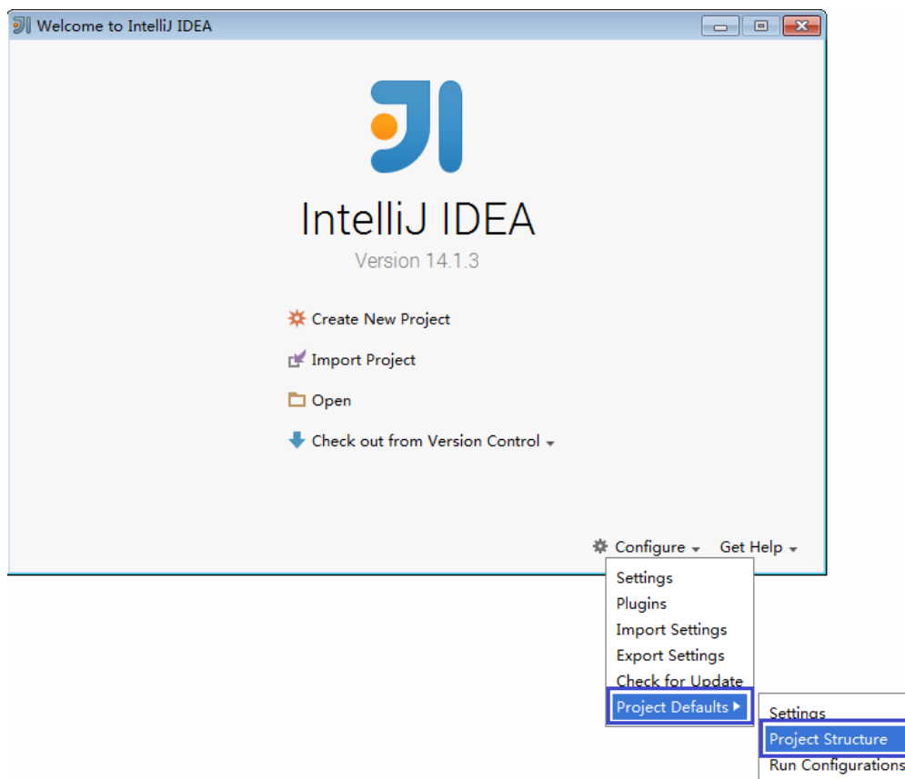
图 5-5 Project Defaults
