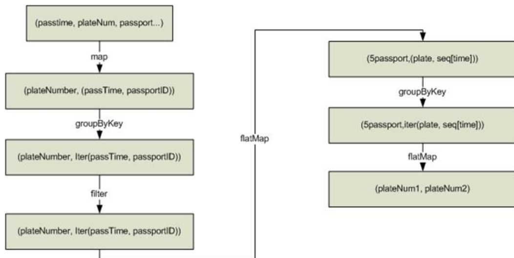
图 14-37 实现 2 逻辑
