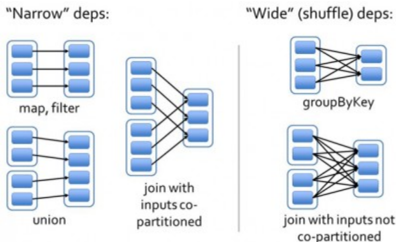
图 14-2 RDD 的依赖
