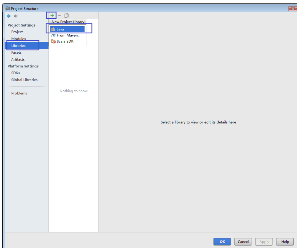
图 5-19 Add Java
