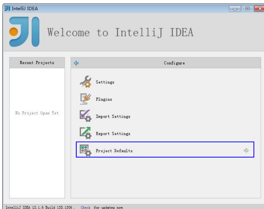
图 14-9 Configure
