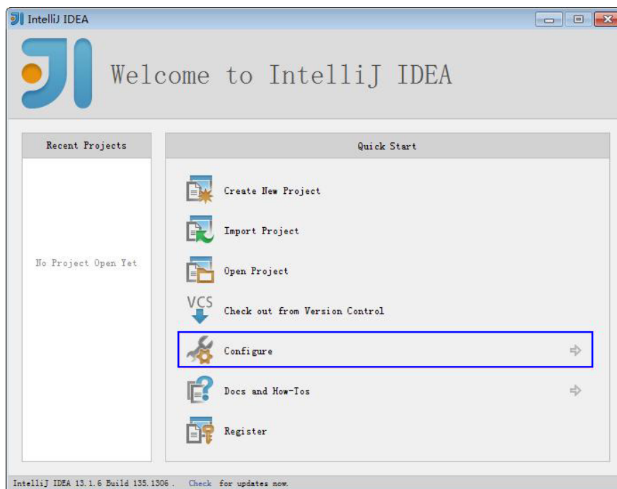
图 14-8 Quick Start
