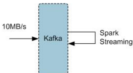
图 14-42 应用场景
