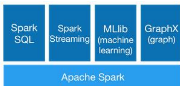
图 14-1 Spark 架构
