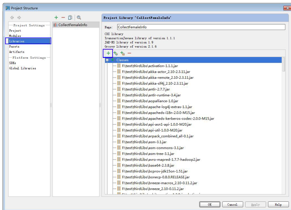
图 14-38 添加依赖包
