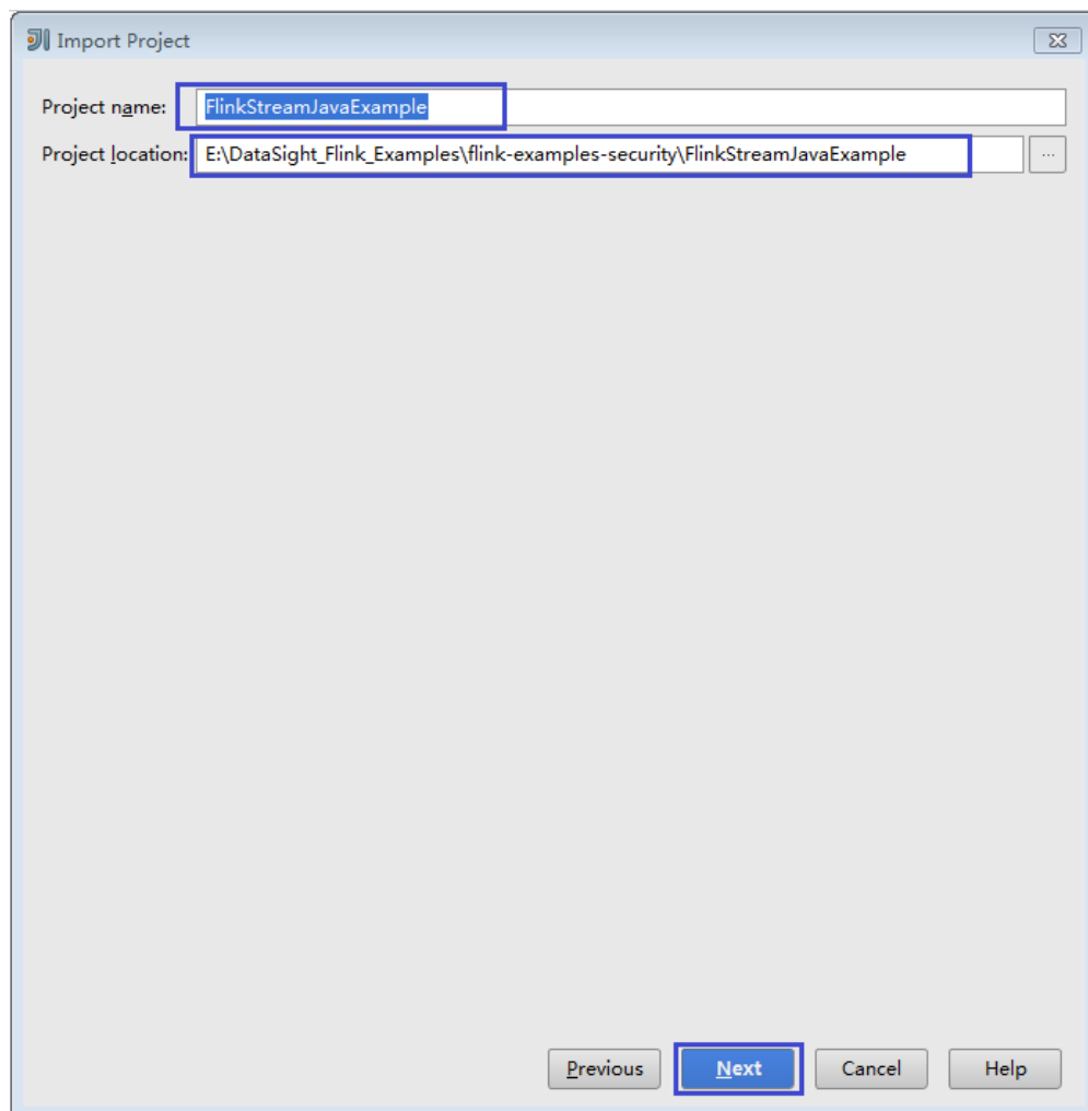
图 5-12 Import Project
