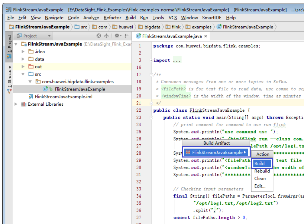
图 5-36 Build
