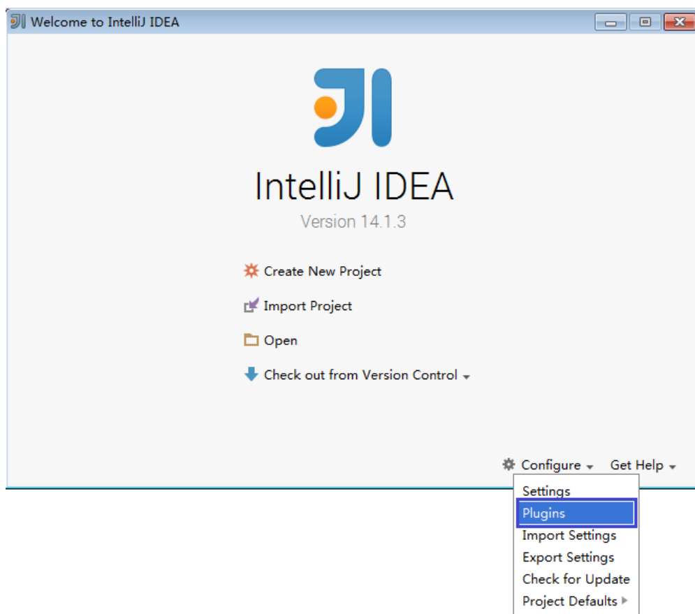
图 5-15 Plugins
