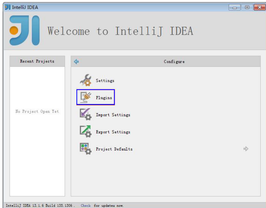
图 14-20 Plugins
