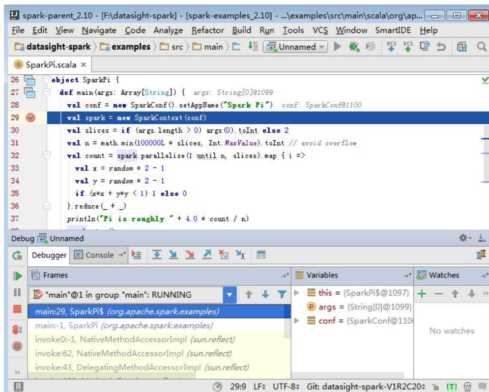
图 14-46 调试
