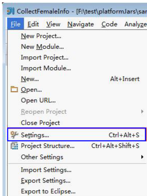
图 5-28 选择 Settings
