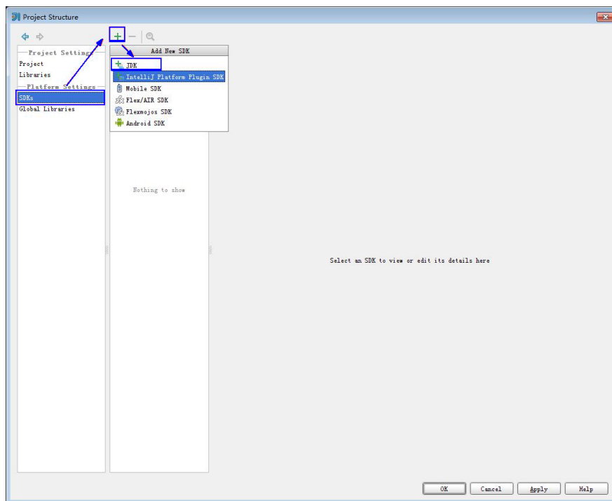
图 14-17 添加 JDK
