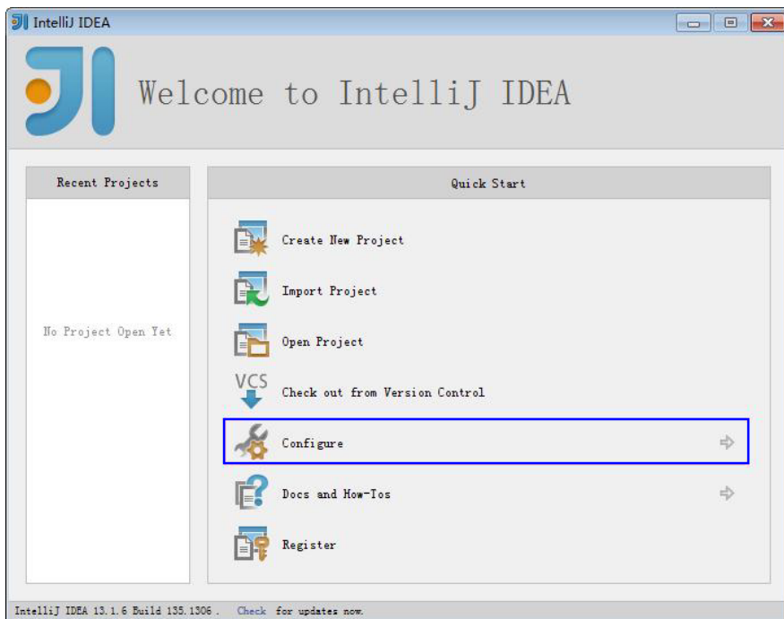
图 14-14 Quick Start
