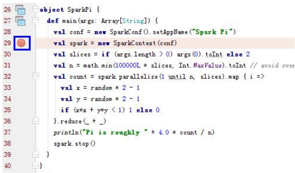
图 14-45 设置断点
