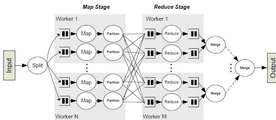
图 14-4 算法流程
