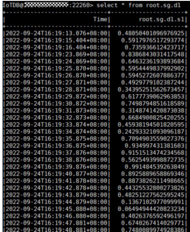
图 18-24 查看写入的数据内容
