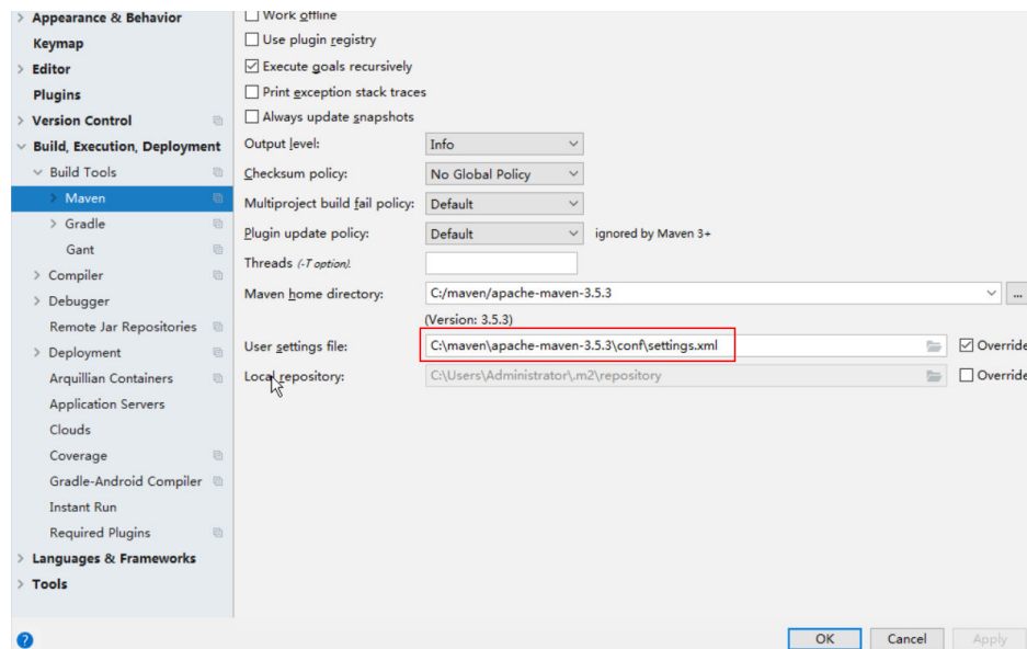
图 22-4 “settings.xml”文件放置目录
