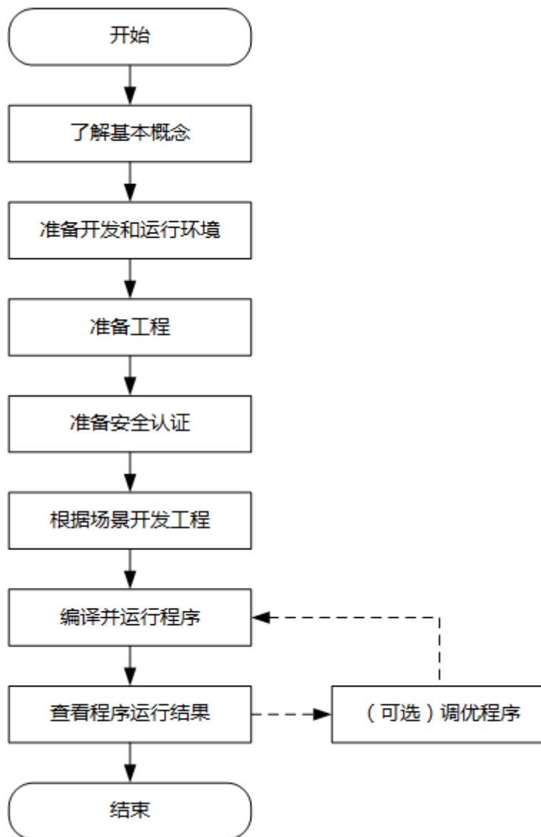
图 8-3 Flink 应用程序开发流程
