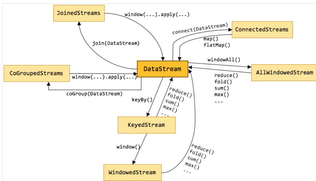
图 9-56 Flink Stream 的各种流类型转换
