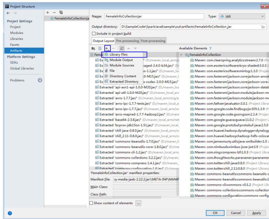
图 27-42 添加 Library Files
