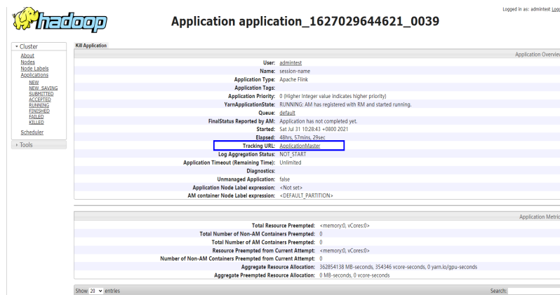
图 18-23 在 Yarn WebUI 查看作业信息
