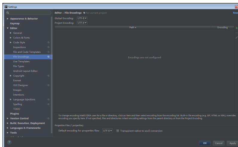
图 22-3 设置 IntelliJ IDEA 的编码格式
