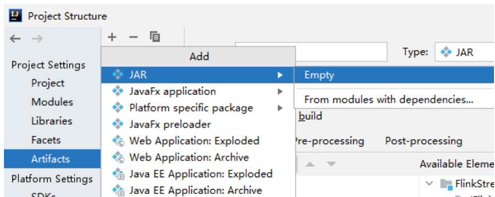
图 5-13 添加 Artifacts
