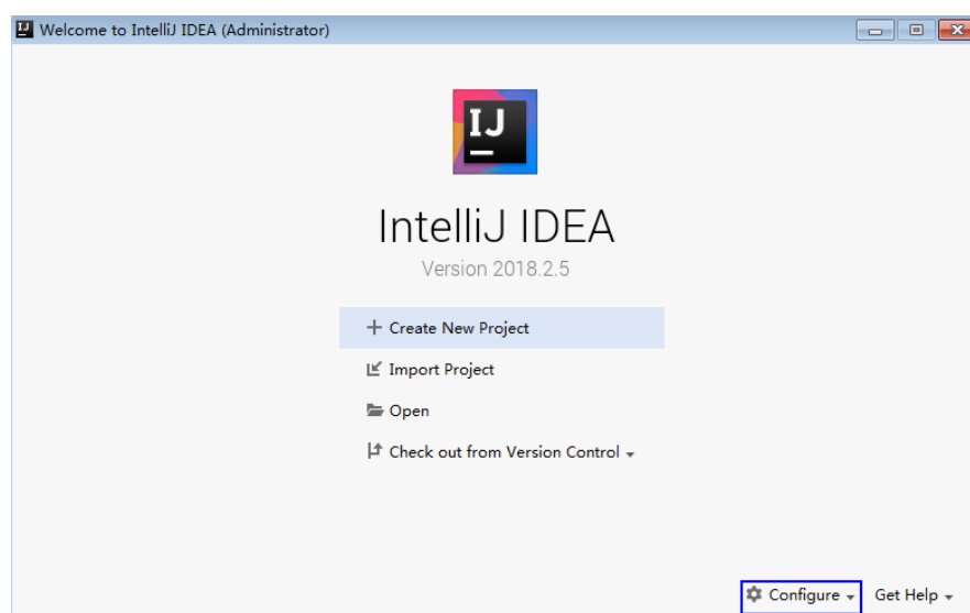
图 26-10 Quick Start
