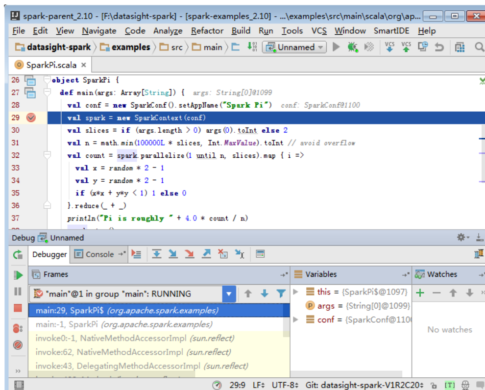
图 27-50 调试
