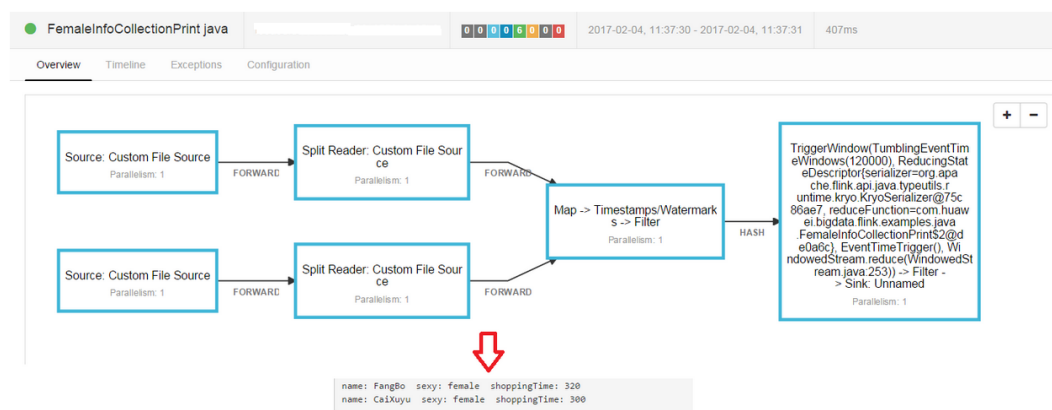
图 9-35 显示图
