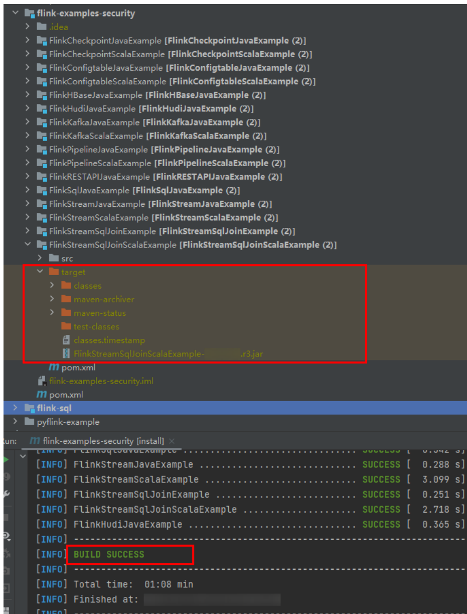
图 8-41 编译完成
