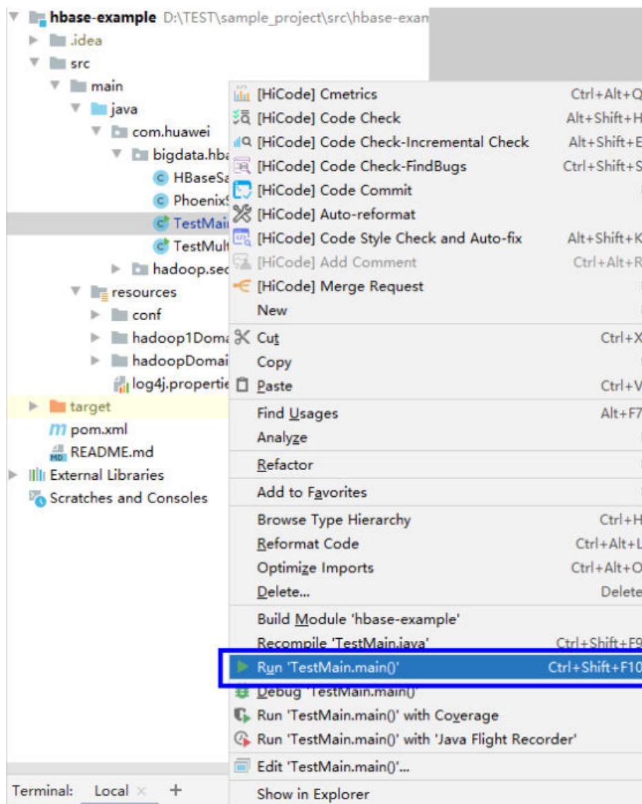
图 5-5 运行程序
