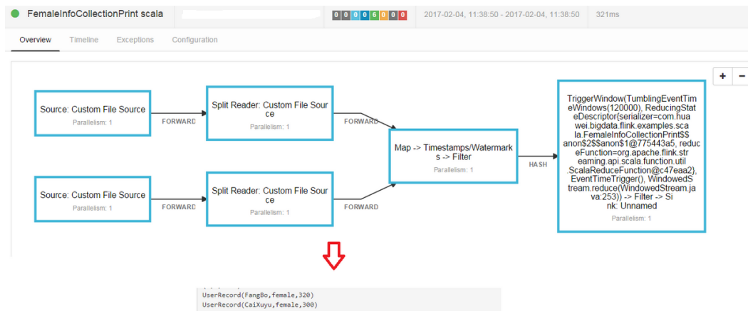
图 9-36 显示图
