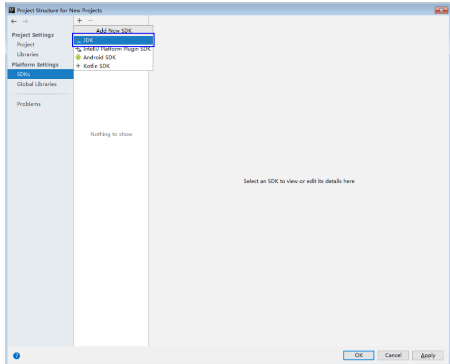
图 26-13 添加 JDK
