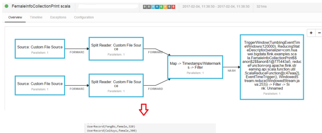
图 8-34 显示图
