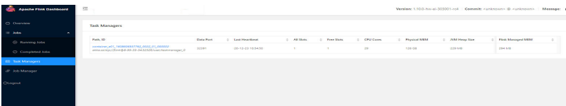
图 9-48 提交的任務
