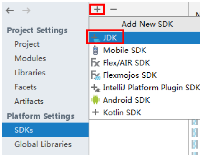
图 17-4 添加 JDK
