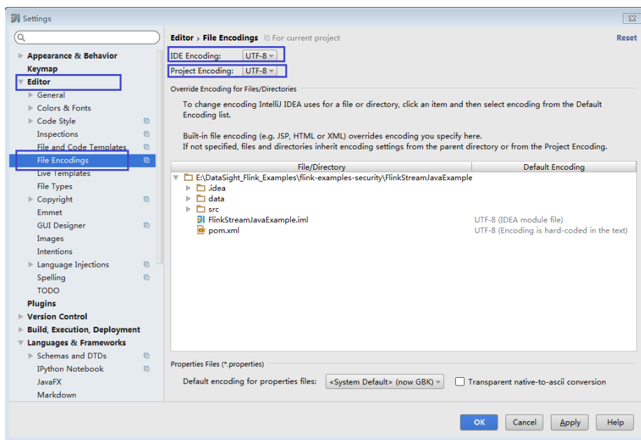
图 8-30 Settings
