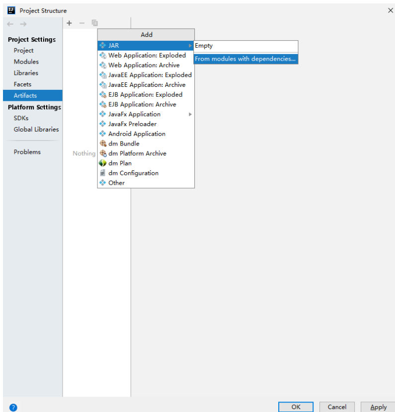
图 19-22 添加 Artifacts
