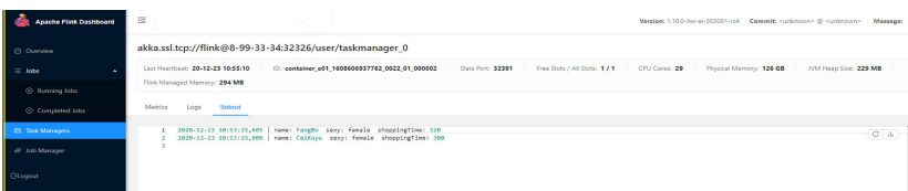
图 9-49 运行结果
