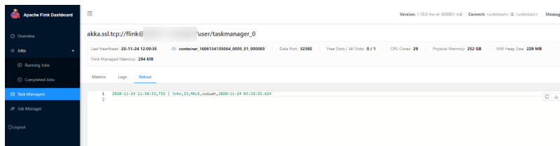
图 8-56 运行结果
