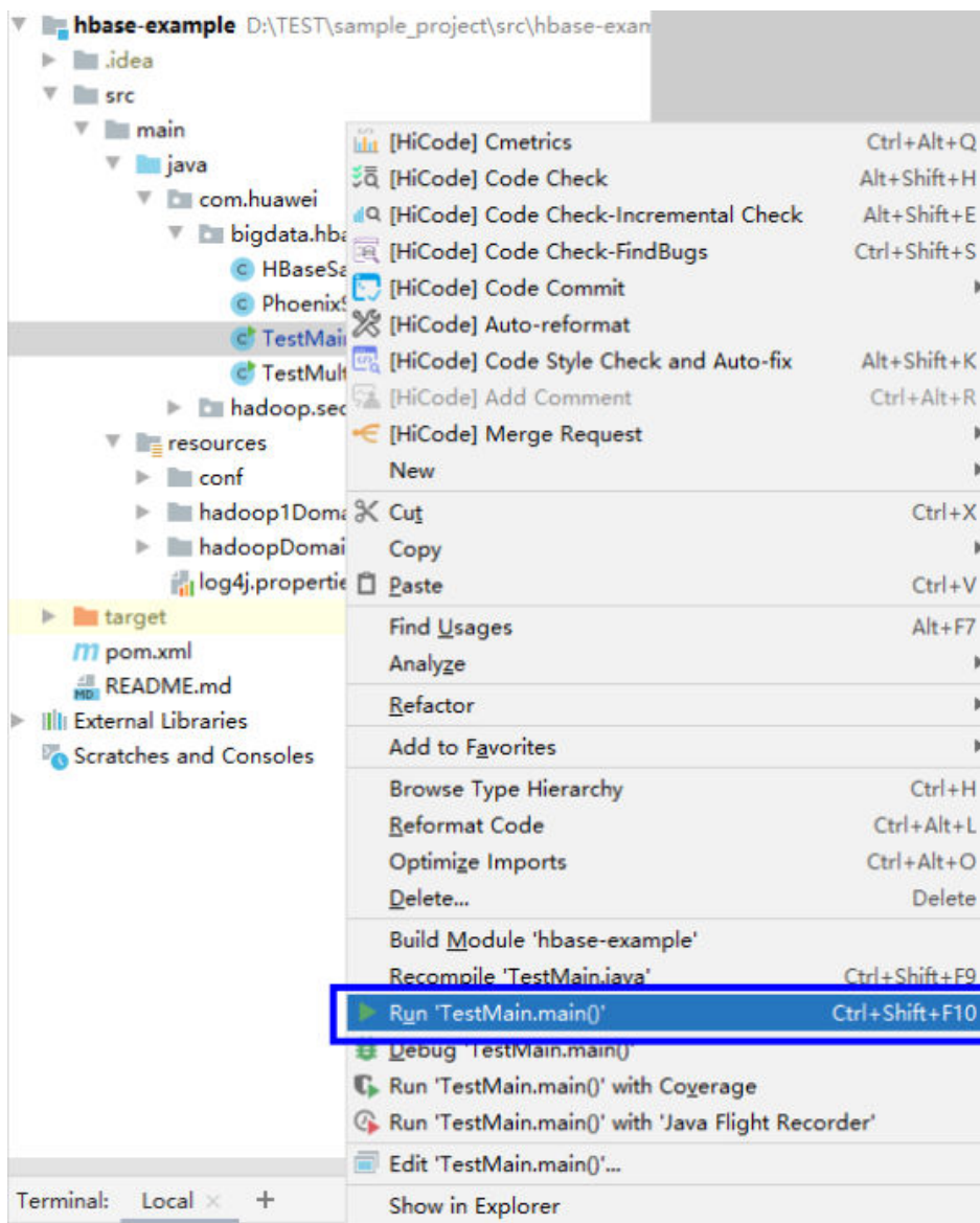
图 10-22 运行程序
