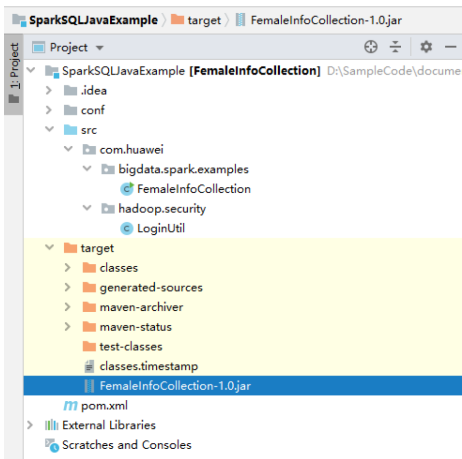
图 27-40 获取 jar 包
