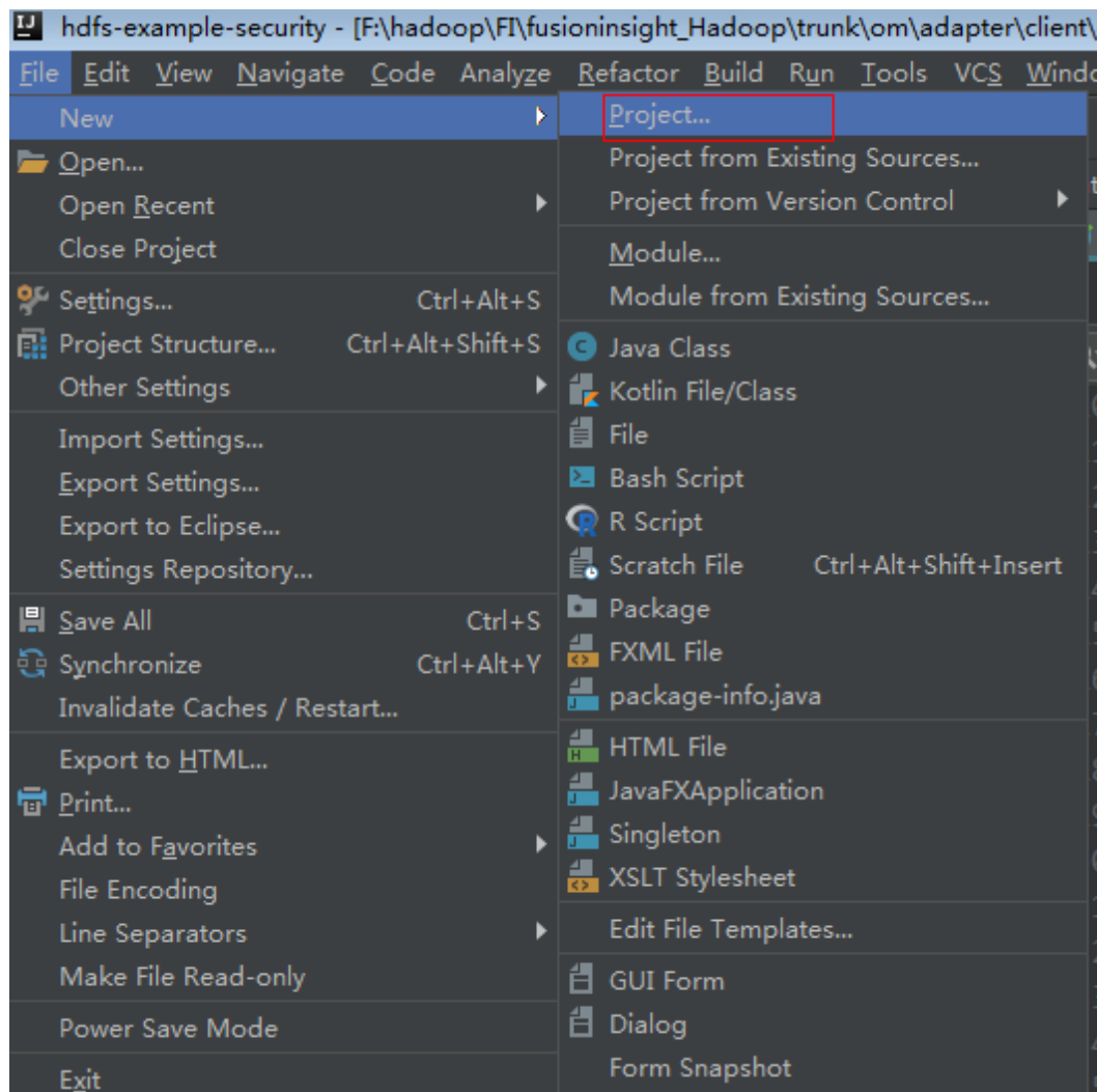
图 22-5 创建工程
