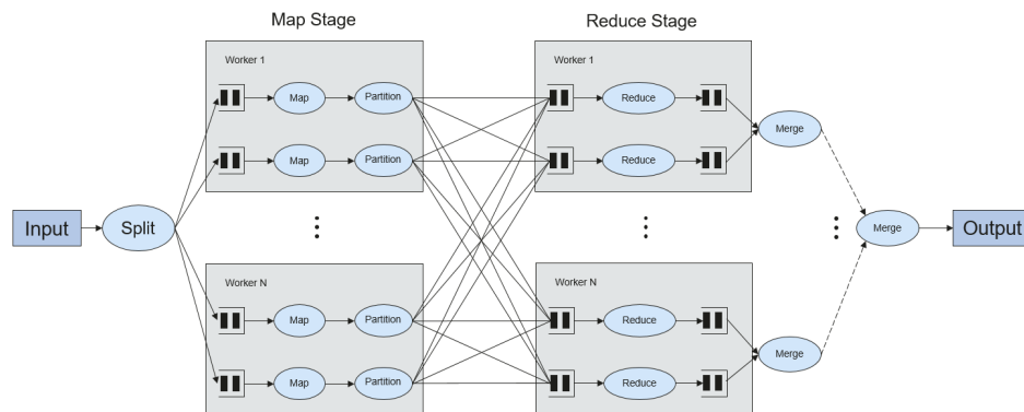
图 27-3 算法流程
