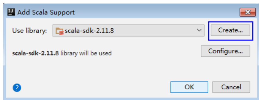
图 26-27 Create...
