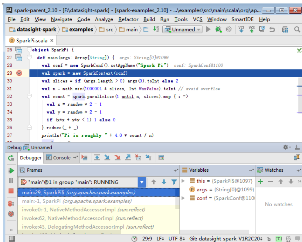
图 26-50 调试
