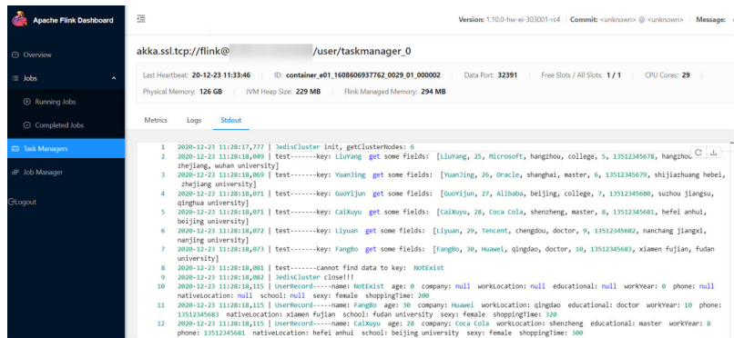
图 8-50 输出结果
