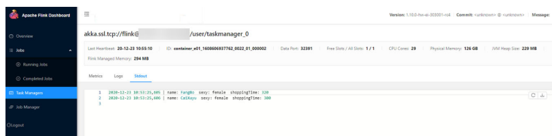
图 8-53 运行结果
