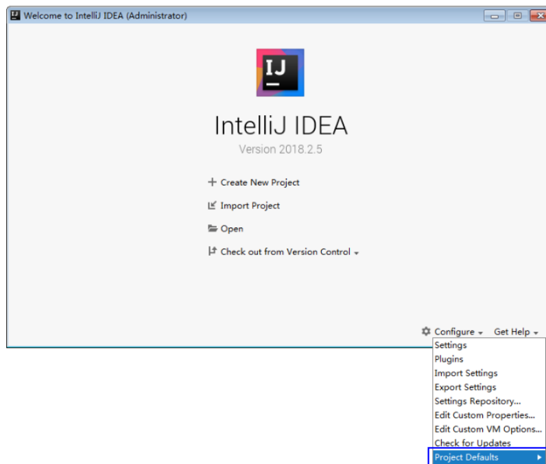
图 27-11 Configure
