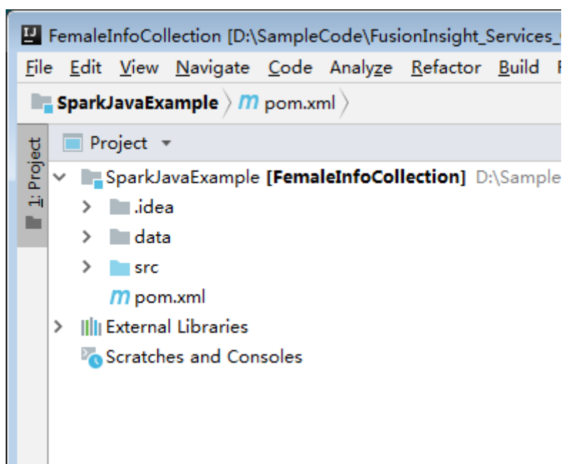
图 26-24 已导入工程
