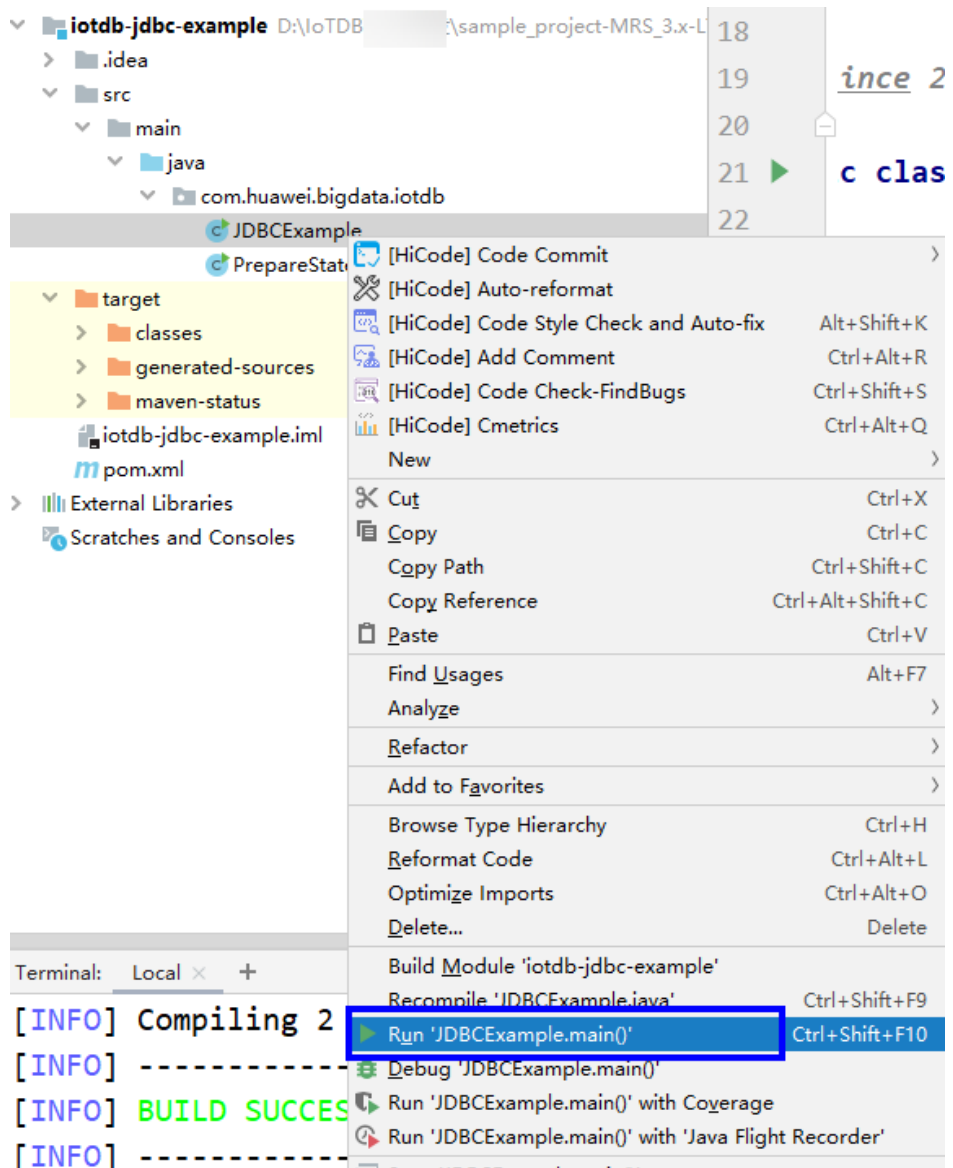
图 18-17 运行程序
