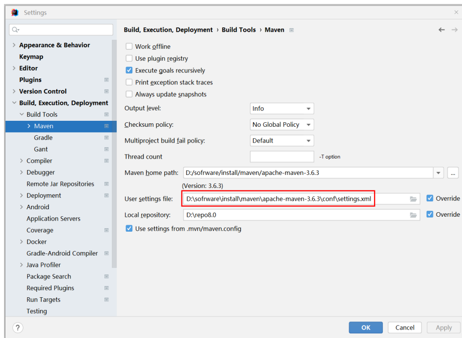
图 9-34 “settings.xml” 文件放置目录
