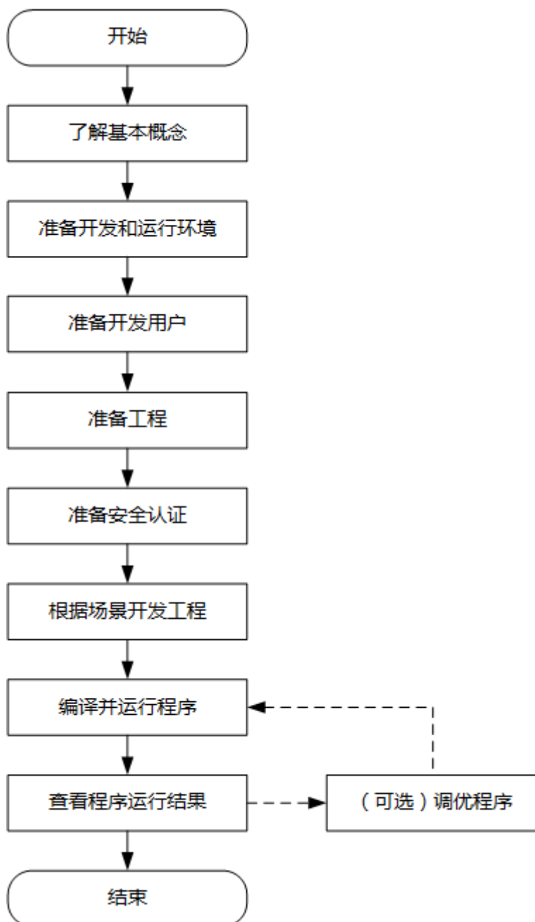
图 26-8 Spark 应用程序开发流程
