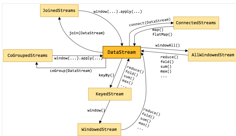
图 8-60 Flink Stream 的各种流类型转换
