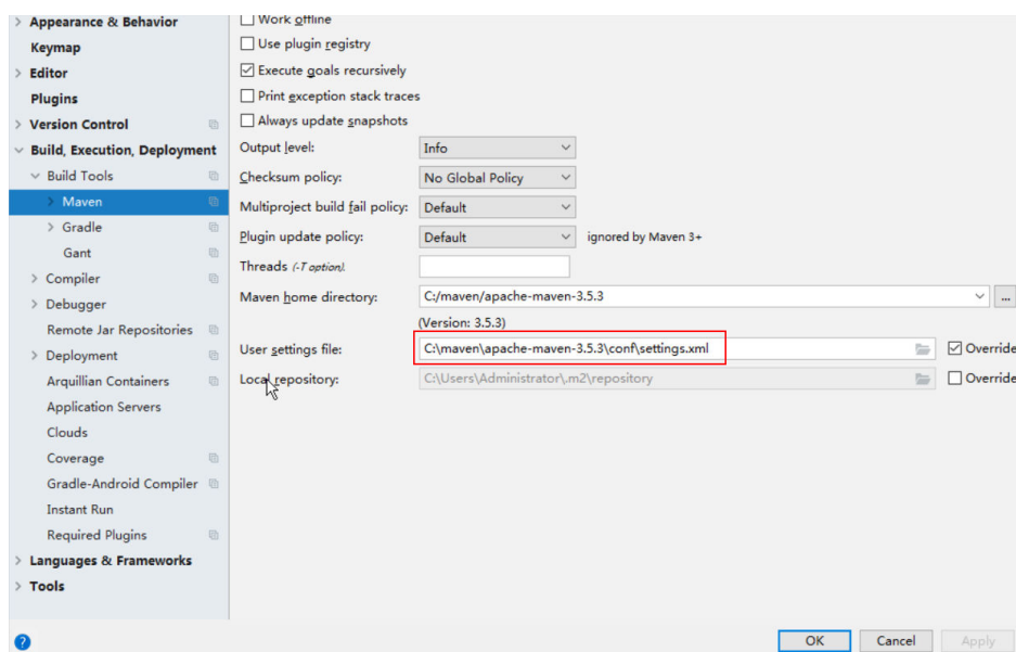
图 17-10 “settings.xml”文件放置目录
