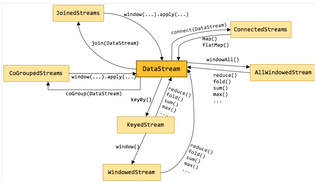
图 9-57 Flink Stream 的各种流类型转换
