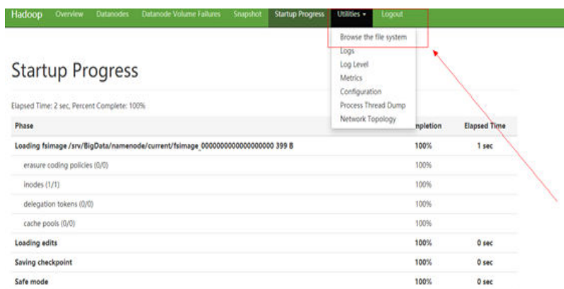
图 19-26 进入“Browse the file system”页面
