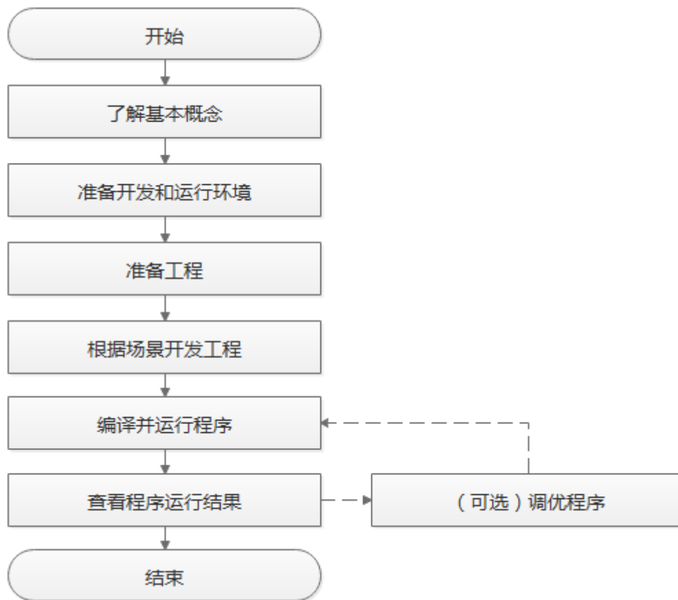
图 15-1 HetuEngine 应用程序开发流程
