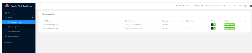
图 9-50 运行的作业
