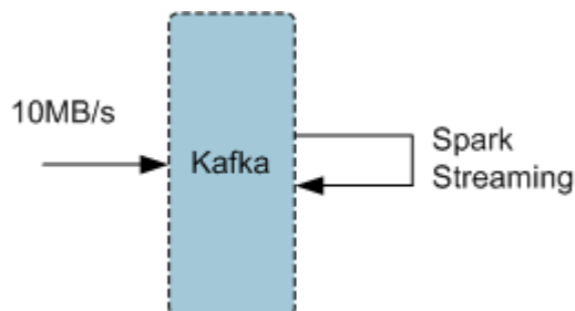
图 26-44 应用场景
