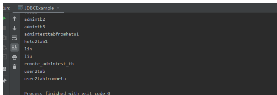
图 15-4 输出结果
