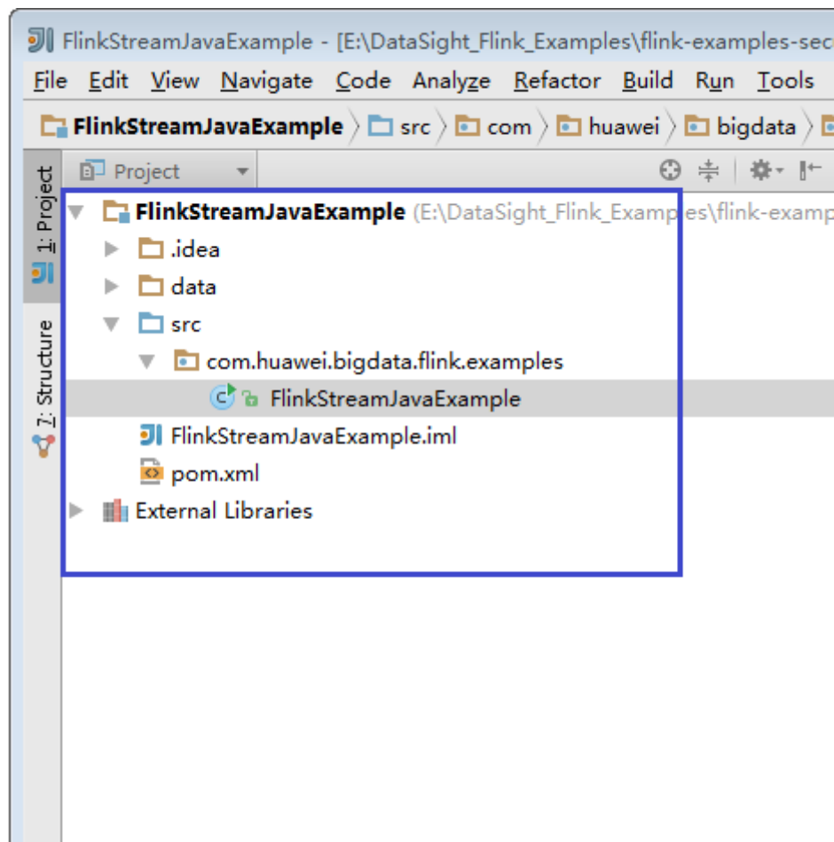
图 8-22 已导入工程
