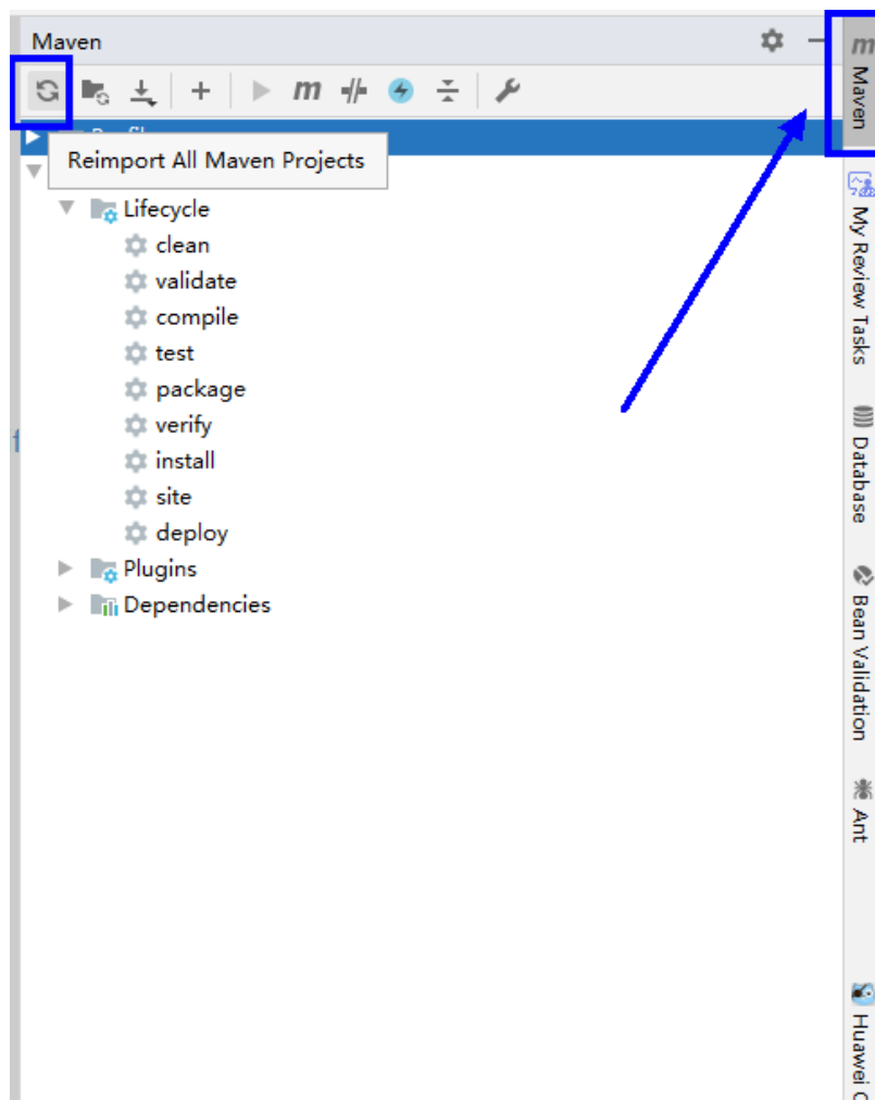
图 10-17 reimport projects
