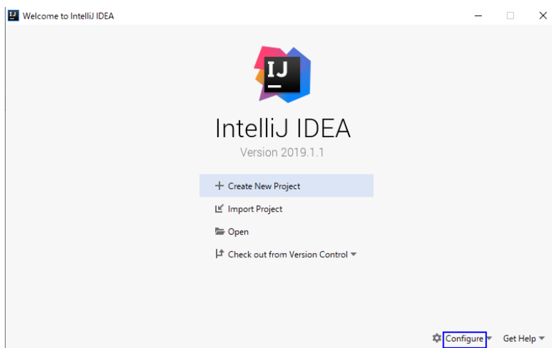
图 10-2 Quick Start
