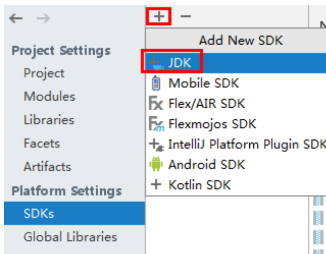
图 16-4 添加 JDK
