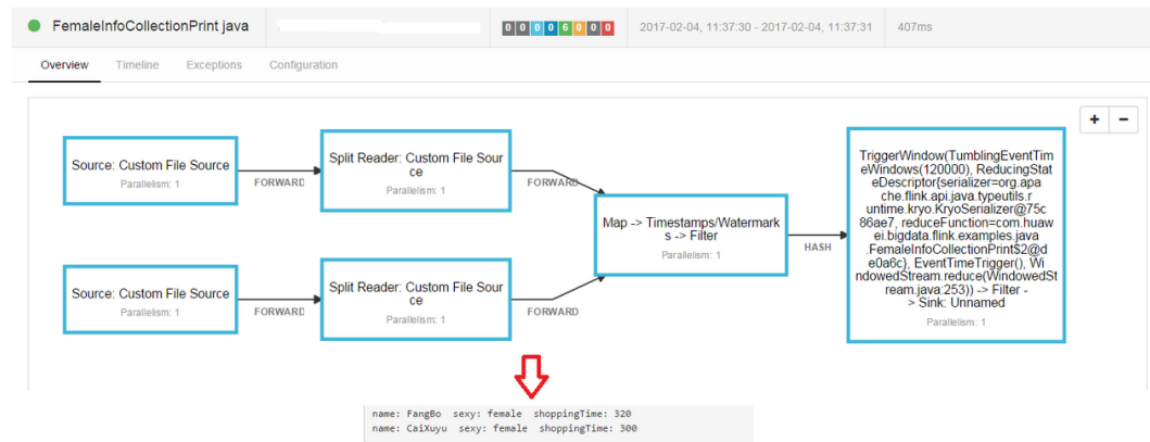
图 9-35 显示图
