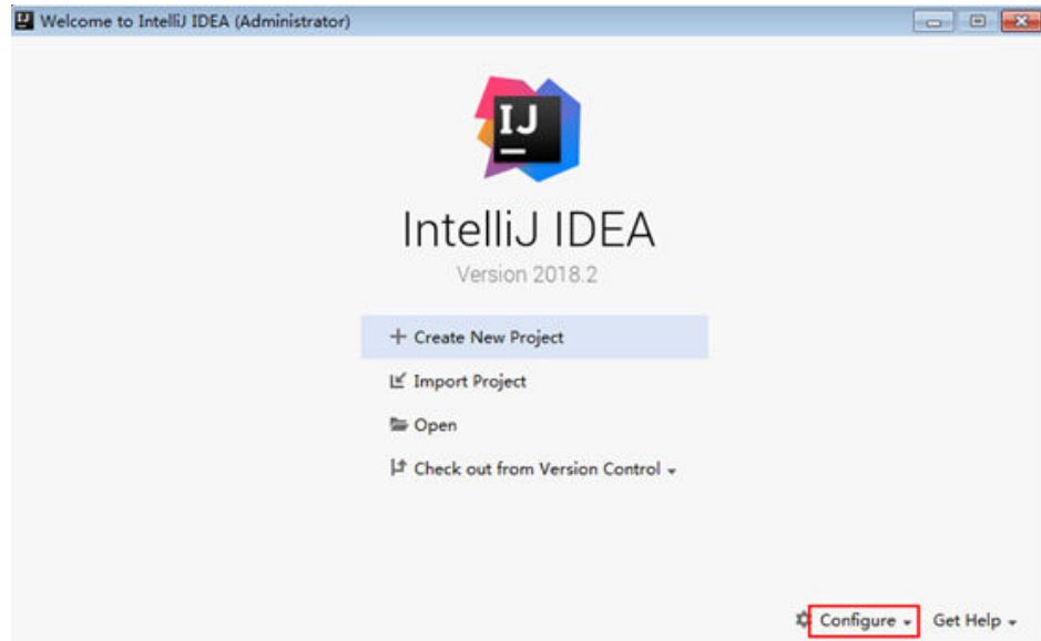
图 12-3 Quick Start
