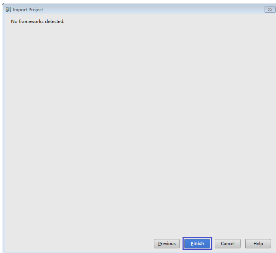
图 8-21 导入结束
