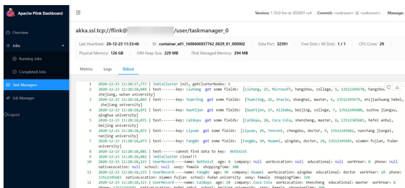
图 8-50 输出结果
