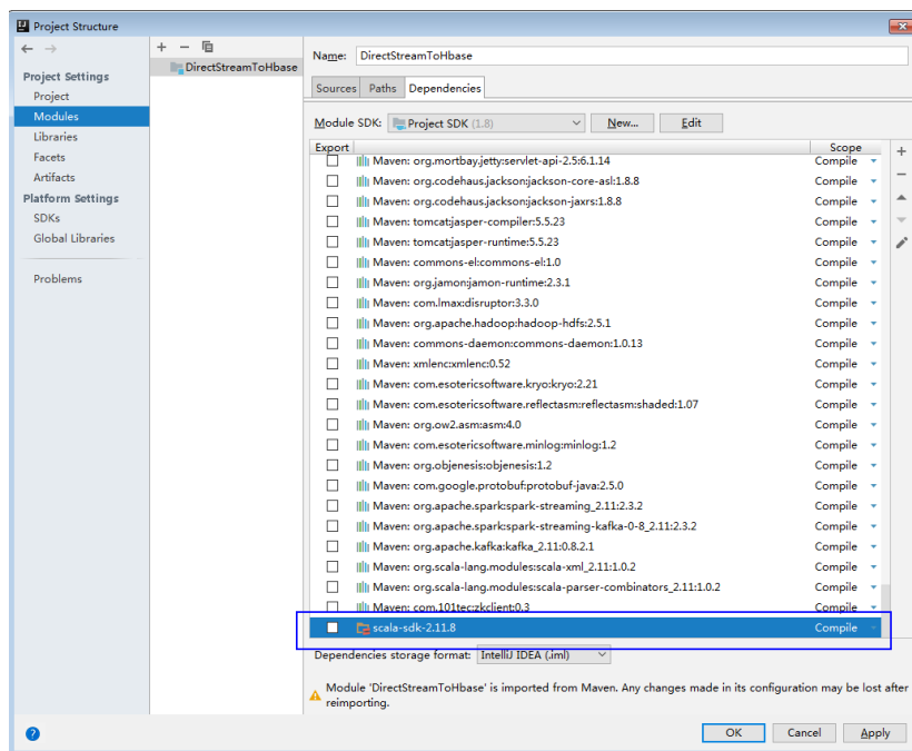
图 27-30 设置成功
