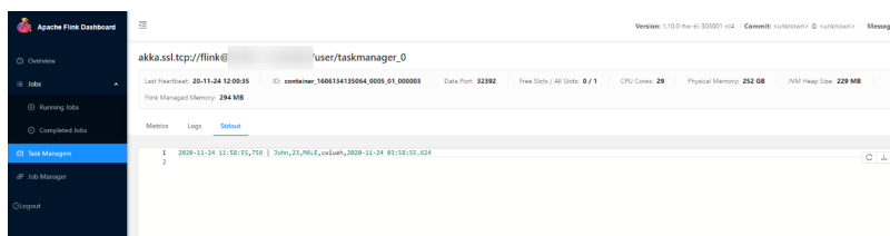
图 8-56 运行结果
