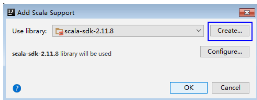
图 27-27 Create...
