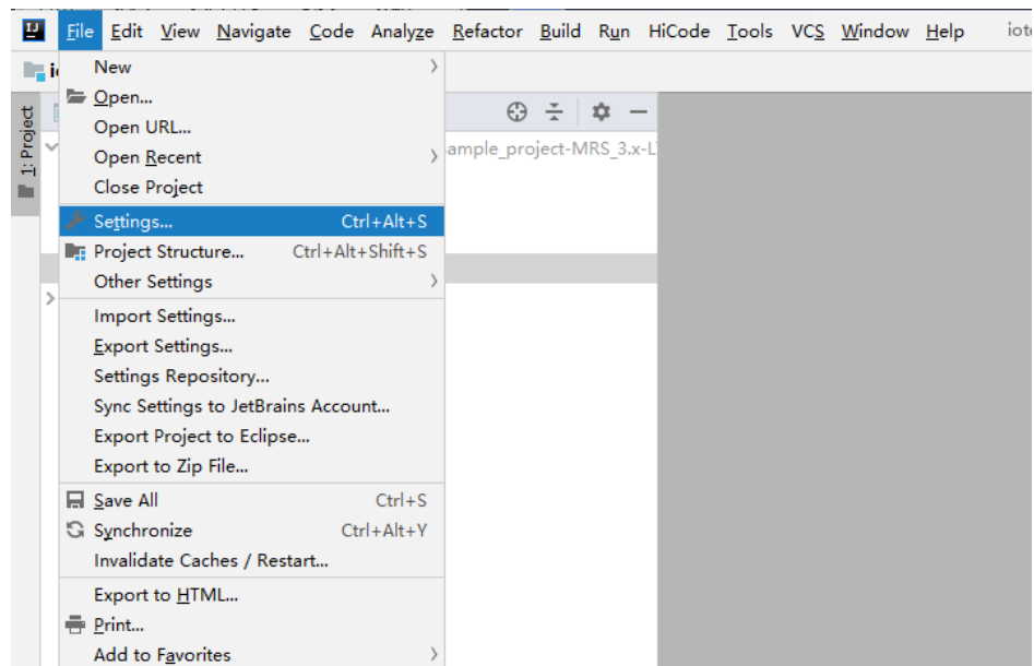
图 19-11 Settings
