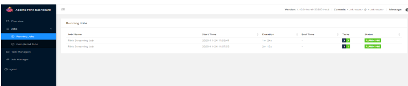
图 9-50 运行的作业
