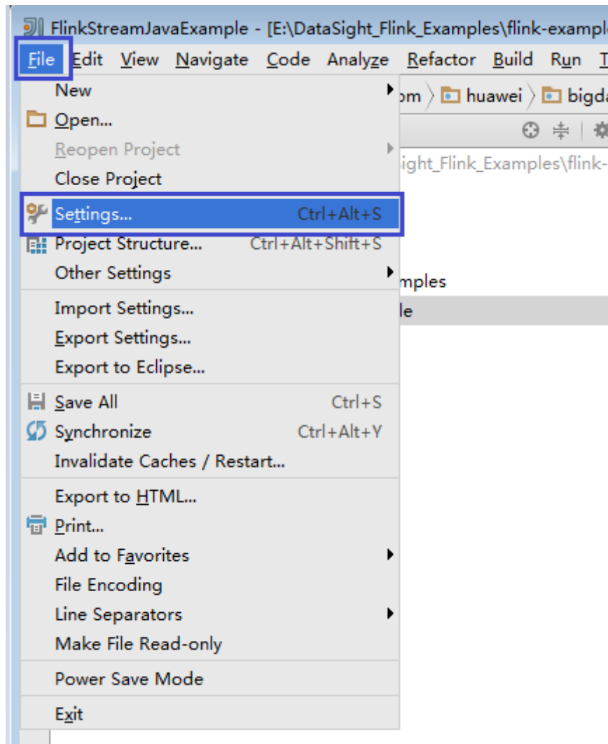
图 9-29 选择 Settings
