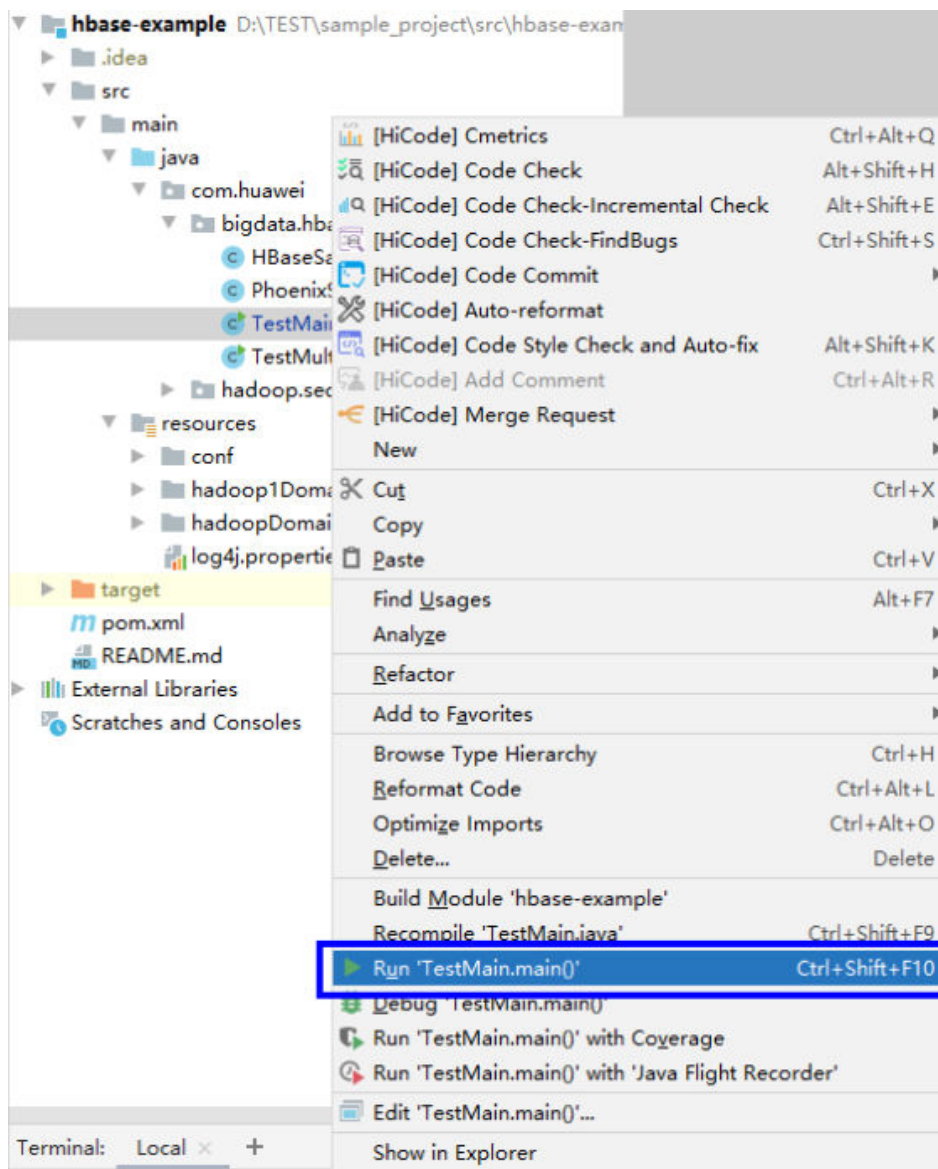
图 10-22 运行程序
