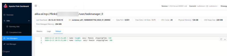
图 8-53 运行结果
