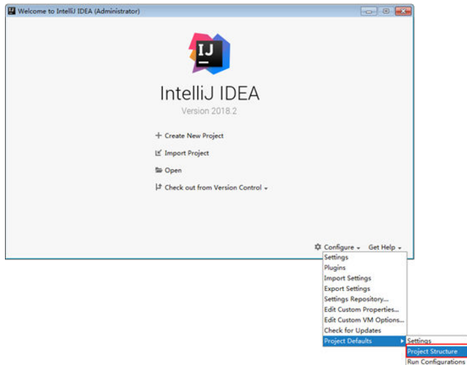
图 12-4 Configure
