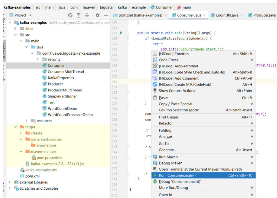
图 21-15 运行 Consumer.java
