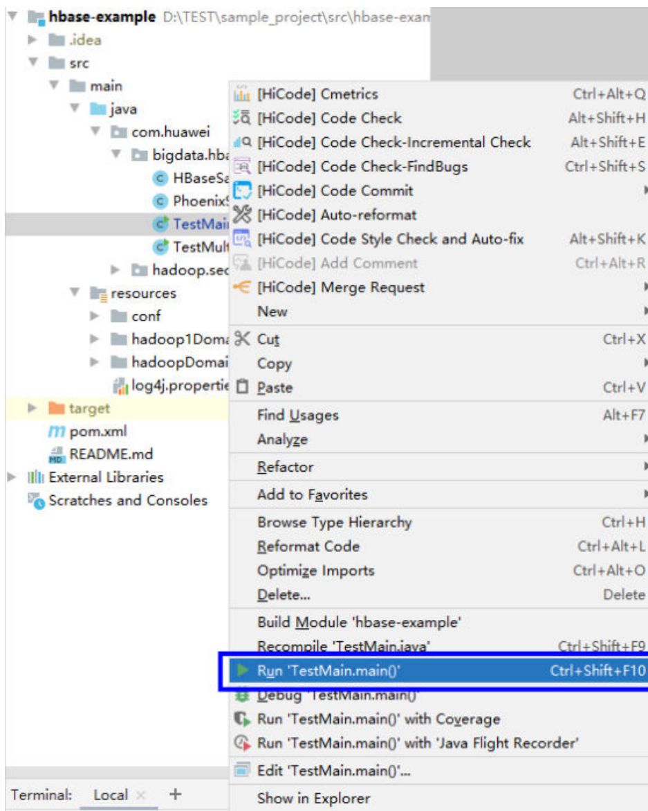
图 11-22 运行程序
