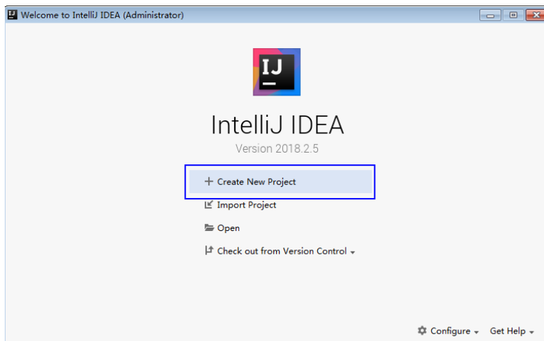
图 26-32 创建工程
