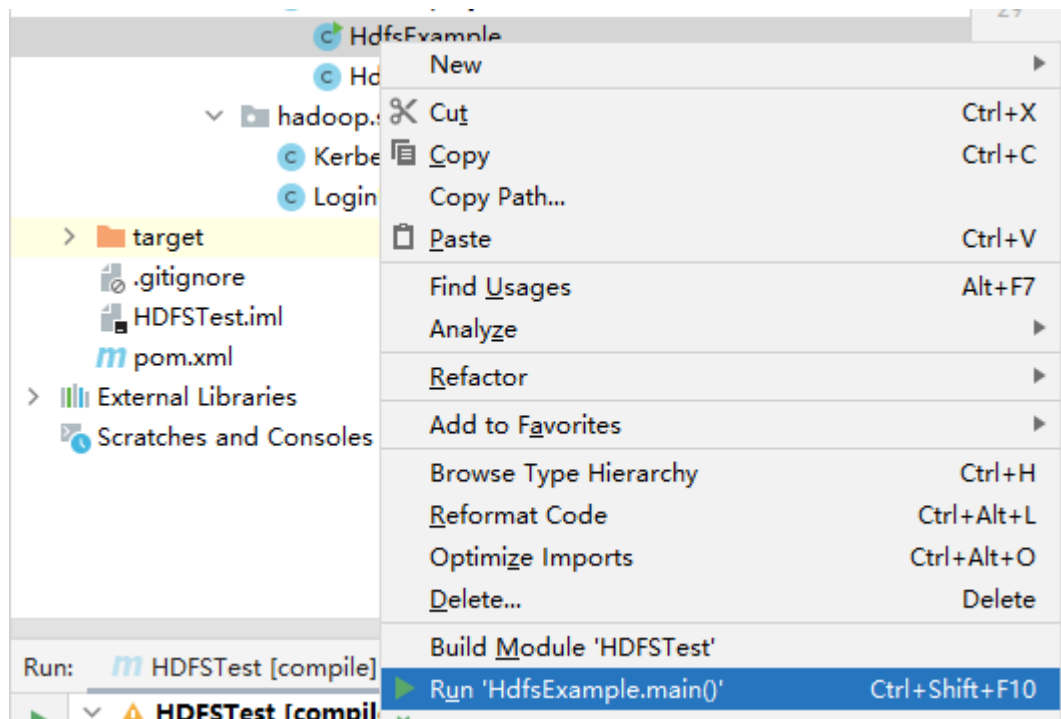
图 5-8 运行程序
