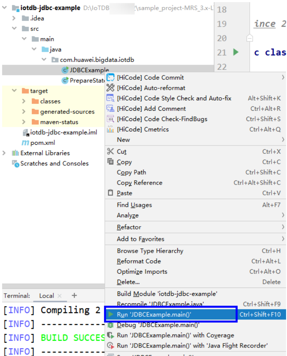
图 18-17 运行程序
