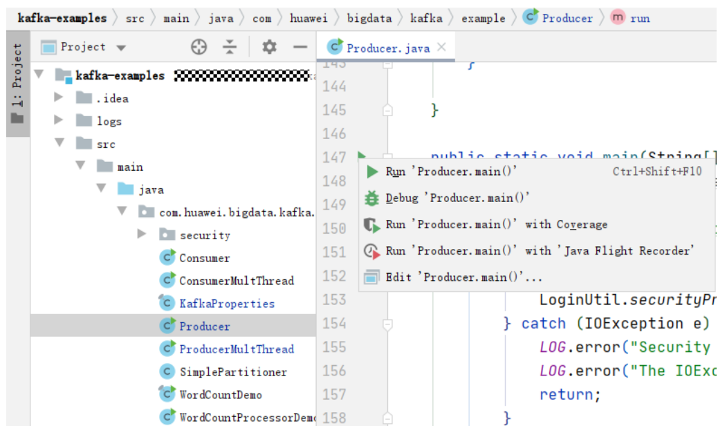
图 20-11 运行 Producer.java
