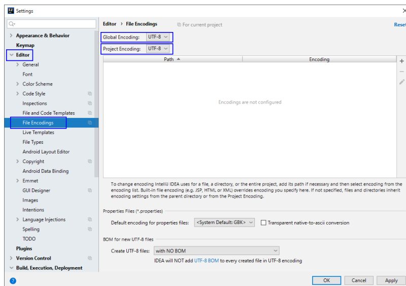
图 11-16 File Encodings
