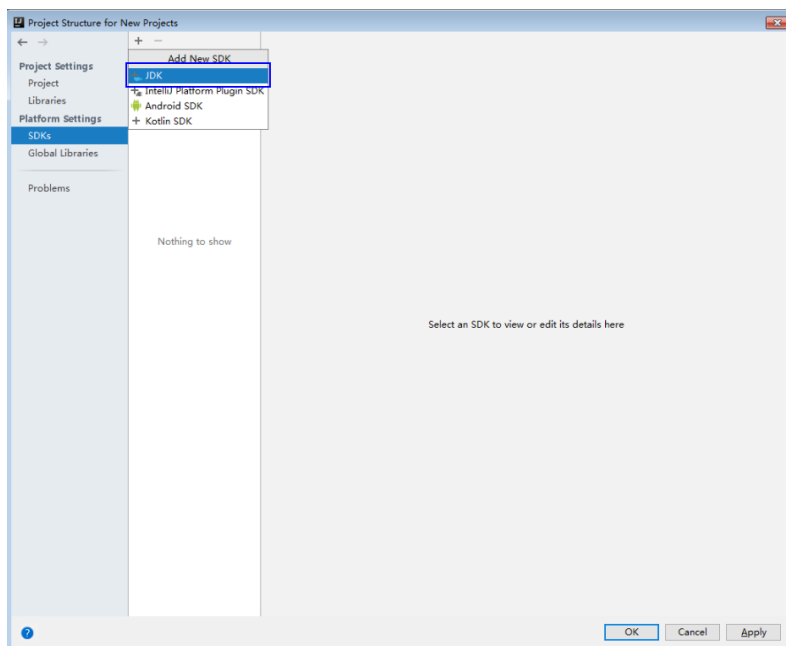
图 27-13 添加 JDK
