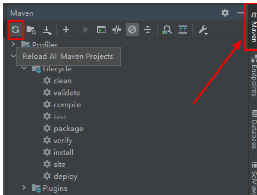
图 9-37 Reload projects
