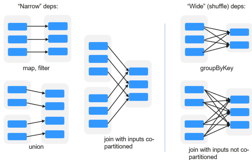
图 26-1 RDD 的依赖
