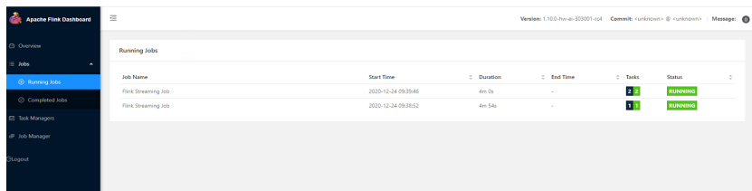
图 9-53 运行的作业
