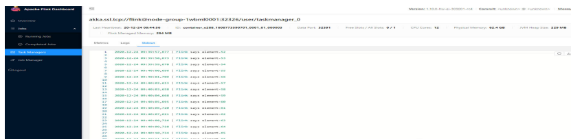
图 9-55 运行结果
