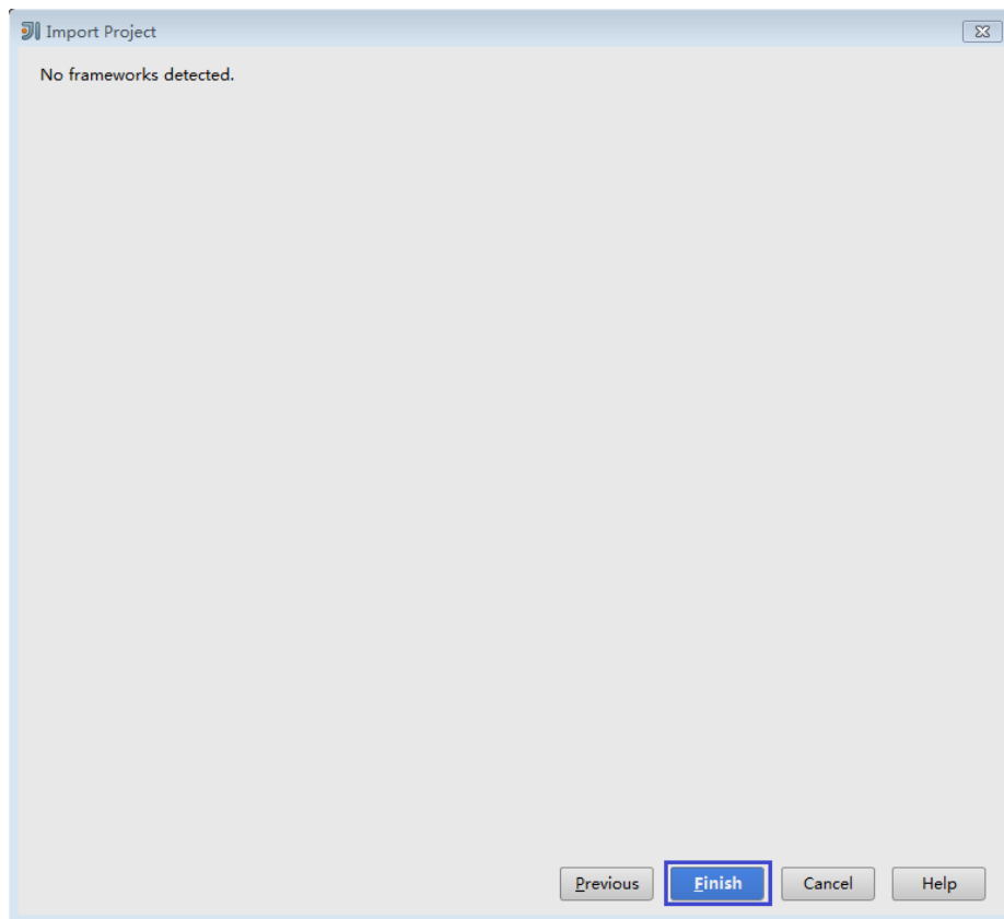
图 9-21 导入结束
