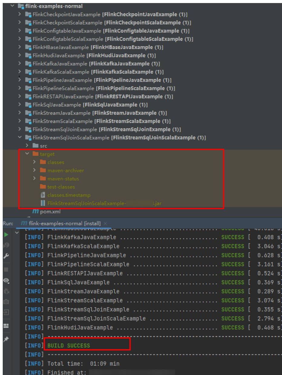
图 9-40 编译完成
