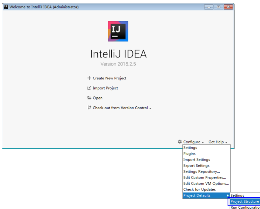
图 26-12 Project Defaults
