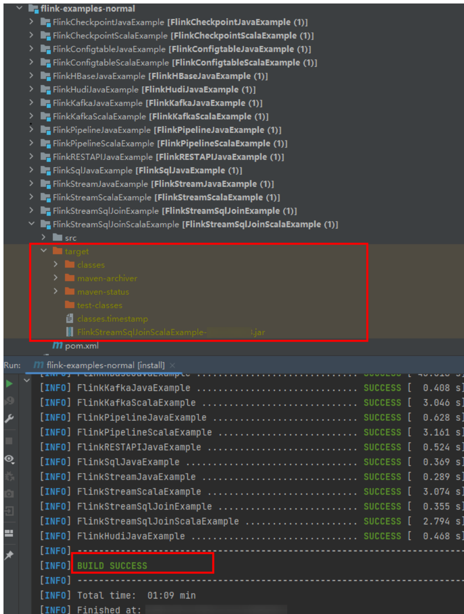
图 9-40 编译完成
