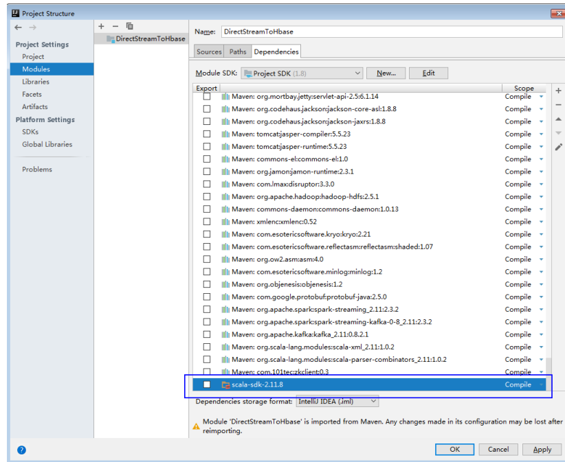
图 27-30 设置成功
