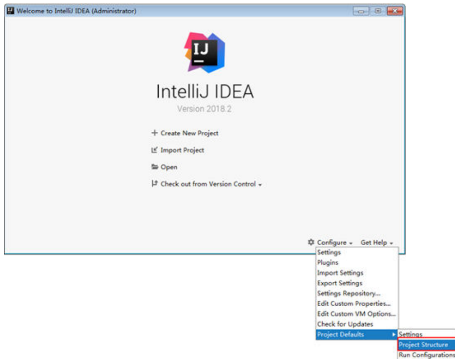
图 12-4 Configure
