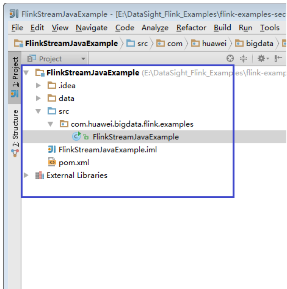
图 9-22 已导入工程
