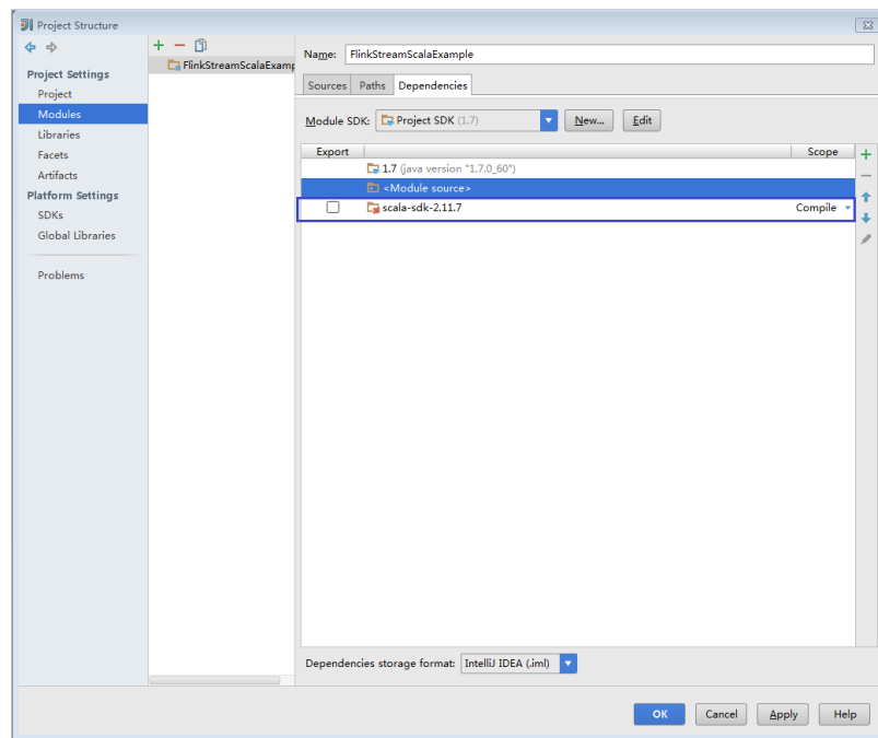
图 9-28 设置成功
