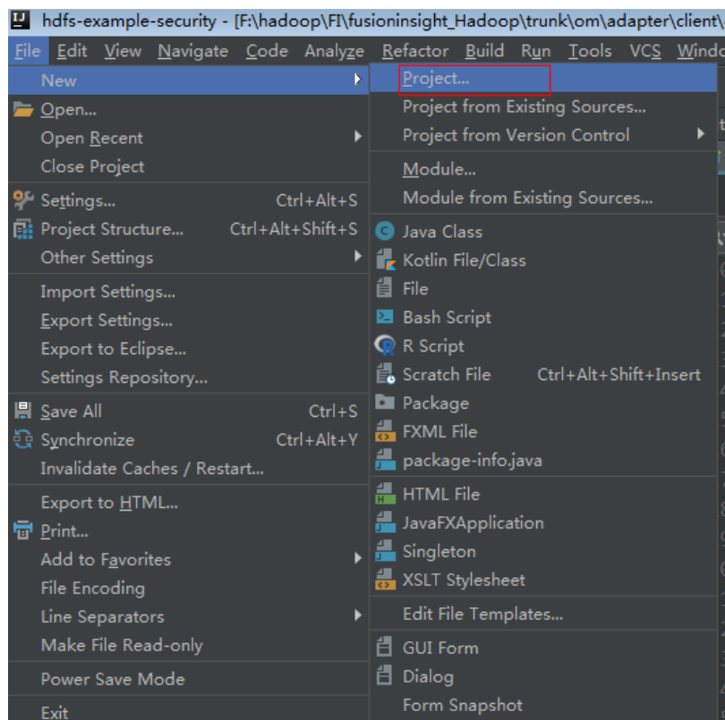
图 23-5 创建工程
