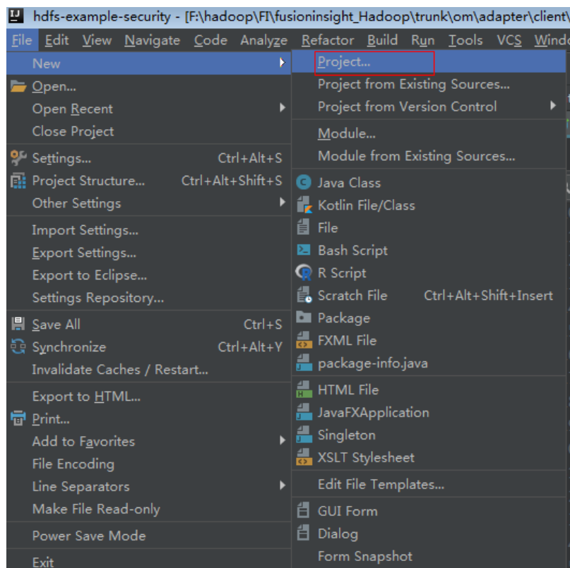
图 23-5 创建工程
