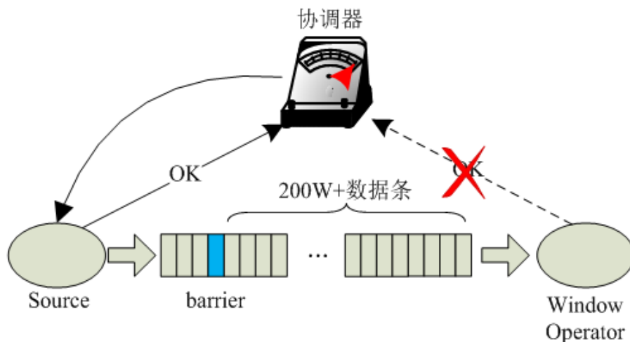
图 8-66 关系图
