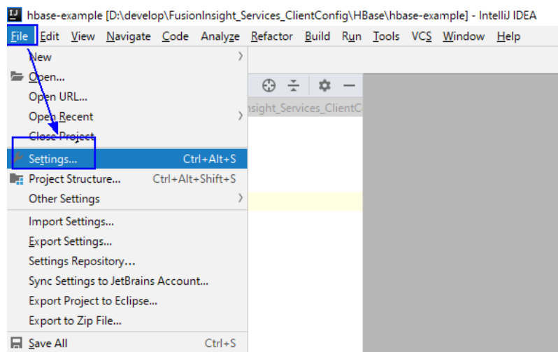
图 11-15 Settings
