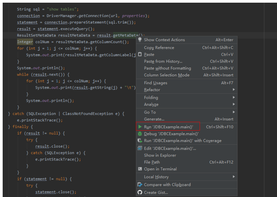
图 15-3 运行程序
