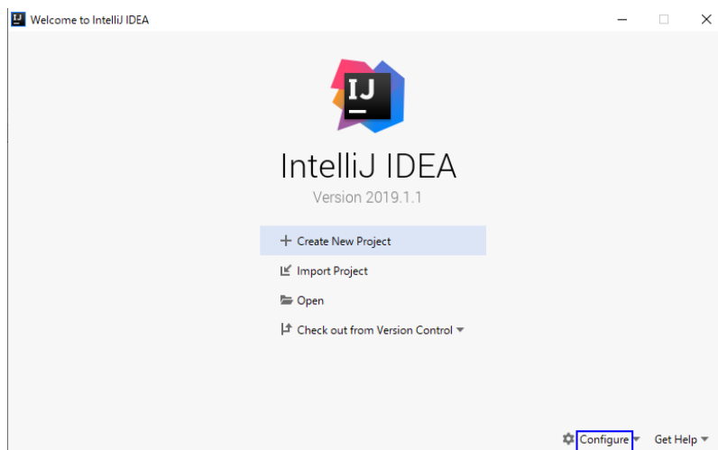
图 11-2 Quick Start
