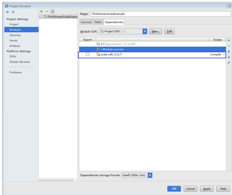
图 9-28 设置成功
