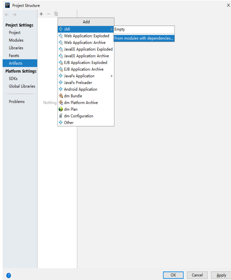
图 18-21 添加 Artifacts
