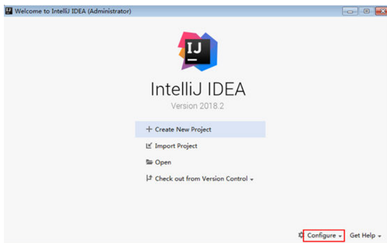
图 20-2 Quick Start
