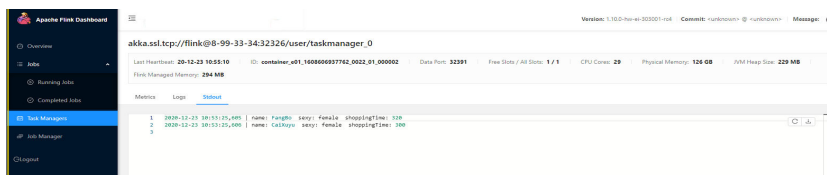
图 9-49 运行结果
