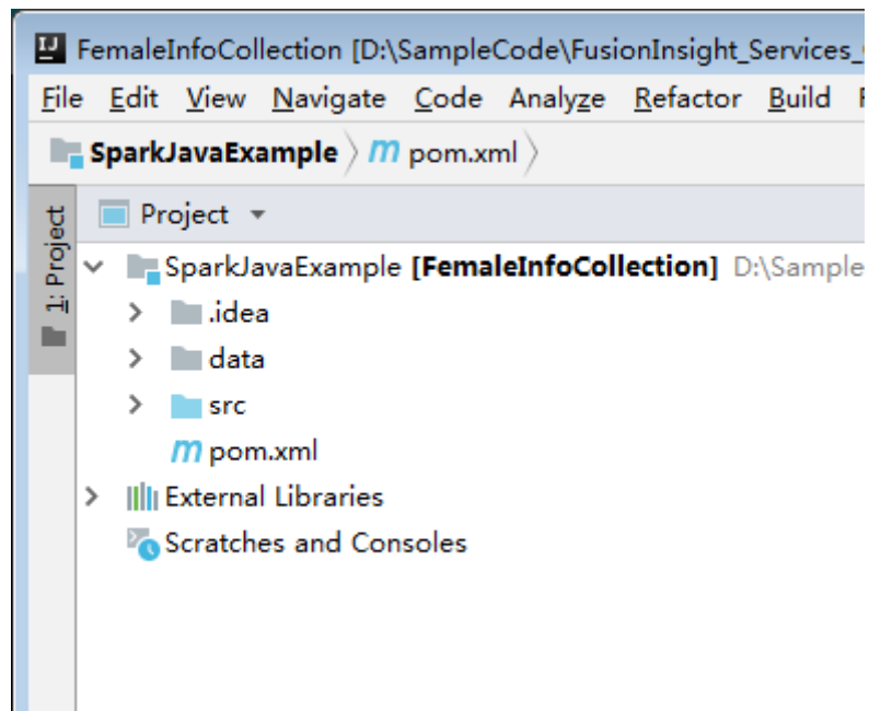
图 27-24 已导入工程
