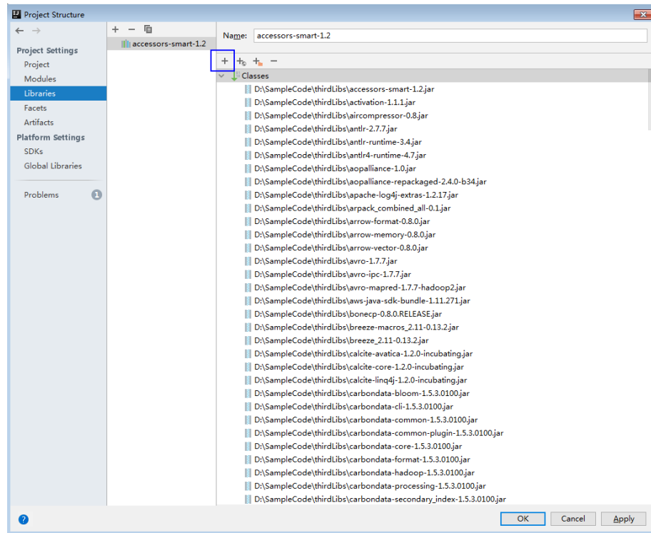
图 27-41 添加依赖包
