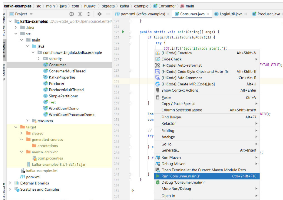
图 20-16 运行 Consumer.java
