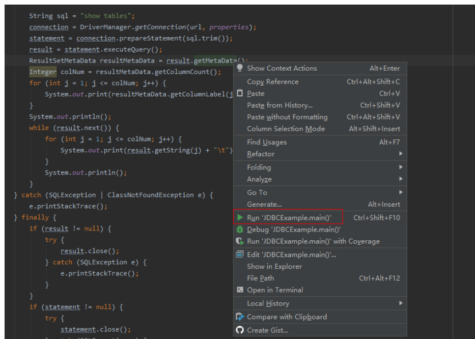
图 15-3 运行程序
