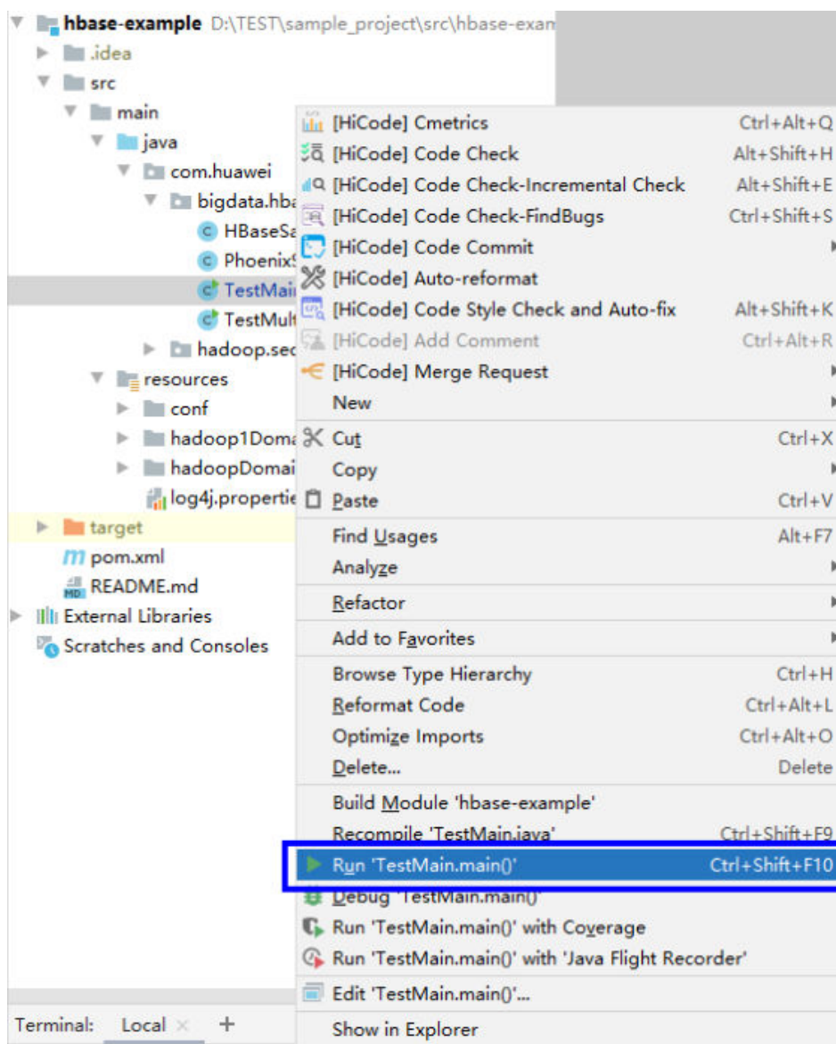
图 11-22 运行程序
