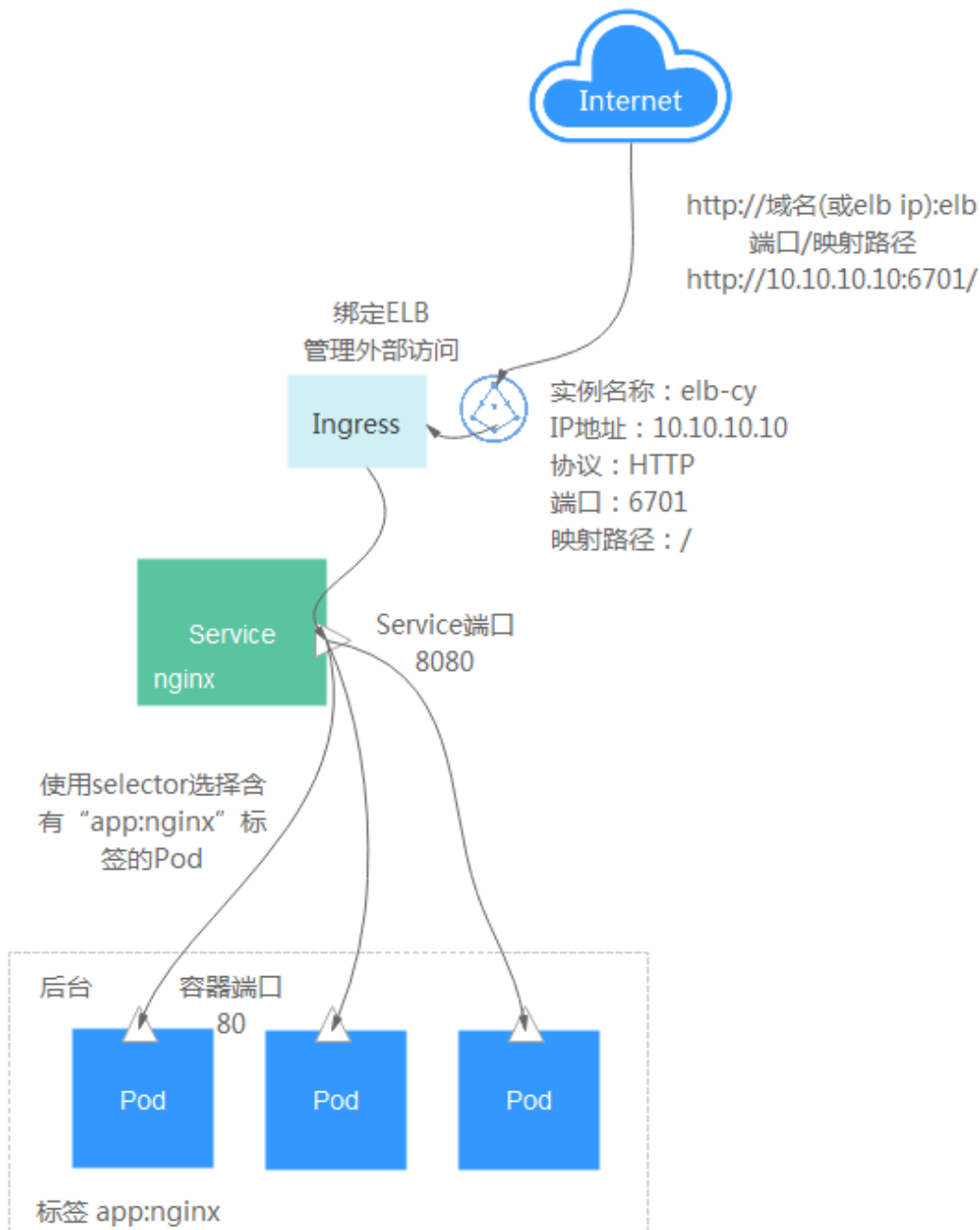
图 11-5 Ingress
