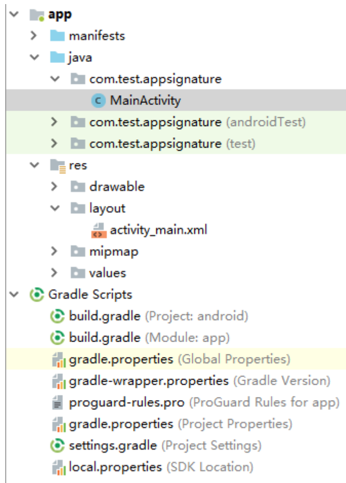
图 2-21 工程目录结构
