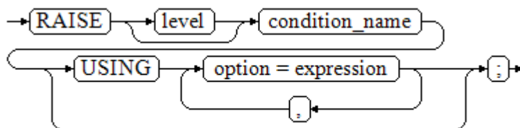
图 10-35 raise_condition::=
