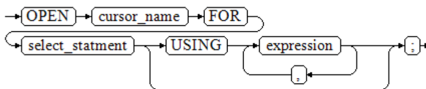
图 10-30 open_dynamic_cursor::=
