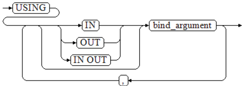
图 10-14 using_clause-4
