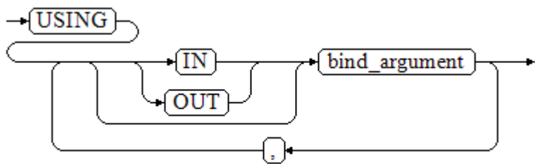
图 10-7 using_clause-1
