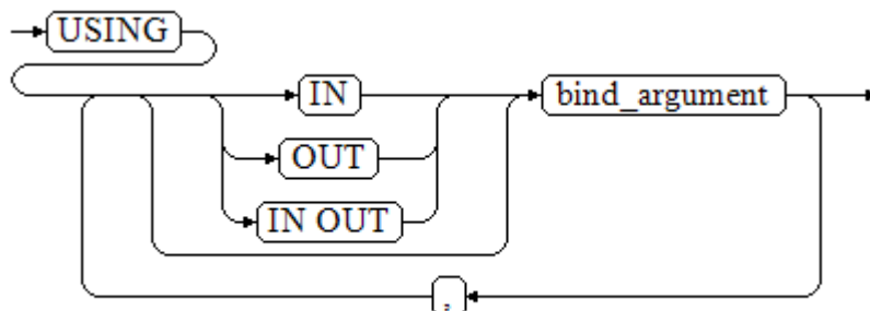
图 9-14 using_clause-4
