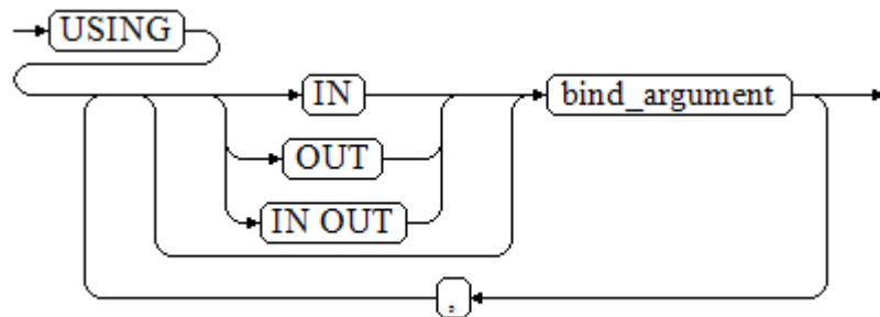
图 9-12 using_clause-3
