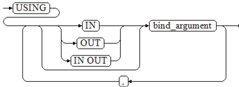
图 9-12 using_clause-3
