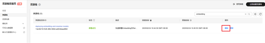
图 3-24 一键卸载
