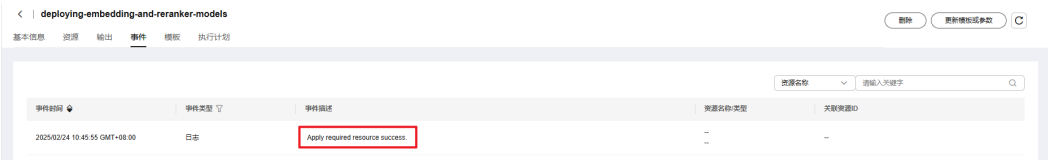
图 3-16 部署完成
