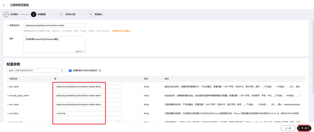
图 3-10 配置参数
