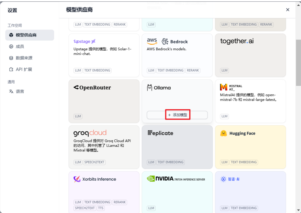
图 3-20 添加模型
