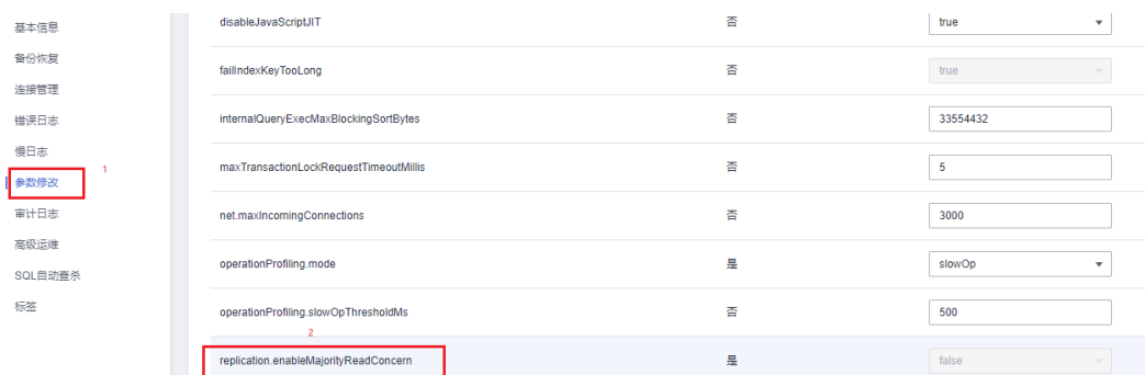
图 17-2 查看参数 enableMajorityReadConcern 的设置值
