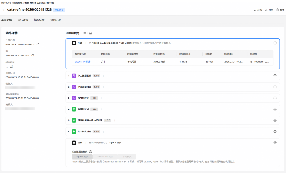
图 4-7 基本信息
