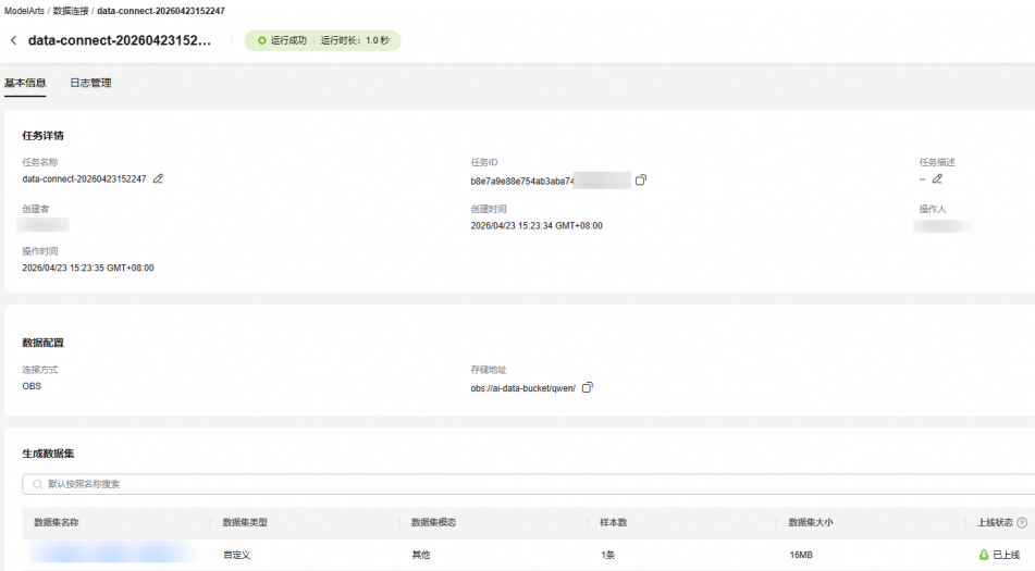
图 3-4 基本信息
