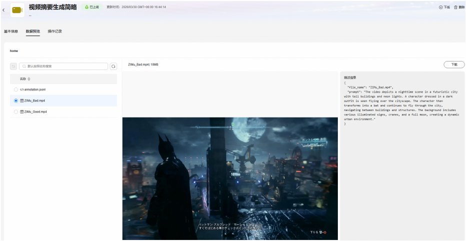
图 4-13 打标样例
