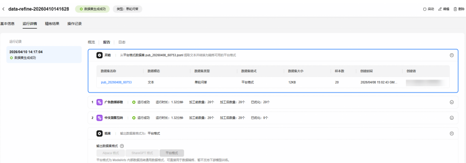
图 4-9 报告
