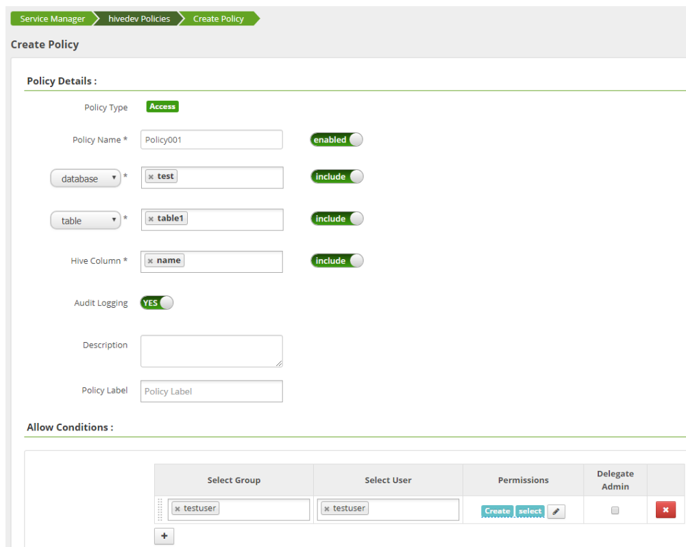
图 23-8 新增 hivedev 的访问控制策略
