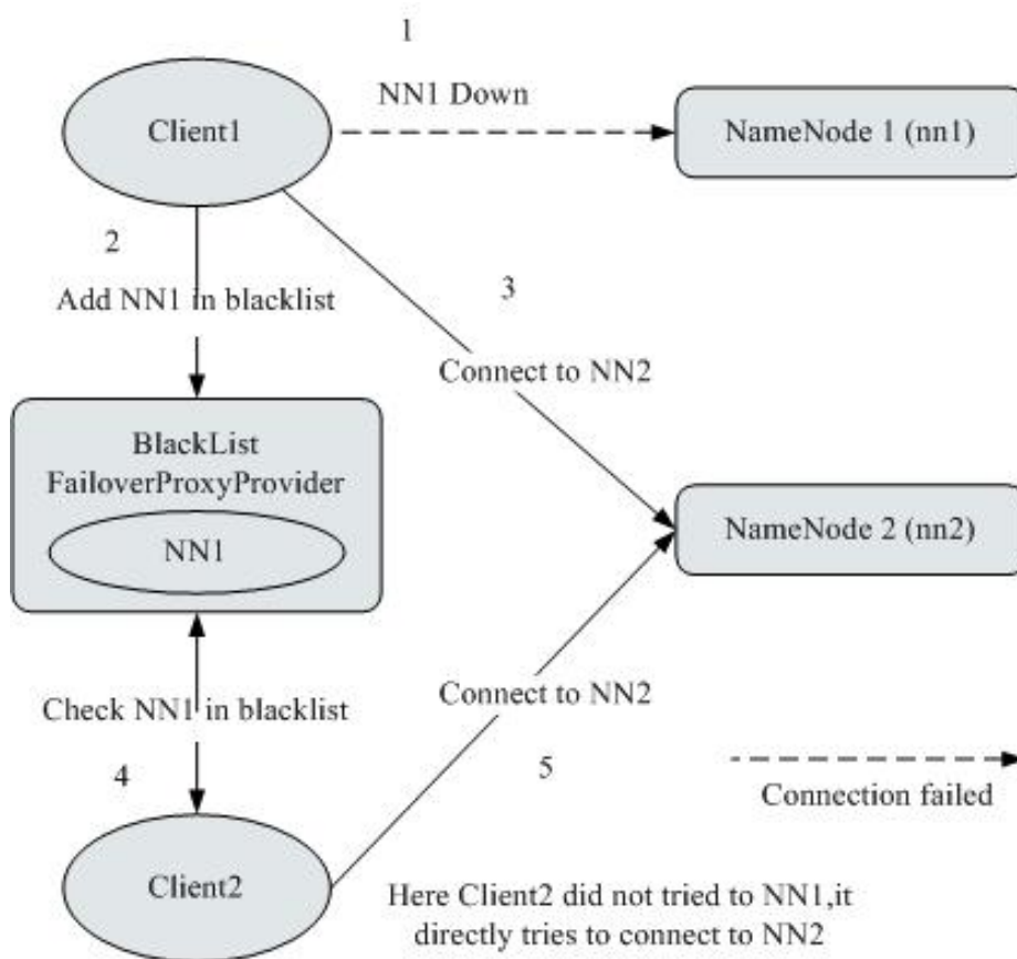
图 9-11 NameNode blacklisting 状态图
