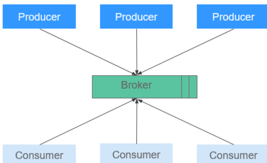
图 15-1 Kafka 结构
