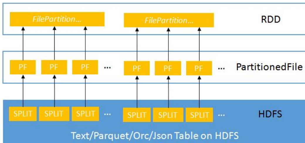
图 26-7 小文件合并
