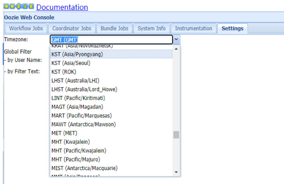
图 13-12 时区参考
