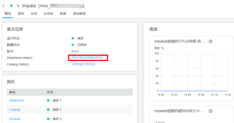
图 14-1 StateStore WebUI
