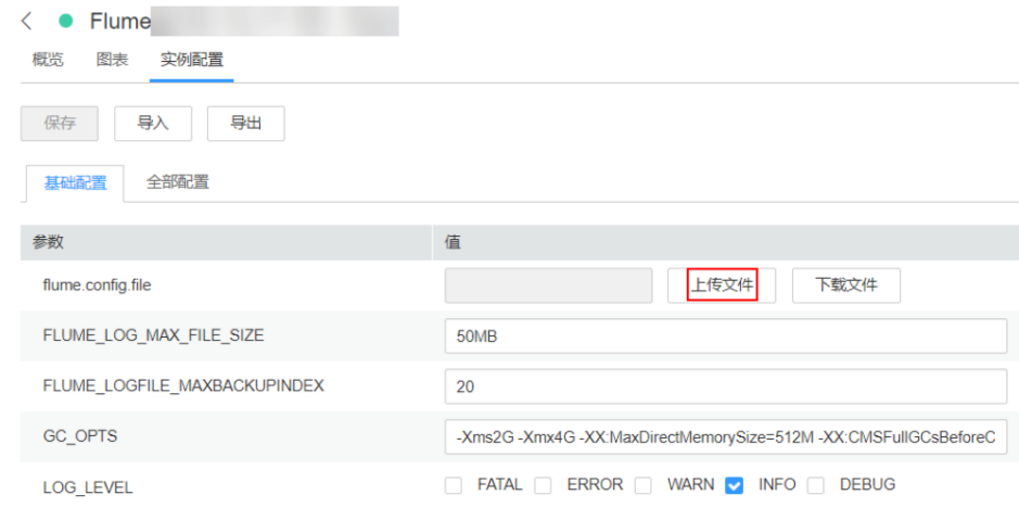
图 7-8 上传文件
