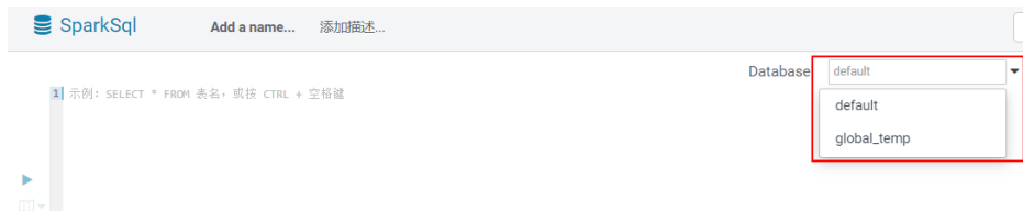
图 13-3 选择数据库
