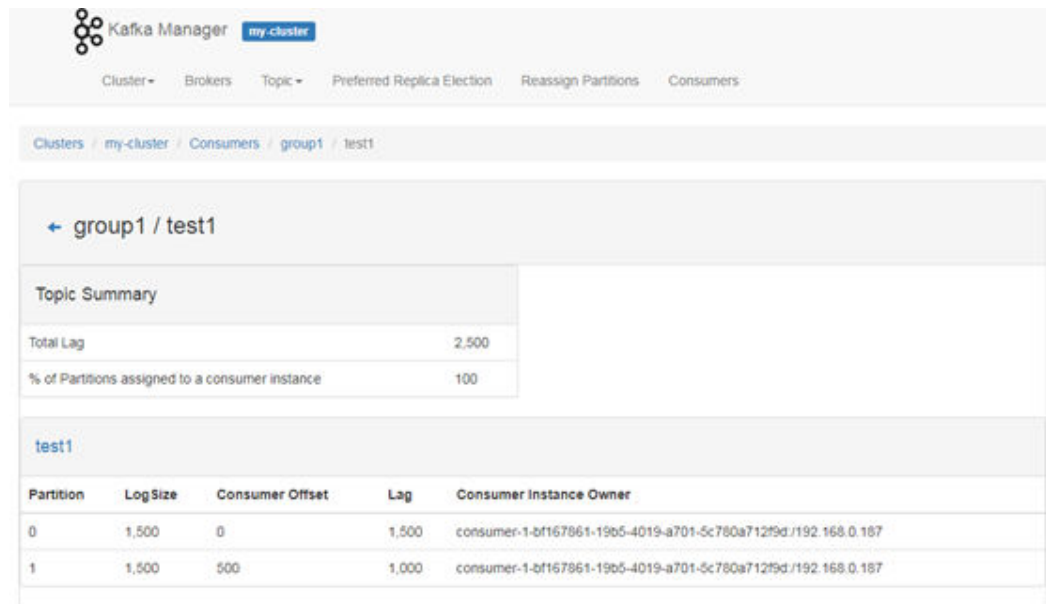
图 16-11 Consumer 对 Topic 的具体消费情况
