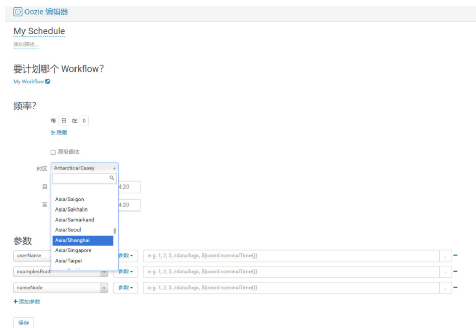
图 13-11 时区选择
