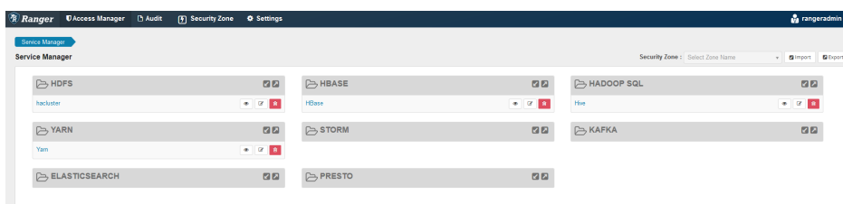
图 24-1 Ranger WebUI
