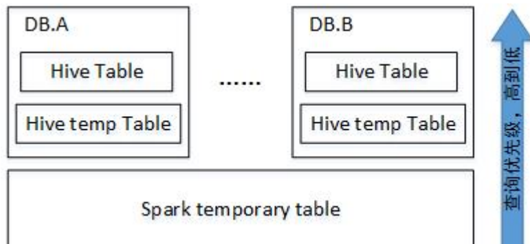
图 25-13 Spark 表管理层次
