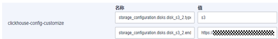
图 3-11 clickhouse-config-customize 参数配置 OBS 盘示例
