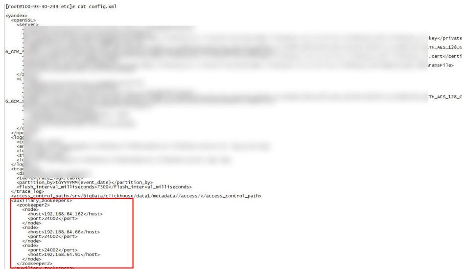
图 3-19 查看已添加的源集群的 ZooKeeper 信息
