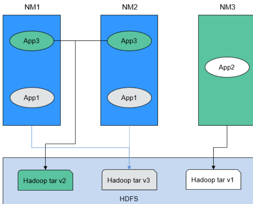
图 21-1 具有多个版本 NodeManagers 及 Applications 的集群
