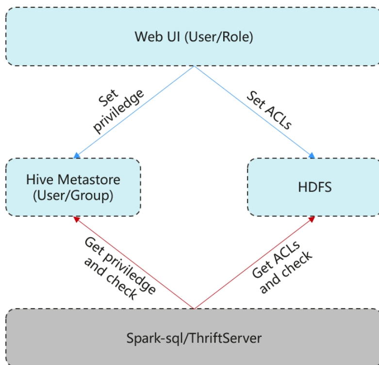
图 25-1 SparkSQL 权限管理架构图
