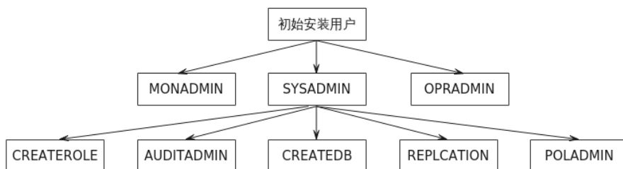
图 8-1 权限架构
