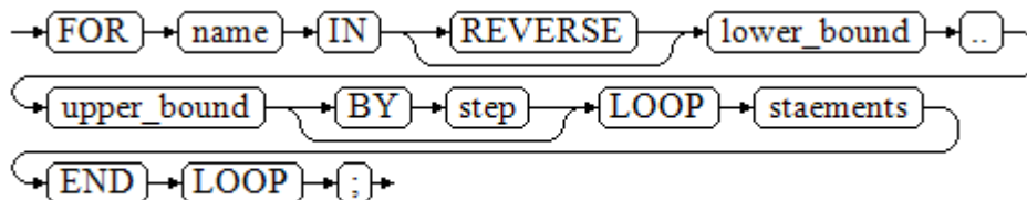
图 10-22 for_loop::=
