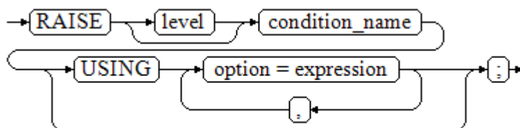
图 10-37 raise_condition::=
