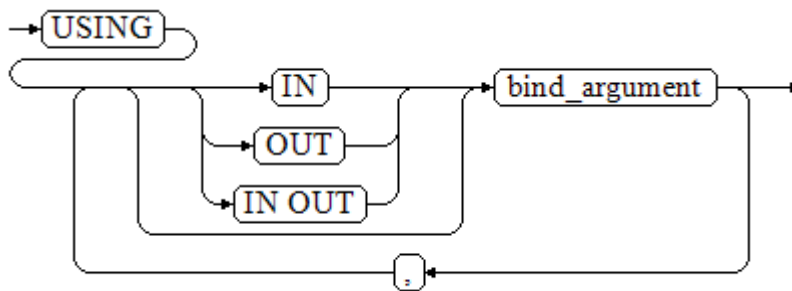
图 10-13 using_clause::=
