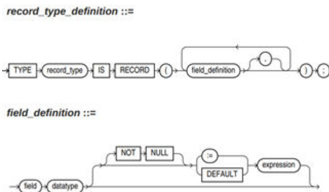
图 10-1 record 类型的语法
