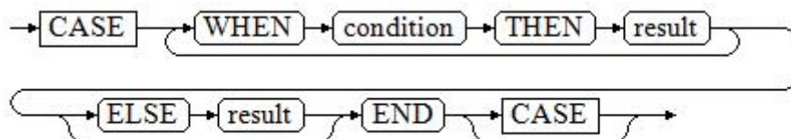
图 11-1 case::=
