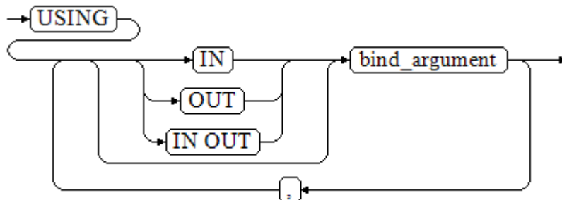
图 12-13 using_clause::=
