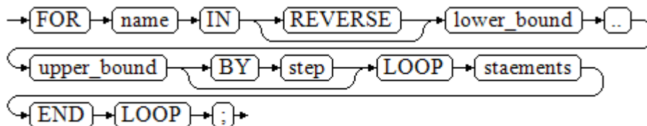
图 12-22 for_loop::=
