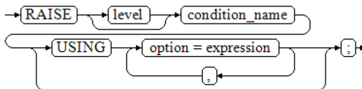
图 12-36 raise_condition::=
