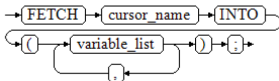
图 12-32 fetch_cursor::=
