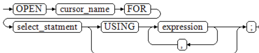
图 12-31 open_dynamic_cursor::=
