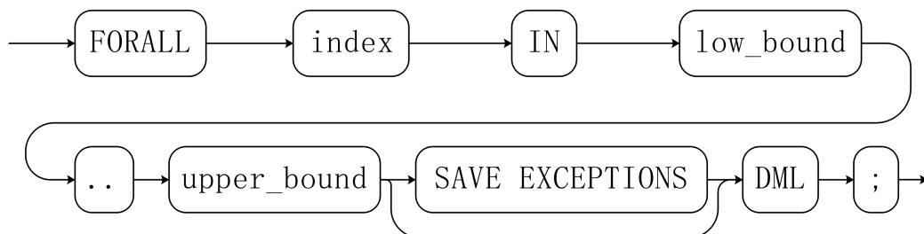
图 12-24 forall::=
