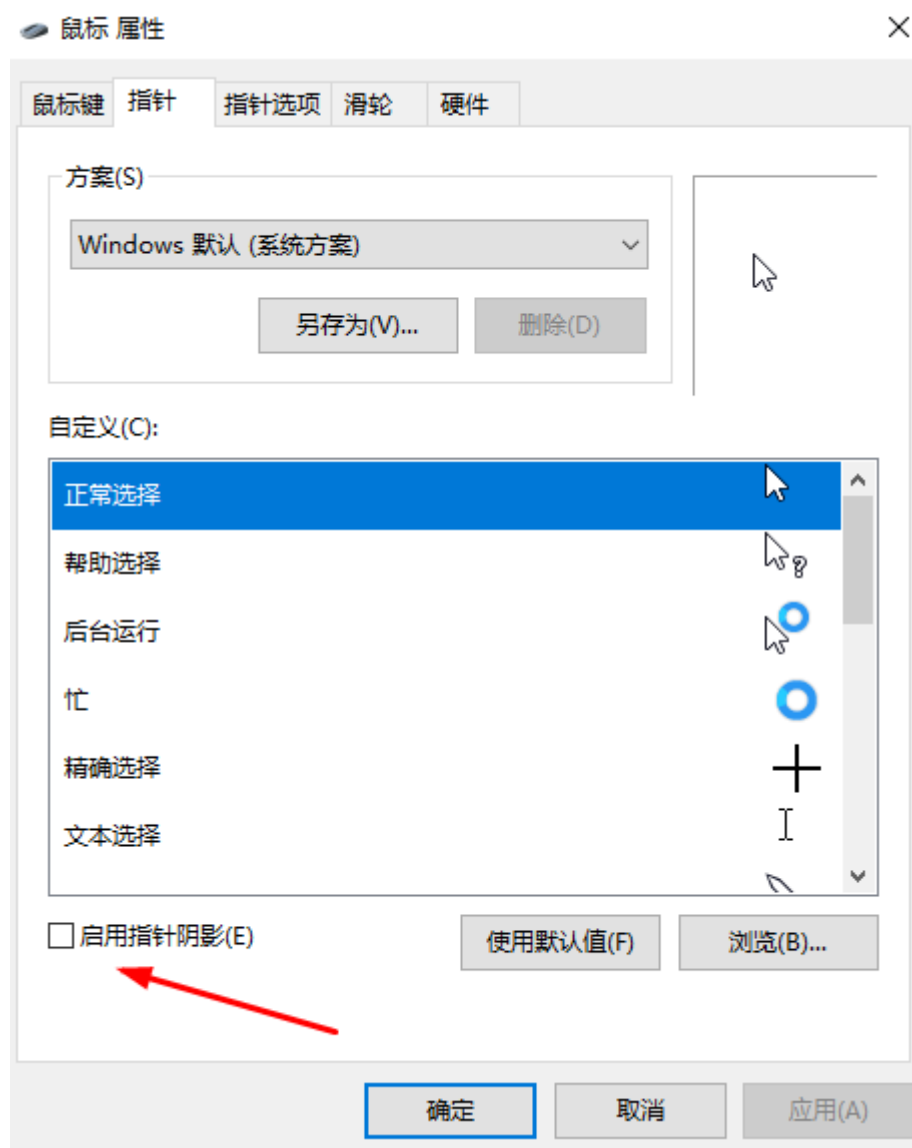
图 12-8 指针
