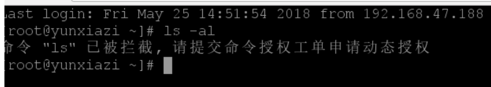
图 9-12 动态拦截
