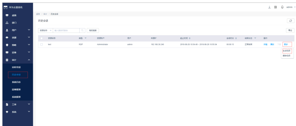
图 11-1 生成视频
