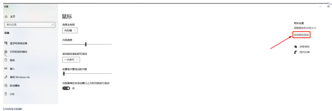
图 12-7 鼠标页面
