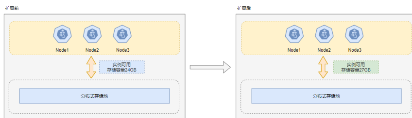
图 4-61 自动扩容实例存储示意图
