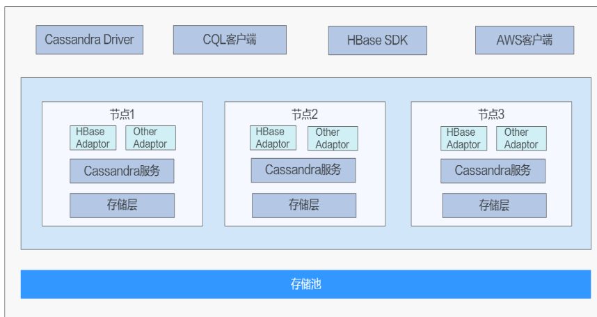
图 9-1 GeminiDB HBase 架构图
