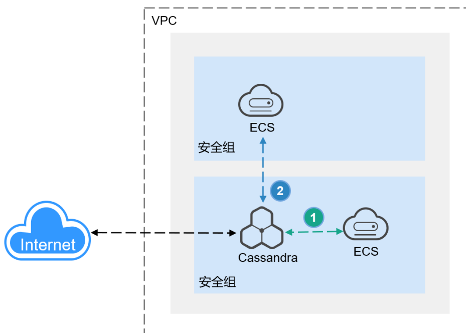
图 4-8 连接方式介绍
