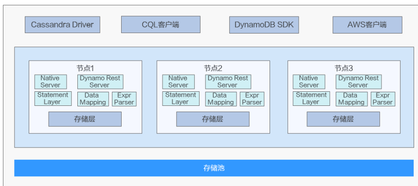
图 8-1 GeminiDB (兼容 DynamoDB API)架构图
