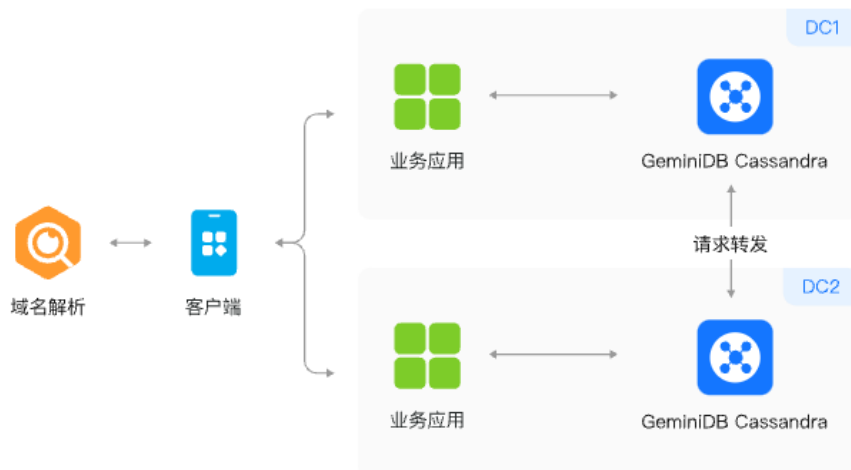
图 5-33 多 DC 部署场景
