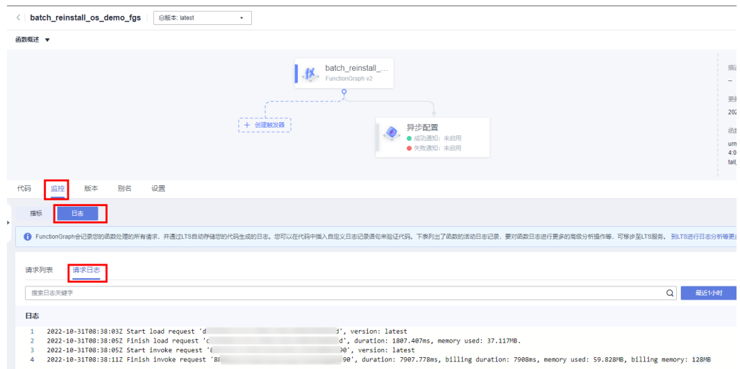
图 3-32 请求日志
