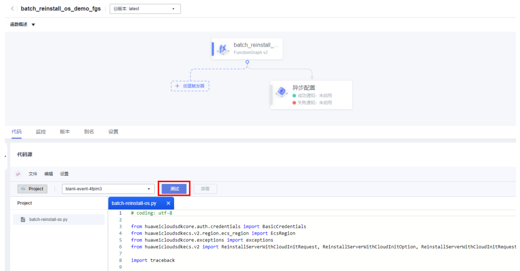
图 3-30 调用函数
