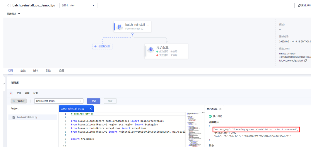
图 3-31 执行成功
