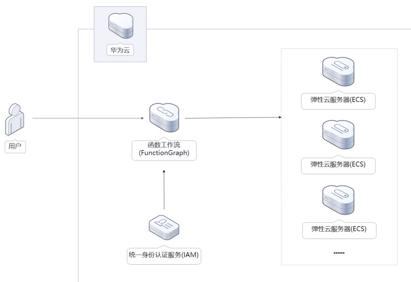
图 1-1 方案架构图
