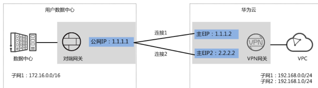
图 1-1 方案架构
