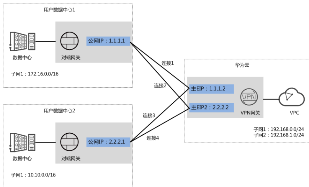
图 1-4 组网方案
