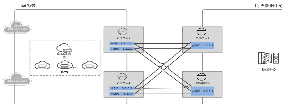
图 1-9 组网方案
