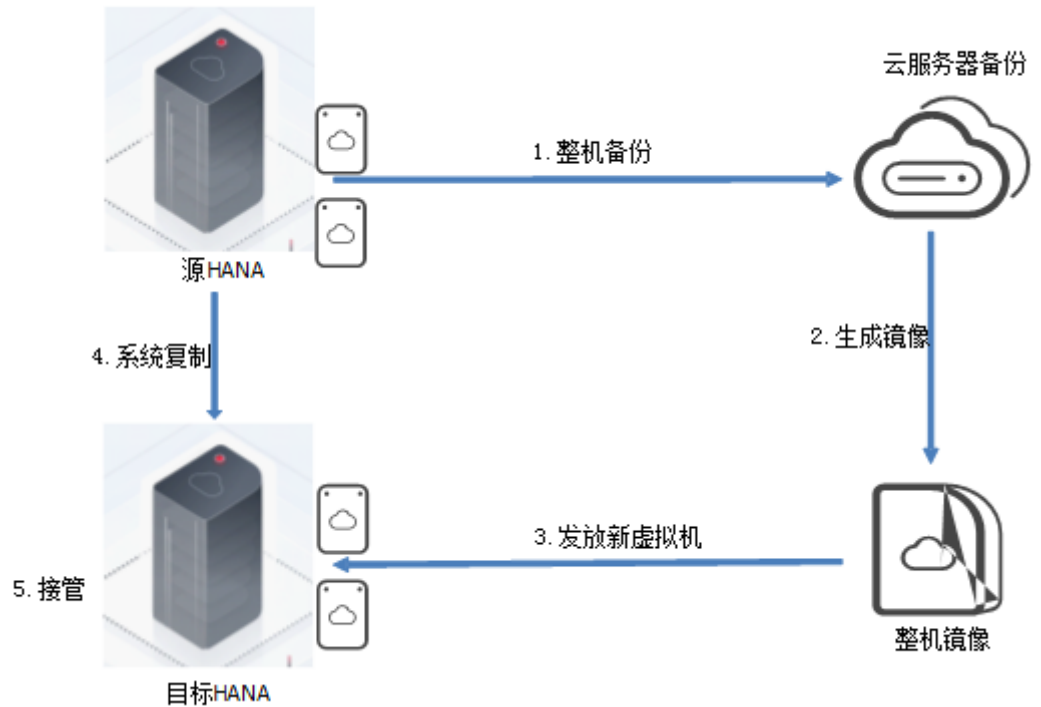
图 15-2 整机备份+系统复制方案
