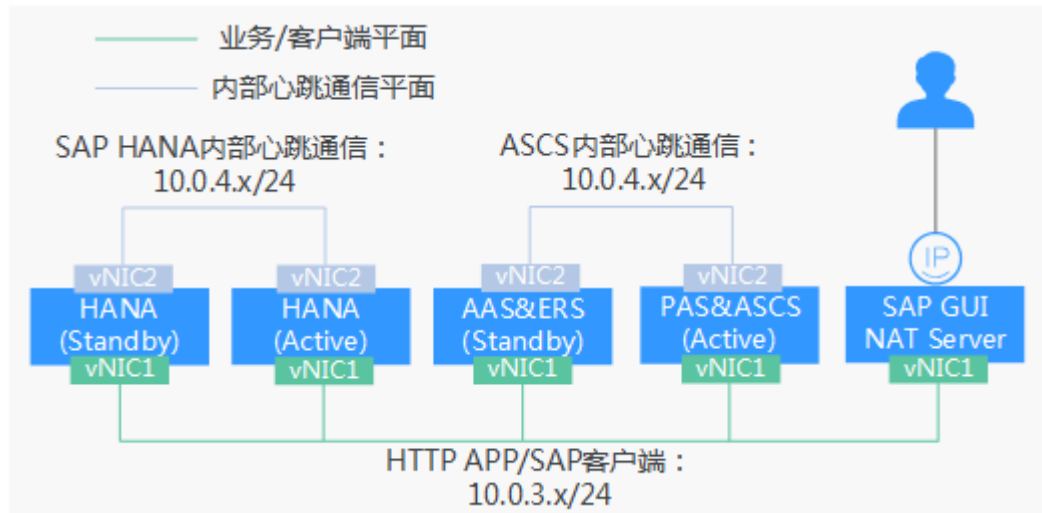
图 4-1 高可用部署网络平面规划
