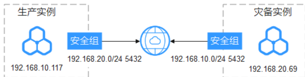
图 3-18 防火墙配置
