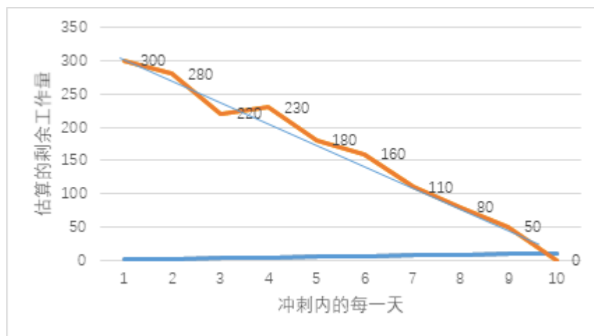
图 2-37 燃尽图
