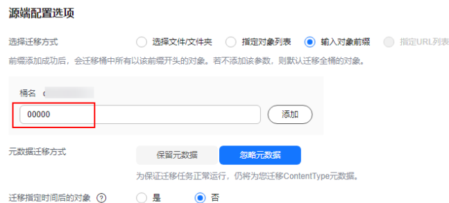
图 5-61 输入对象数据名称或名称前缀
