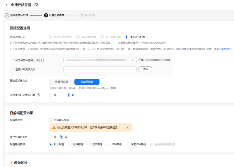
图 5-159 设置任务参数页面
