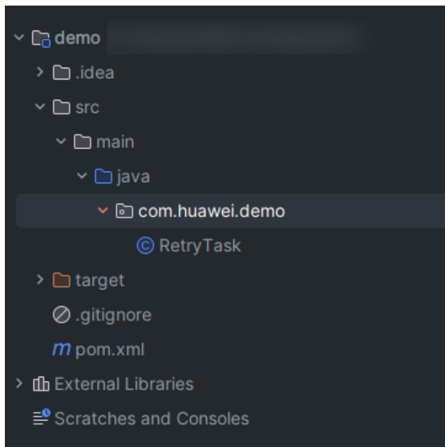
图 2-2 目录结构
