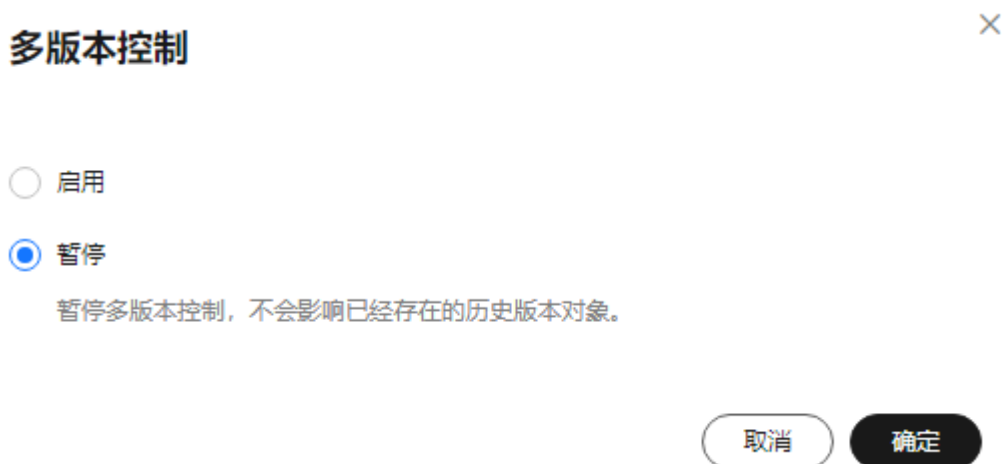
图 5-8 多版本控制
