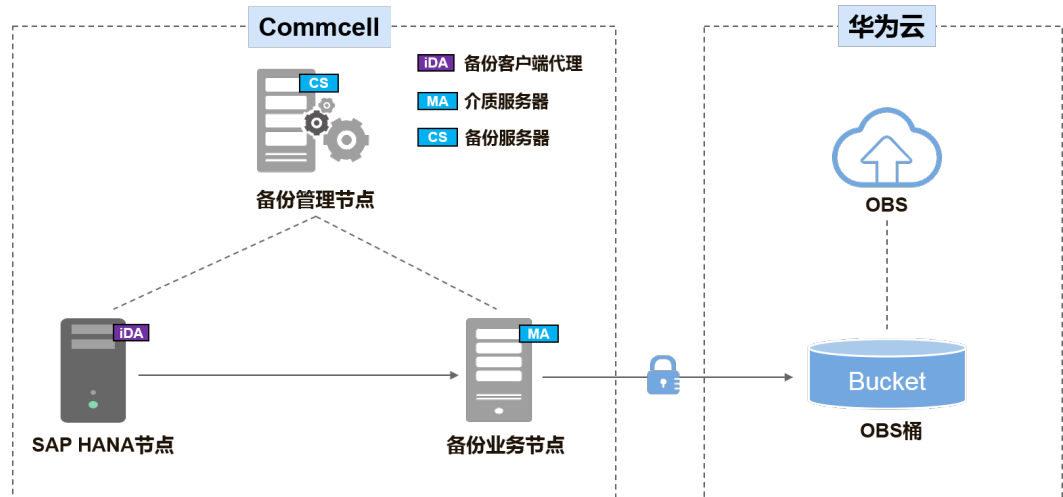
图 3-5 逻辑架构
