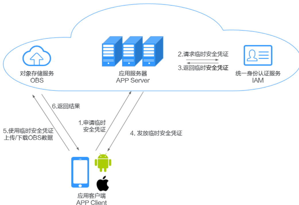
图 2-3 使用临时安全凭证直传 OBS 流程
