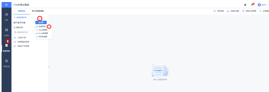
图 5-18 配置数据
