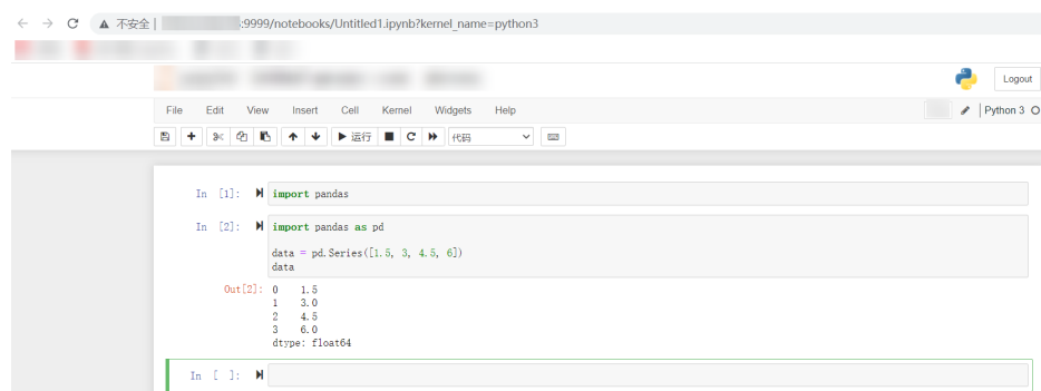
图 5-38 验证 pandas
