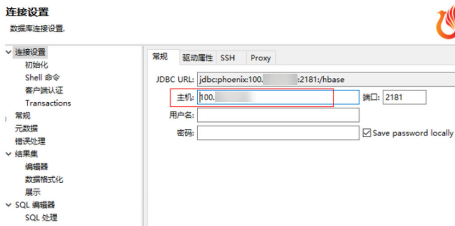
图 5-10 配置主机
