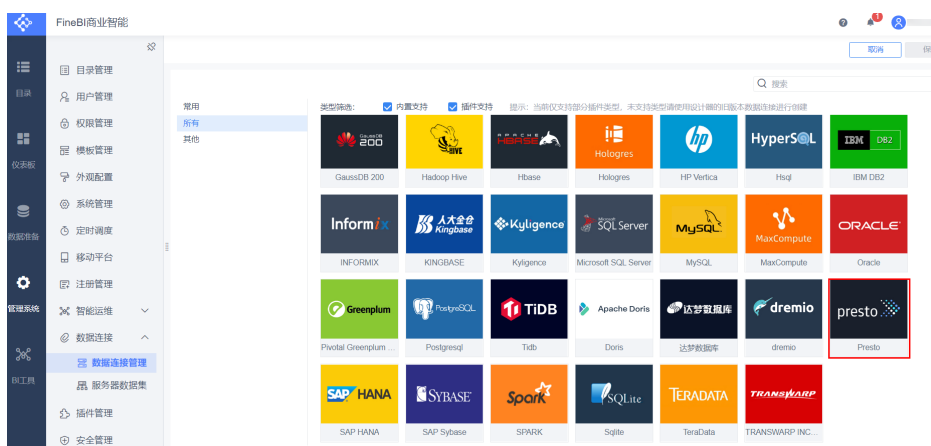
图 5-17 新建连接
