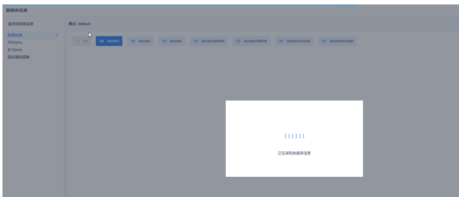
图 5-20 选择数据库
