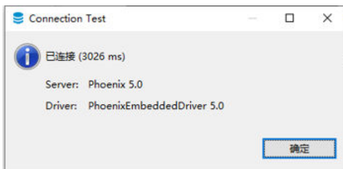
图 5-11 测试连接
