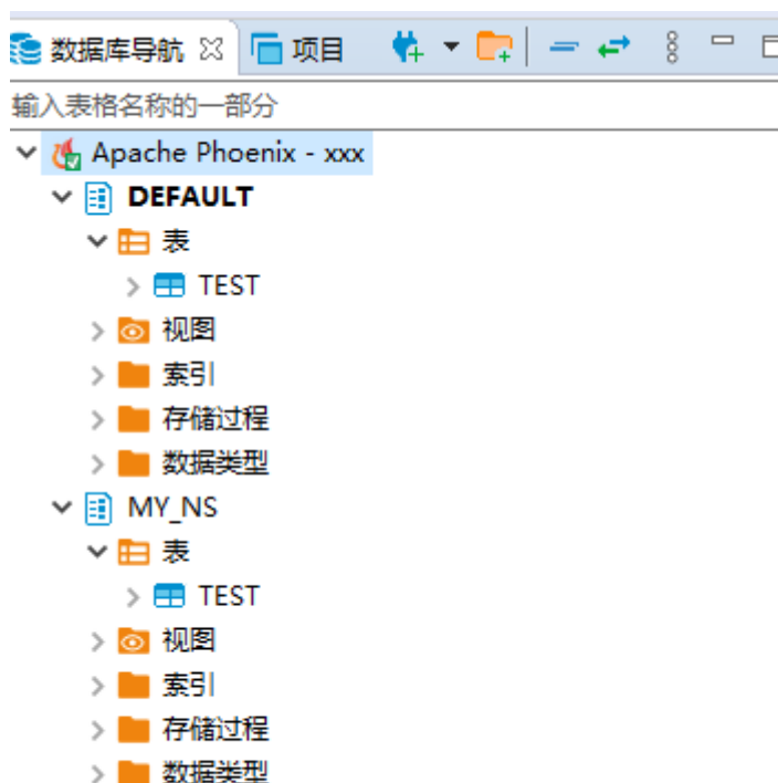
图 5-12 查看表
