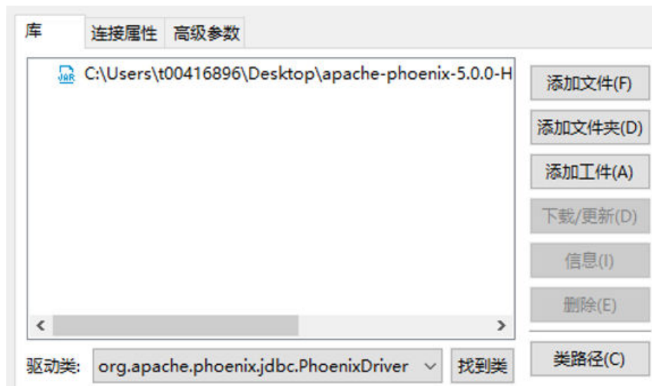
图 5-7 加载驱动类
