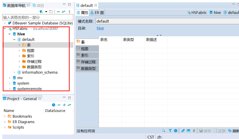
图 5-16 连接成功
