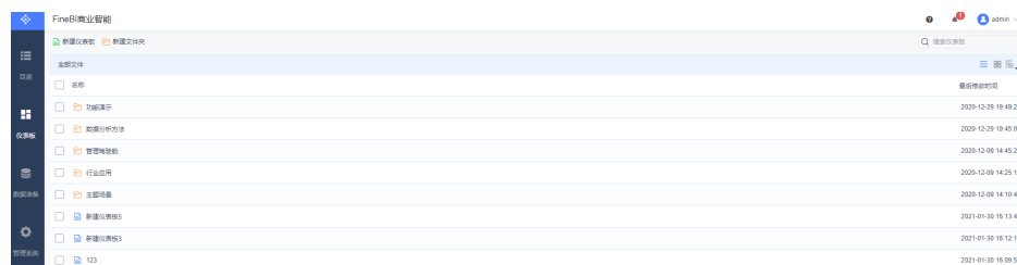
图 5-23 新建仪表板
