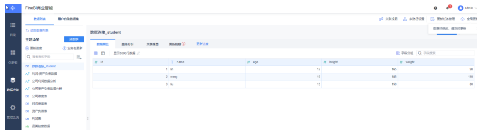
图 5-21 数据预览
