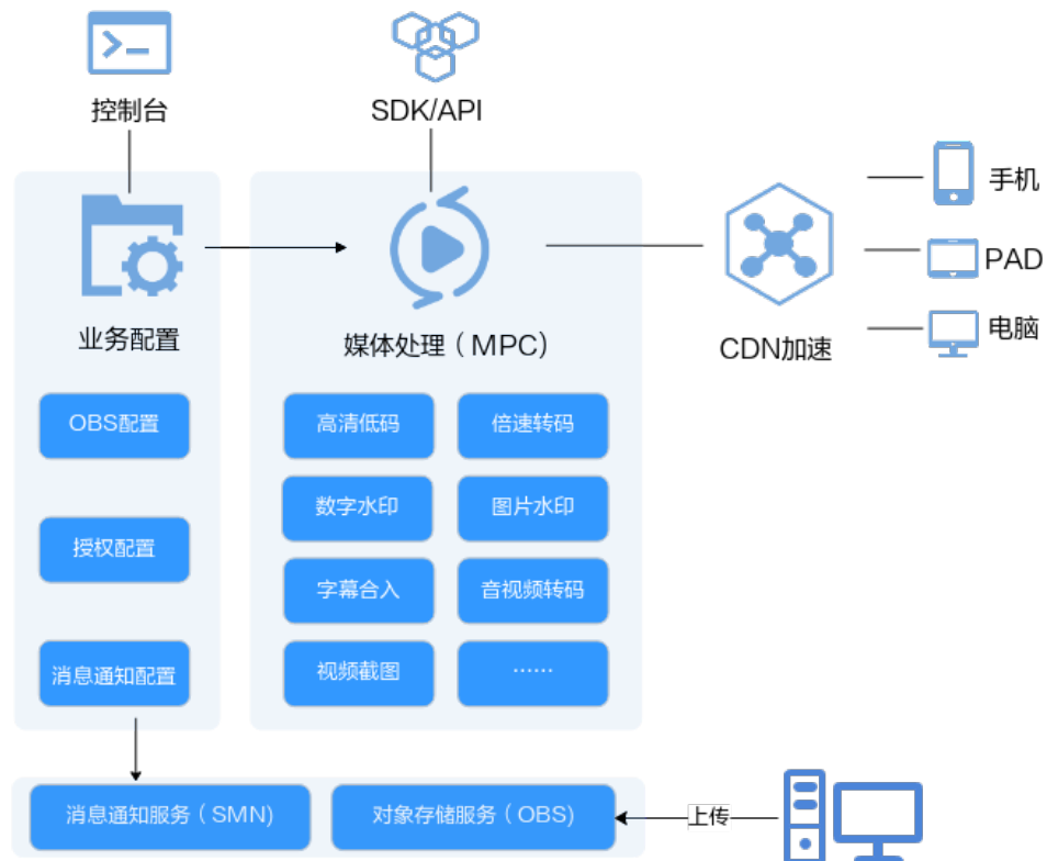
图 3-1 实现原理图
