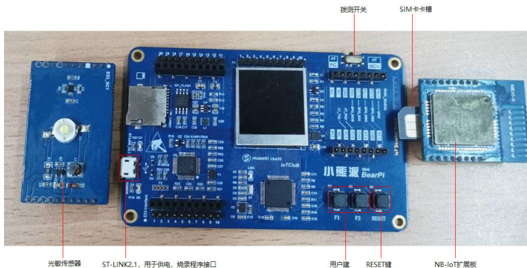
图 2-26 小熊派开发板
