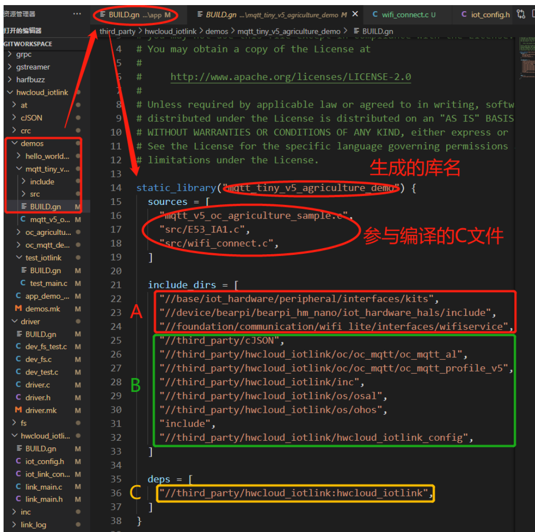
图 2-104 代码编译文件
