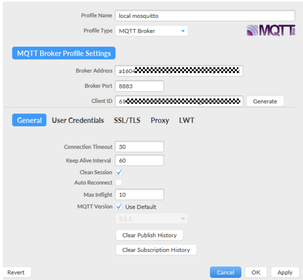
图 2-93 “General” 可以使用工具默认信息
