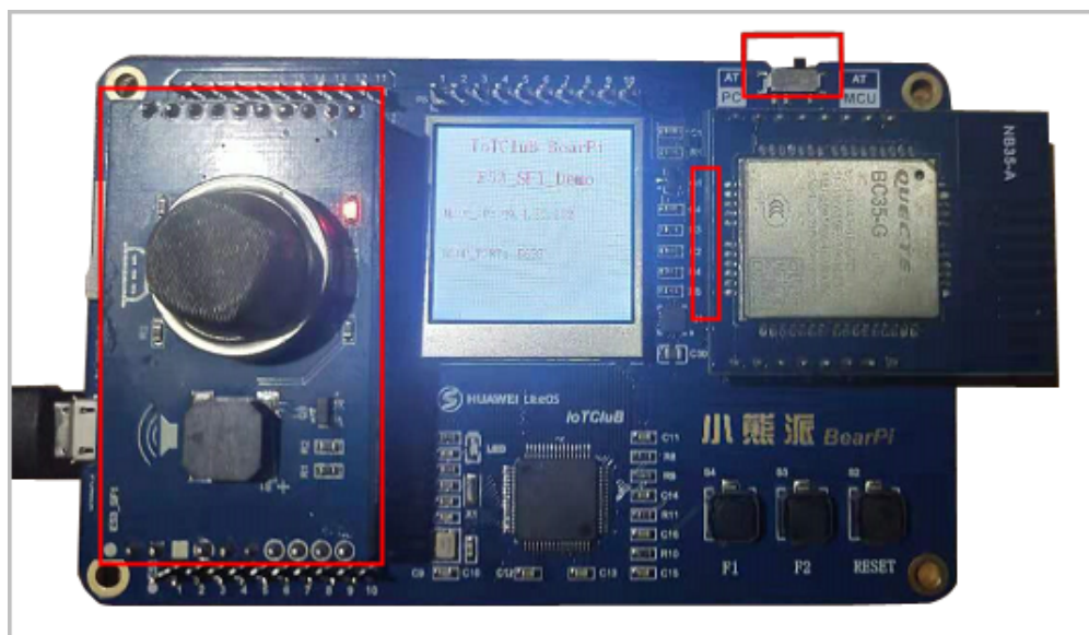
图 2-38 硬件连接
