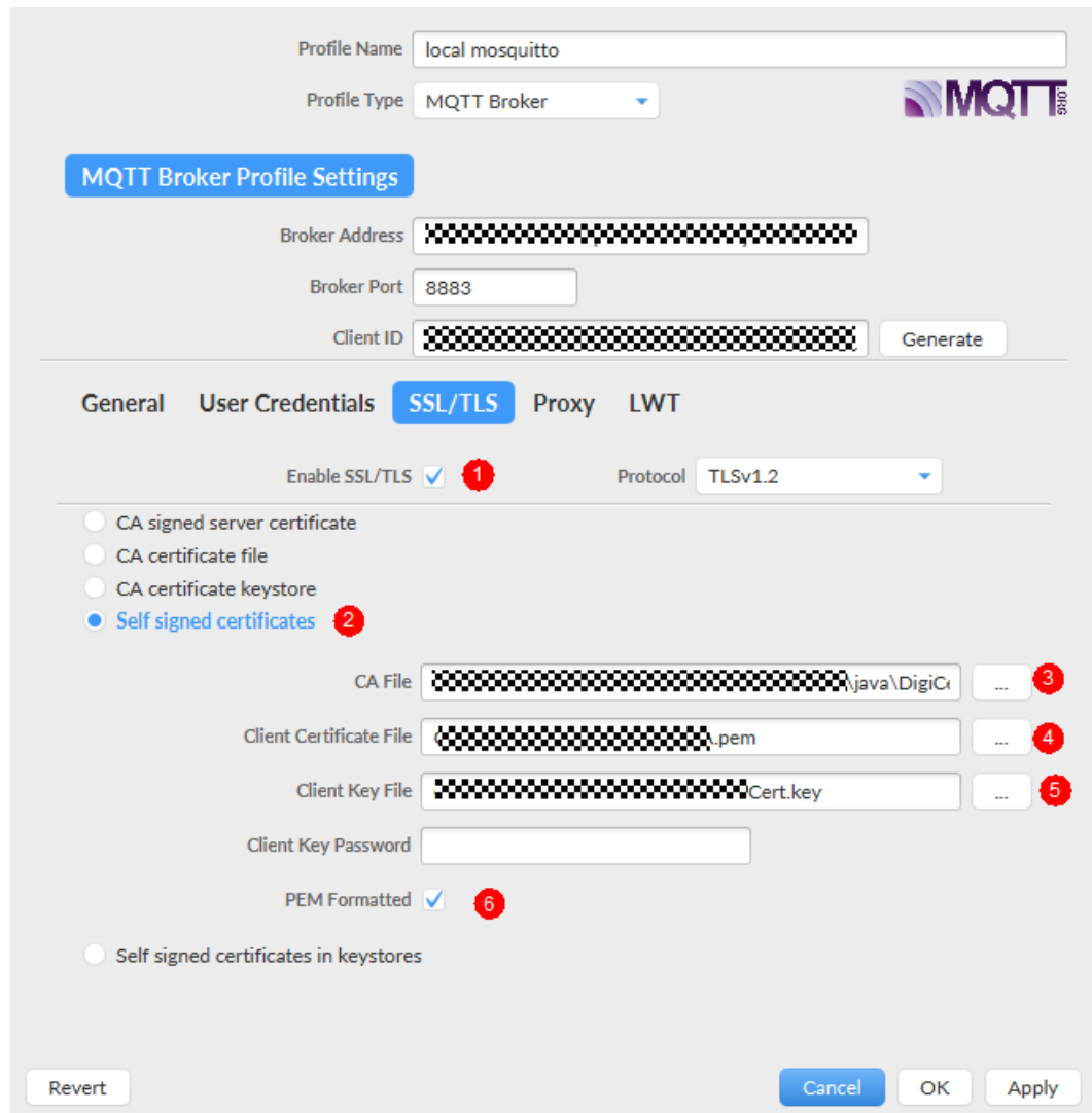
图 2-95 填写“SSL/TLS”相关参数
