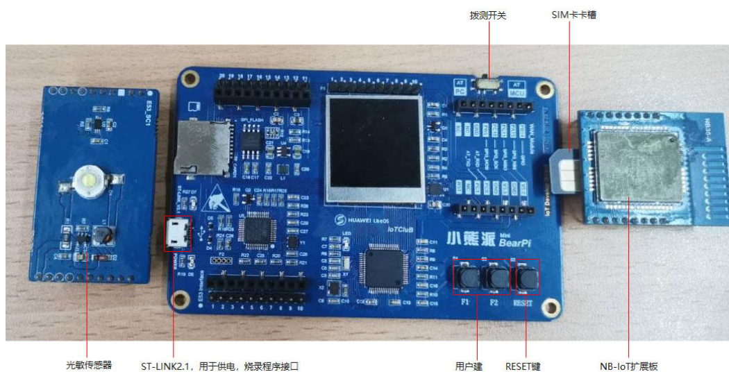
图 2-37 小熊派开发板
