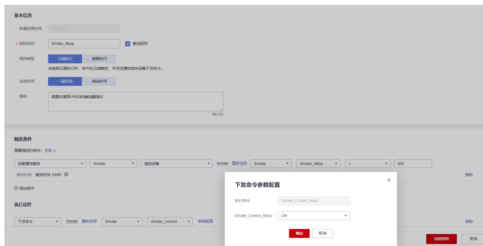
图 2-51 新建联动规则-Smoke_Beep
