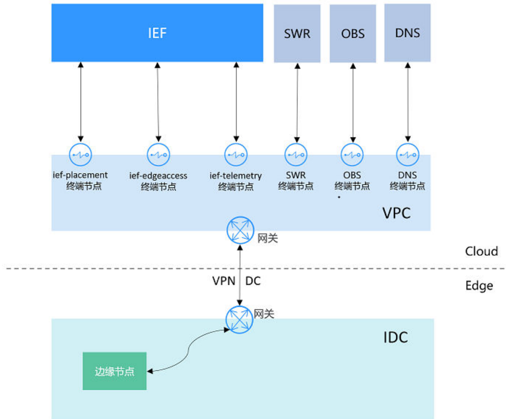
图 2-1 通过专线或 VPN 连接 IEF
