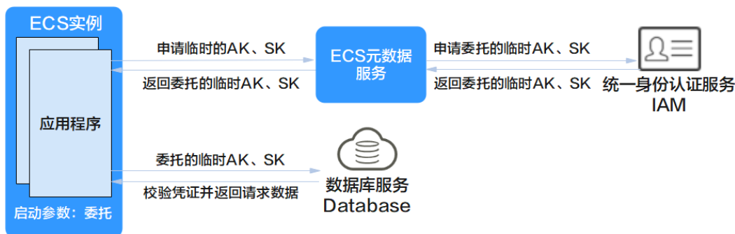
图 5-1 应用程序获取临时访问密钥
