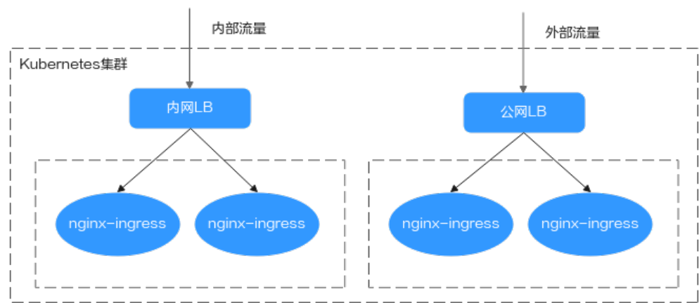
图 6-3 多个 Nginx Ingress 应用场景
