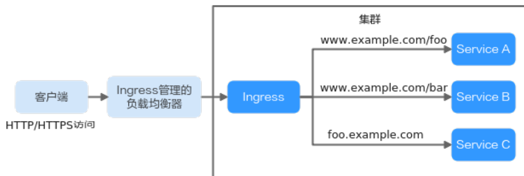
图 6-2 Ingress 示意图
