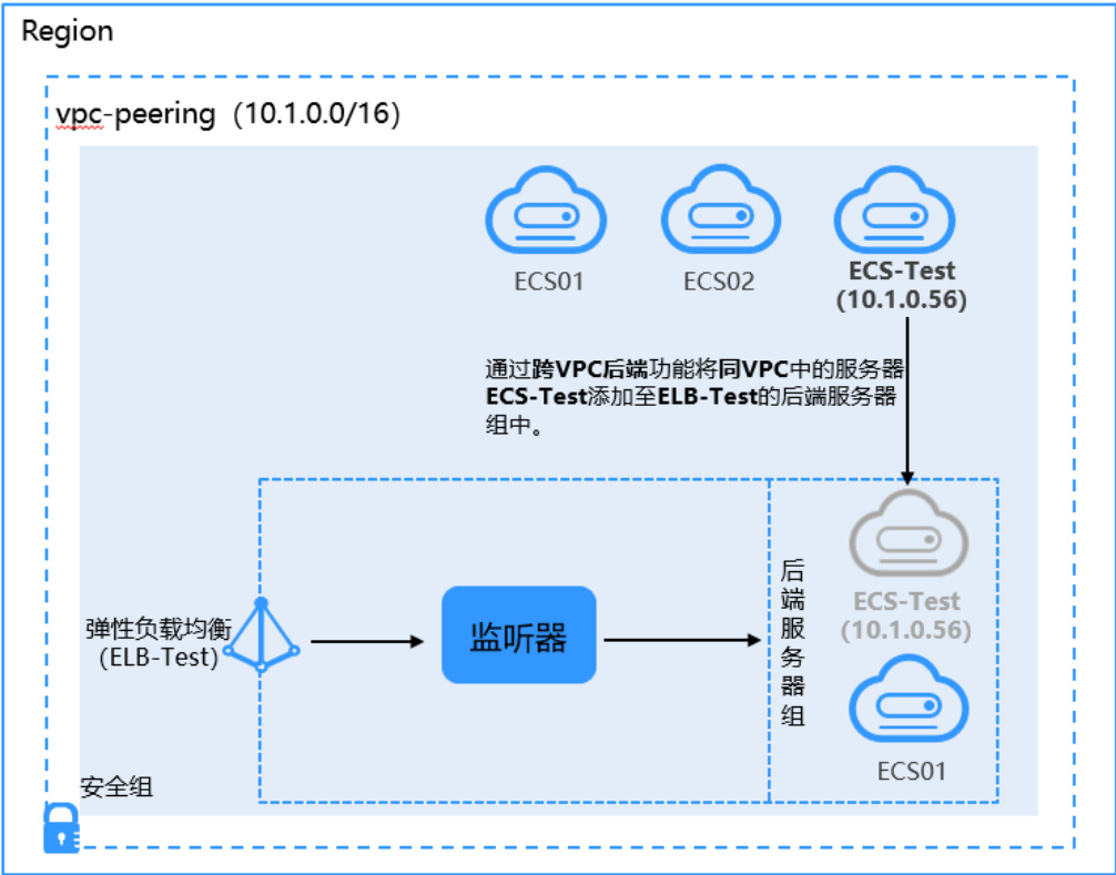
图 1-13 使用 IP 类型后端功能添加同 VPC 的 ECS 至 ELB
