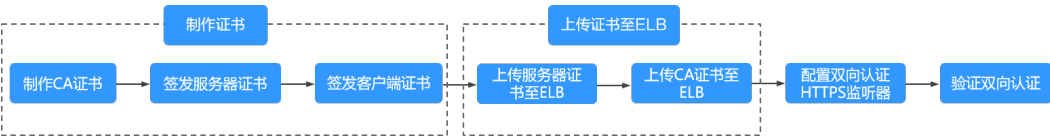
图 3-10 配置 HTTPS 业务双向认证操作流程
