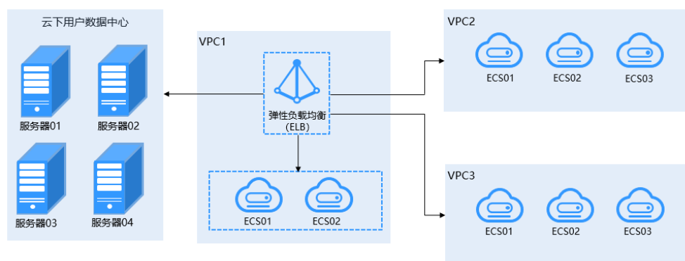
图 1-6 添加云上、云下多台后端服务器至 ELB
