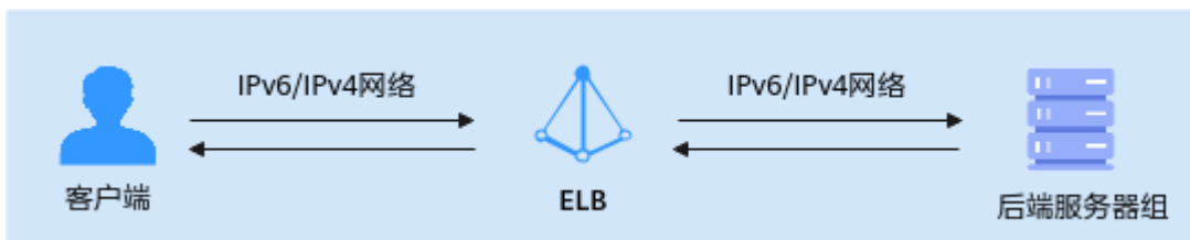
图 4-21 四层（TCP 和 UDP 协议）ELB 开启 IPv4/IPv6 地址转换业务架构图
