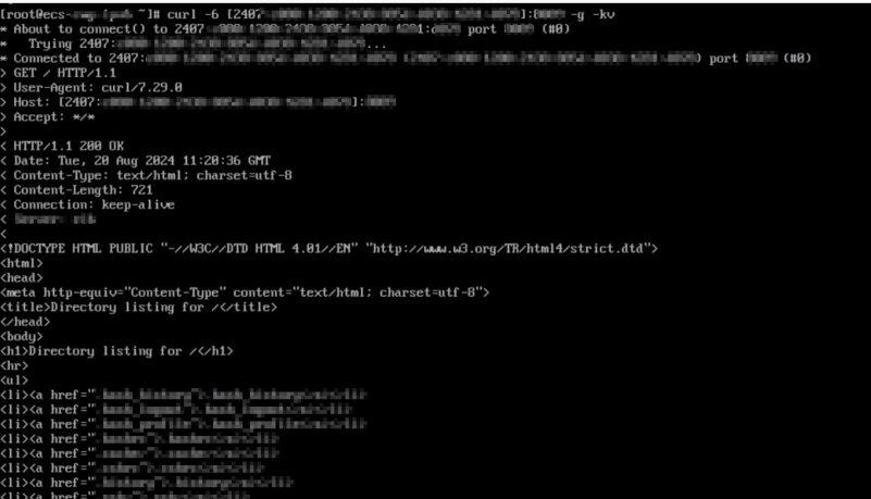
图 4-27 验证 Web 类服务应用的连通性
