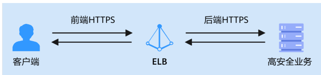
图 2-1 全链路 HTTPS
