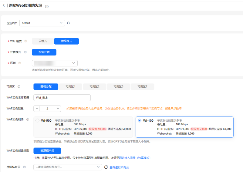
图 2-11 创建独享模式 WAF 实例
