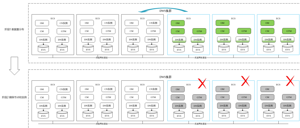
图 8-7 集群缩容
