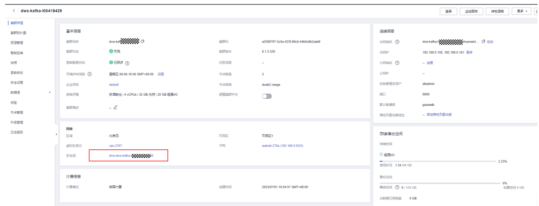
图 2-26 DWS 安全组
