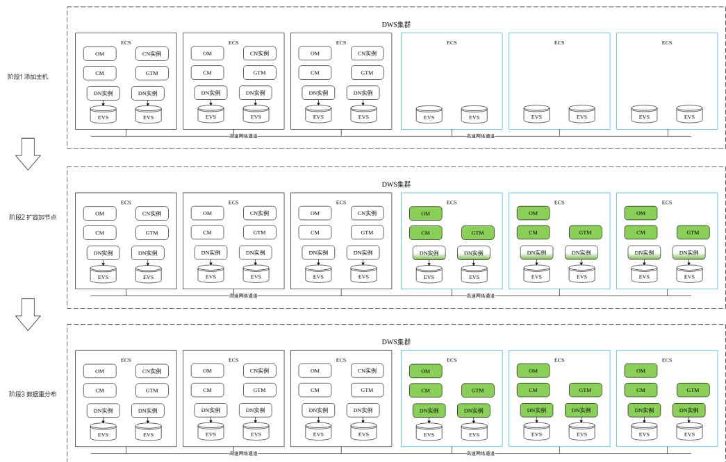
图 8-5 集群扩容
