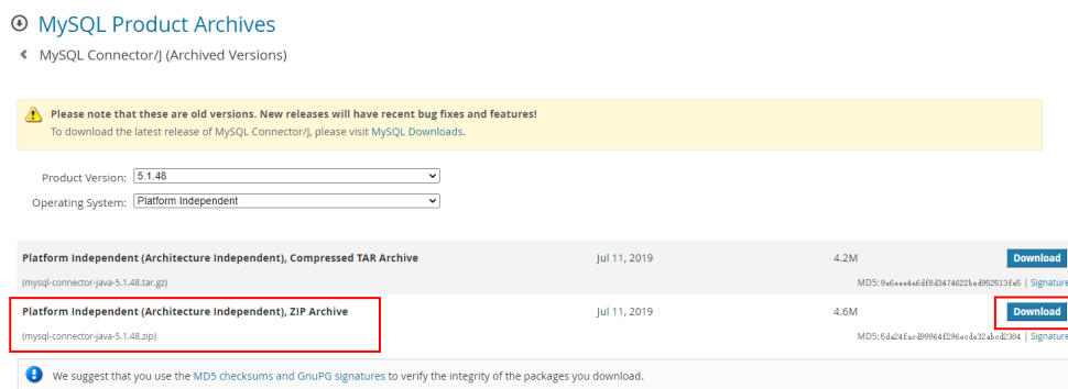
图 2-9 下载驱动
