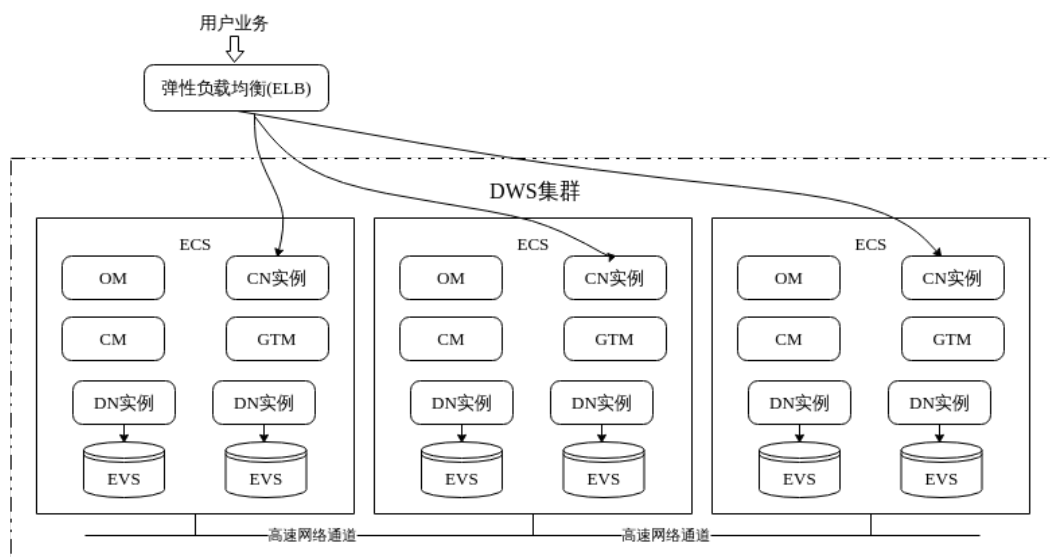
图 8-1 集群拓扑
