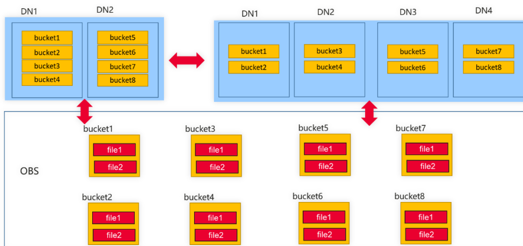
图 4-3 Bucket 存储
