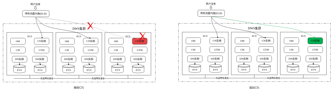
图 8-8 增删 CN
