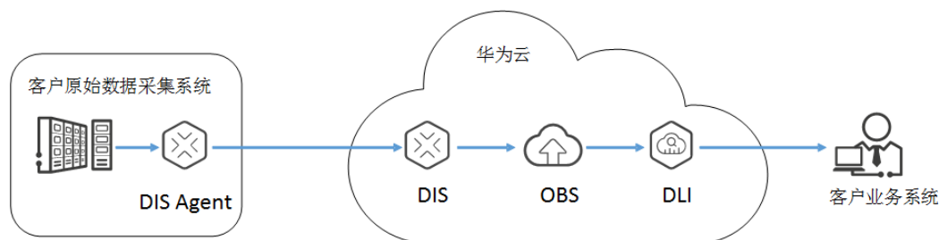
图 2-1 业务流程图
