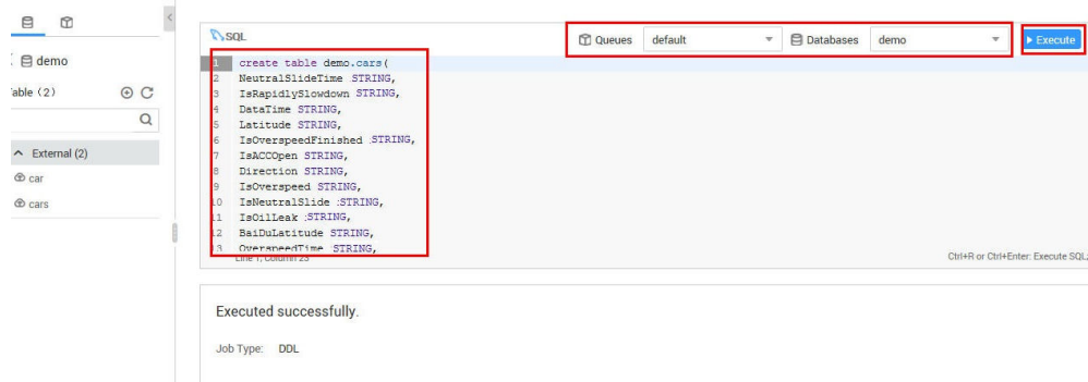
图 2-3 创建表
