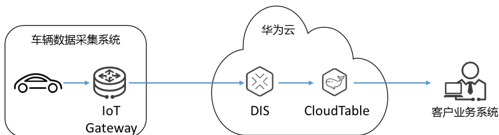
图 1-1 业务流程图
