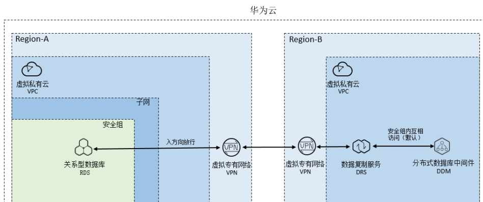
图 11-1 VPN 场景
