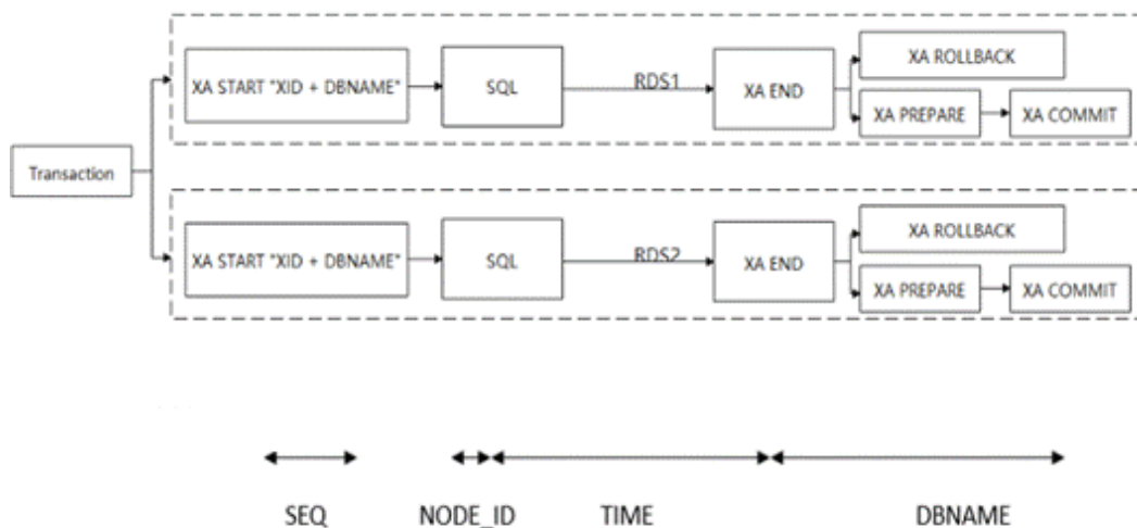
图 5-1 分布式事务执行流程
