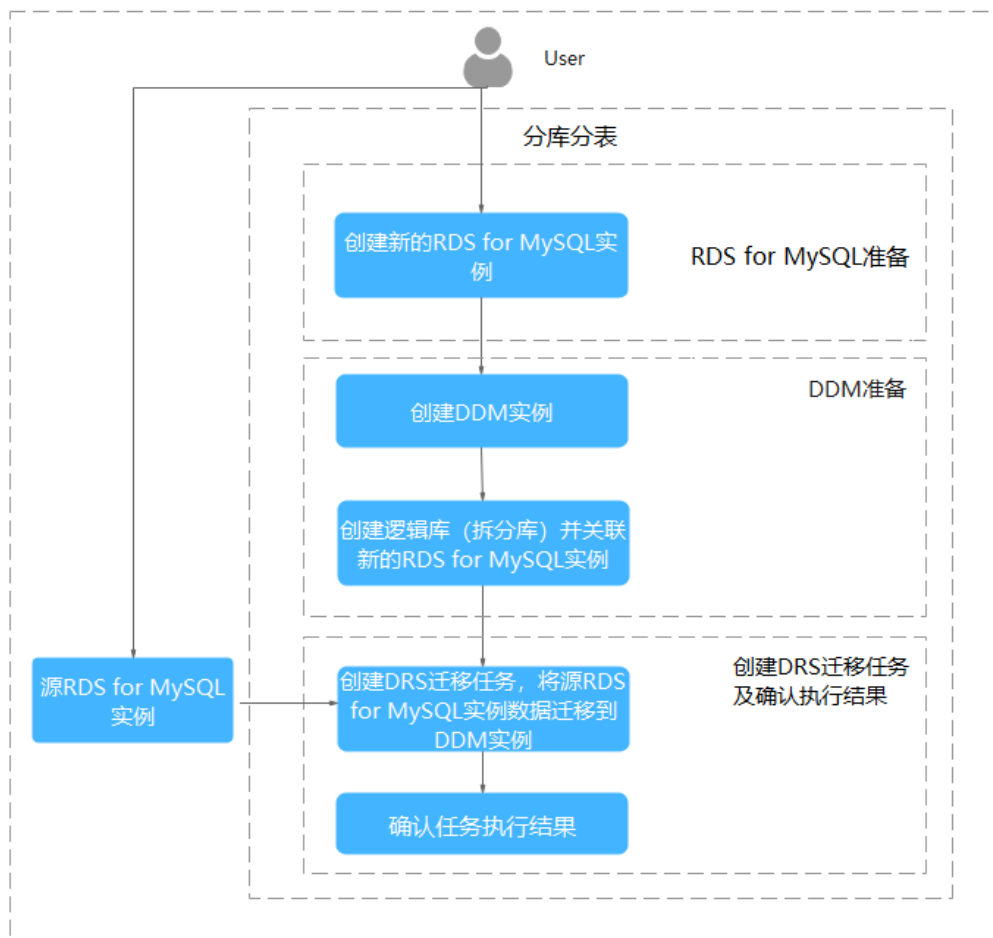
图 12-1 流程图
