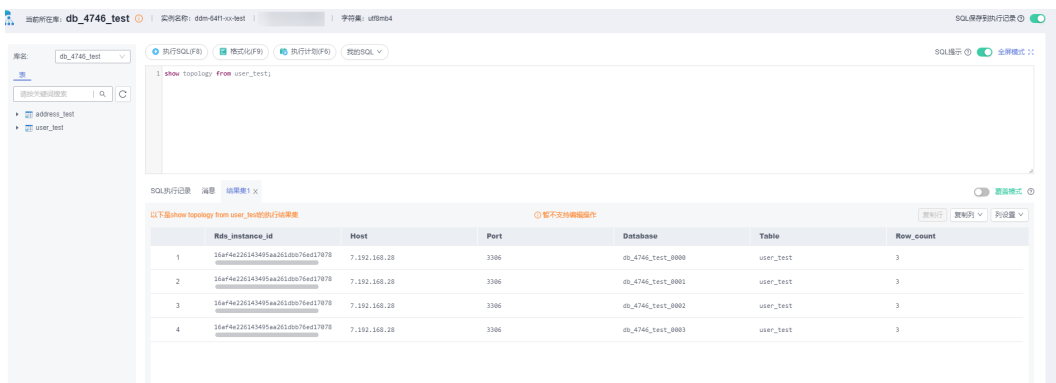
图 12-26 广播表 user_test
