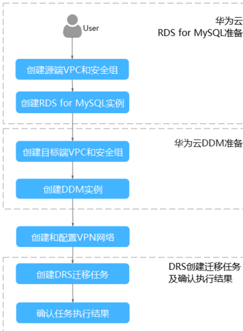
图 11-2 流程图
