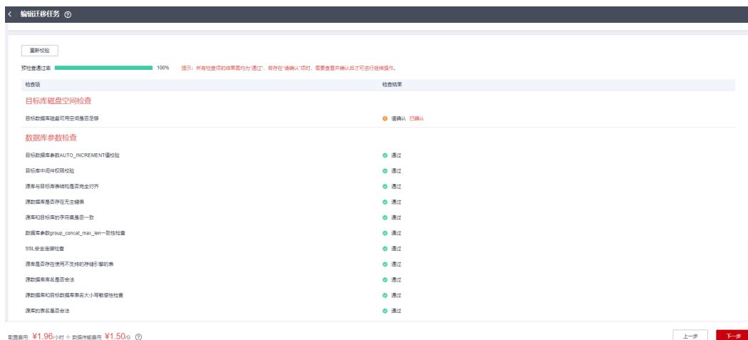
图 12-22 预检查
