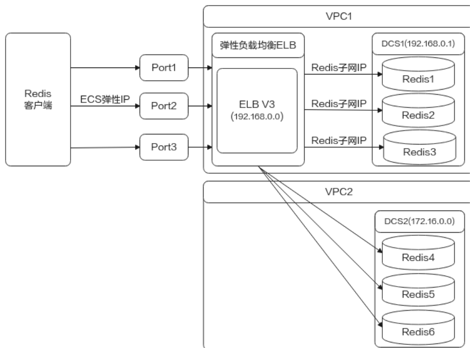
图 12-1 ELB 访问 DCS 流程图
