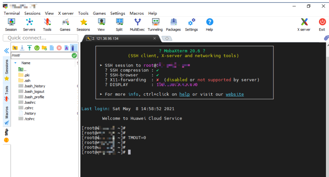
图 11-2 输入 TMOUT=0
