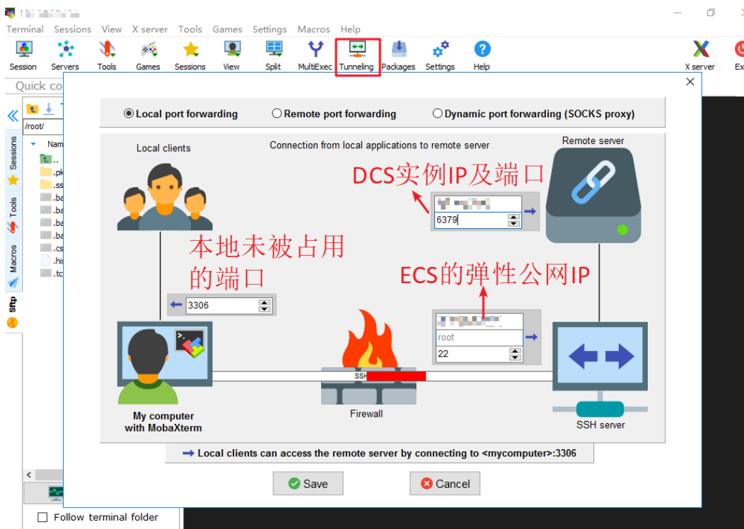
图 11-3 创建隧道
