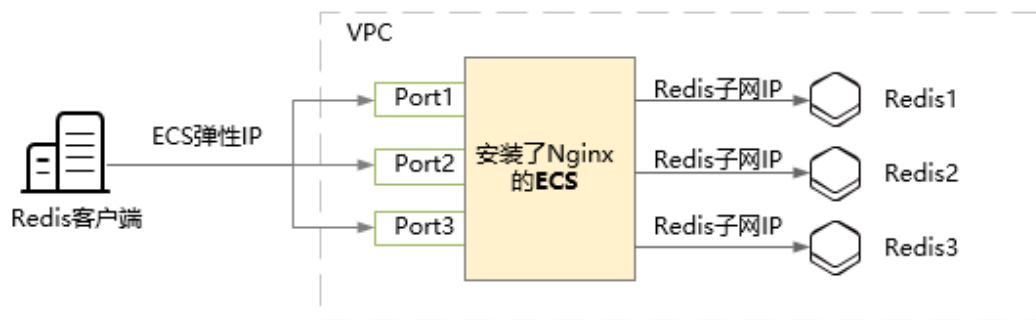
图 10-1 通过 Nginx 访问 VPC 内 DCS Redis
