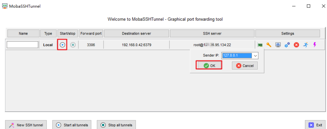
图 11-4 启动隧道
