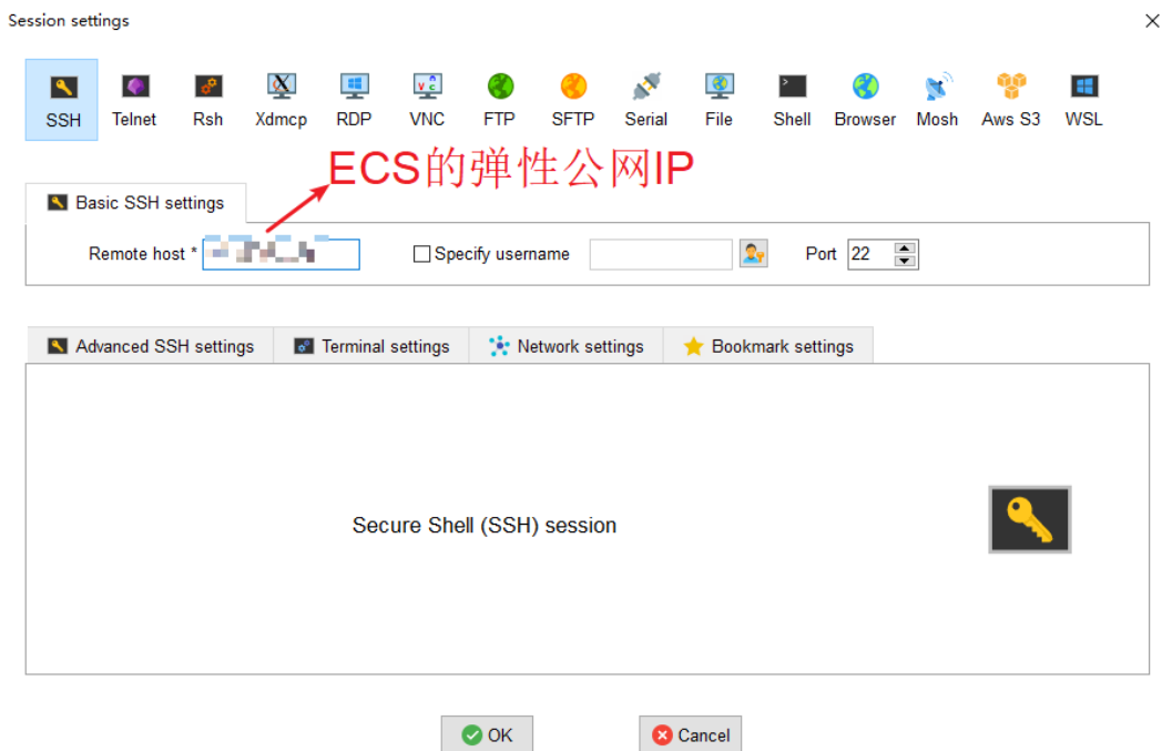
图 11-1 连接 ECS
