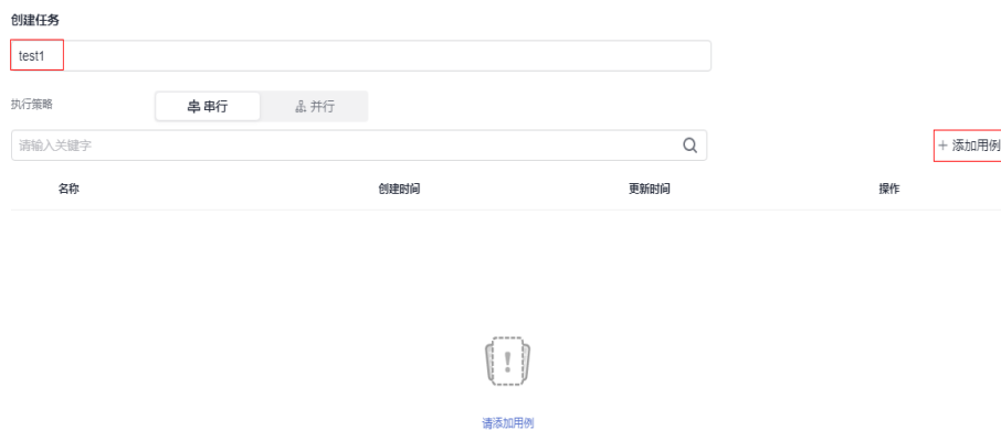
图 2-7 添加用例
