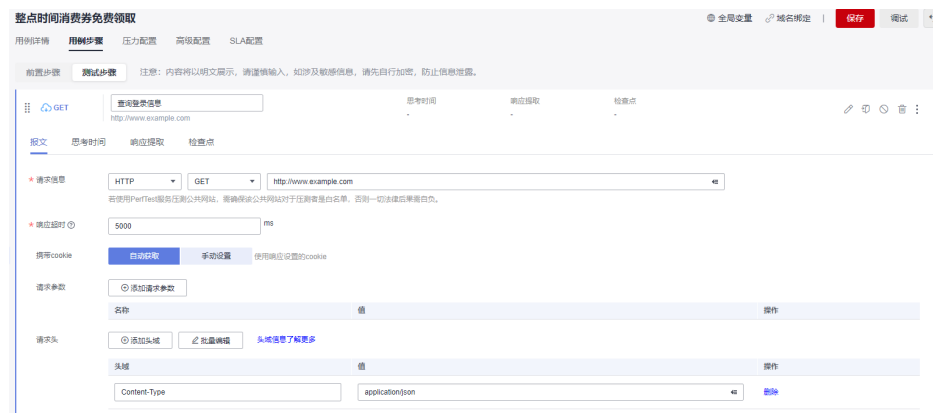
图 2-6 修改参数
