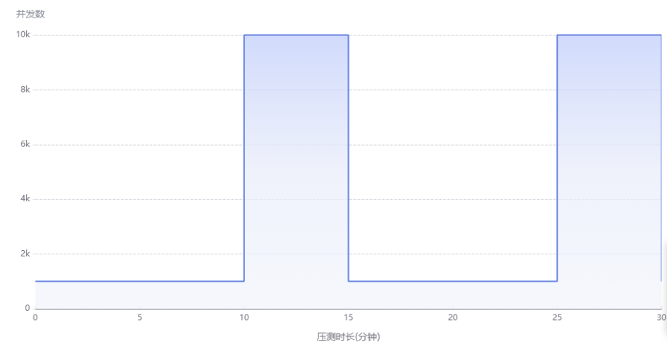
图 1-4 模型样例 4
