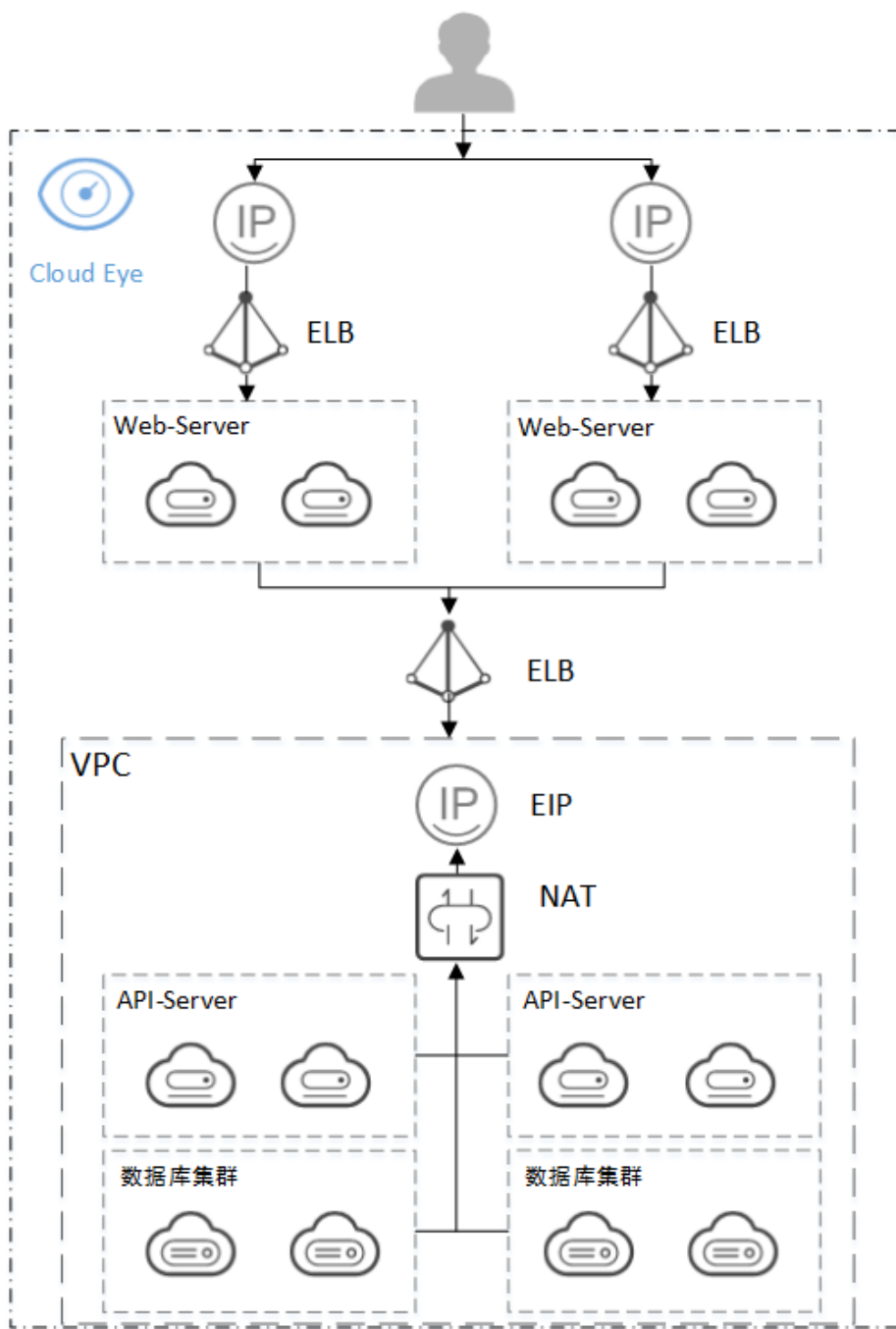
图 3-1 众包平台架构图
