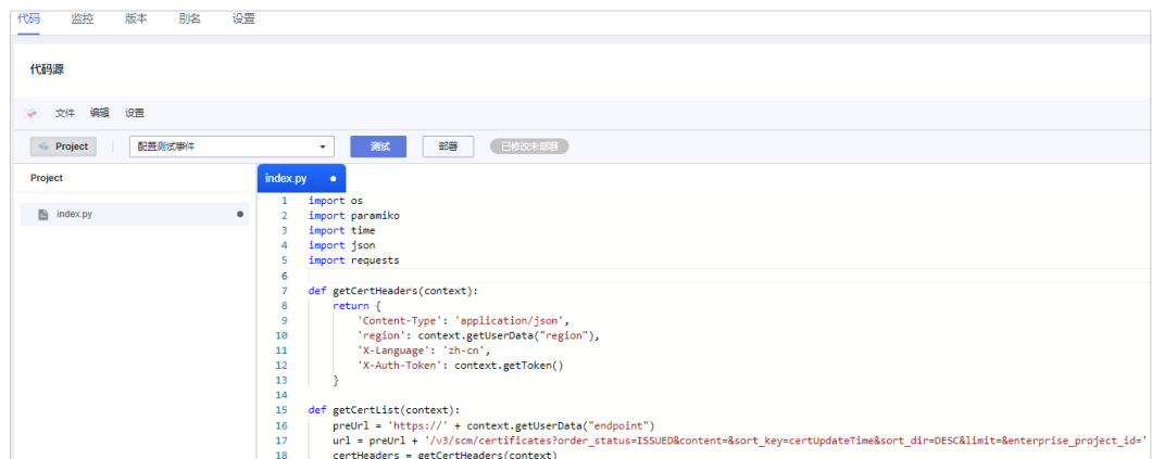
图 2-26 添加代码
