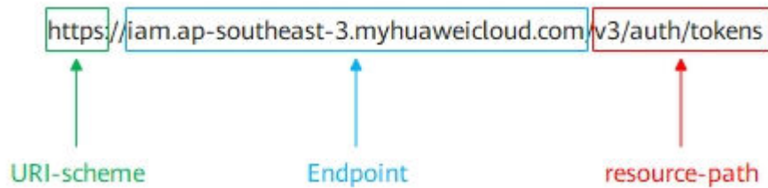
图 3-1 URI 示意图
