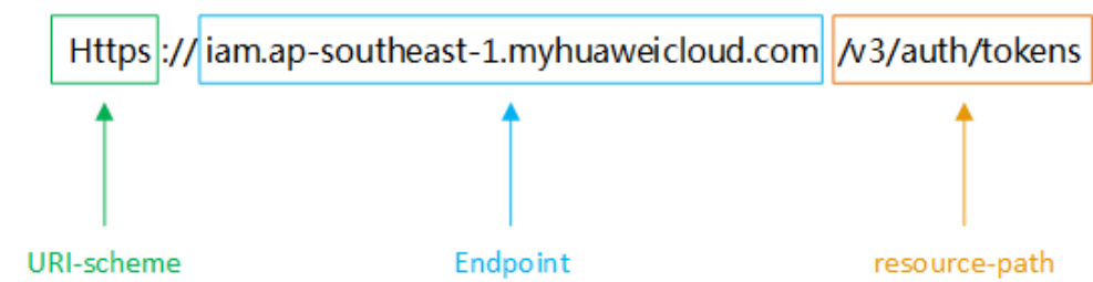
图 3-1 URI 示意图
