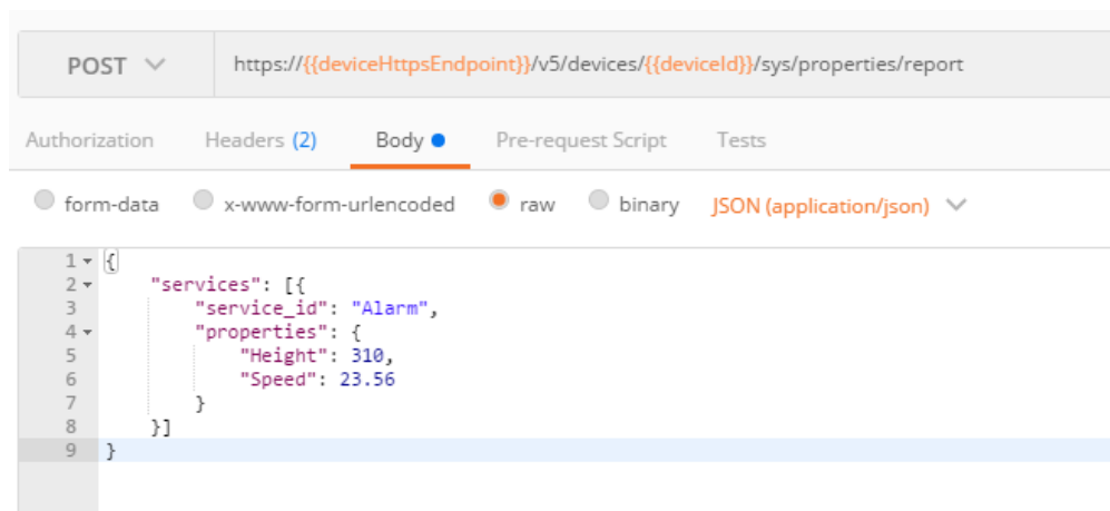
图 3-4 上报属性
