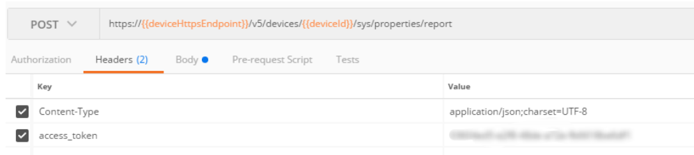
图 3-3 上报属性
