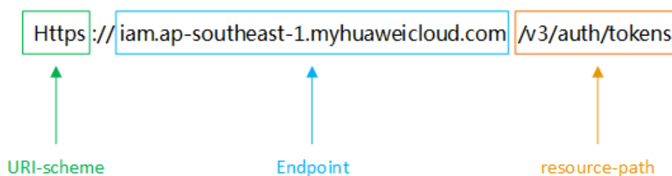
图 3-2 URI 示意图
