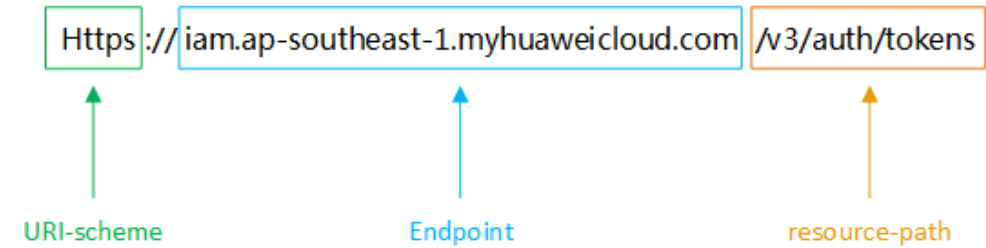
图 3-2 URI 示意图
