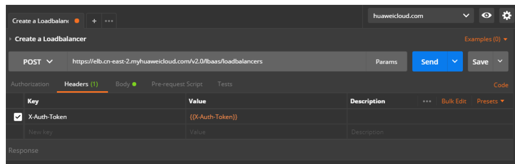
图 10-15 设置请求消息头-创建白名单
