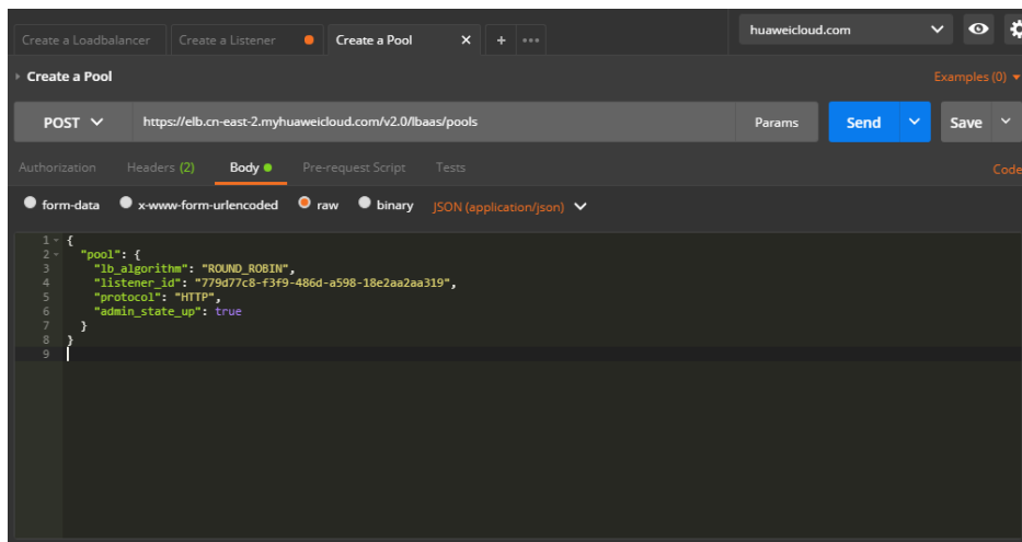
图 10-10 填写请求消息体-创建后端云服务器组
