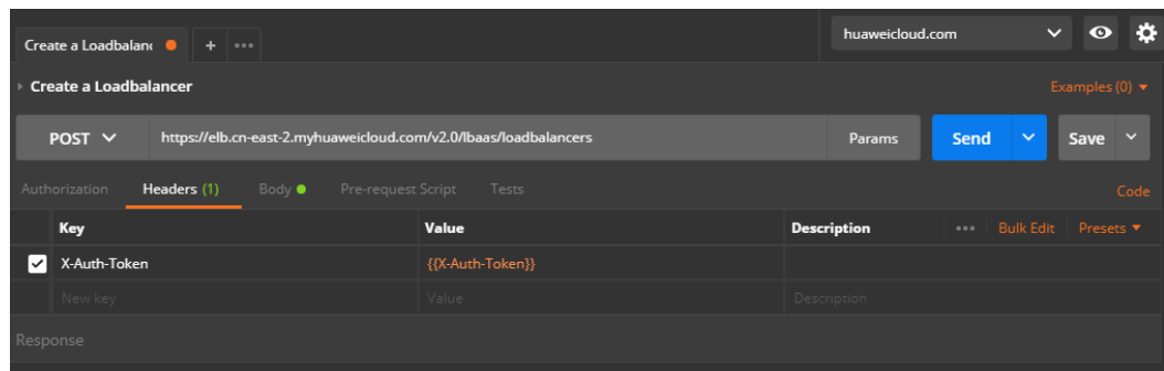
图 10-13 设置请求消息头-创建健康检查
