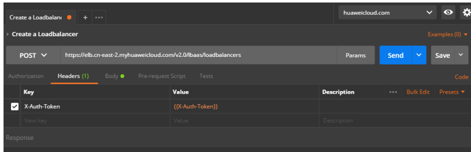
图 10-9 设置请求消息头-创建后端云服务器组
