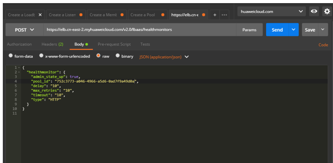
图 10-14 填写请求消息体-创建健康检查
