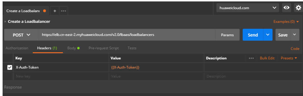
图 10-17 设置请求消息头-创建 SSL 证书
