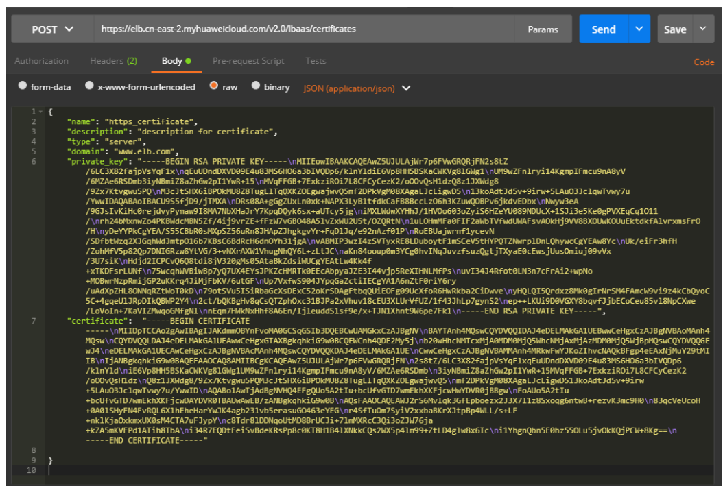
图 10-18 填写请求消息体-创建 SSL 证书
