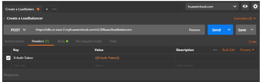
图 10-1 设置请求消息头-创建负载均衡器
