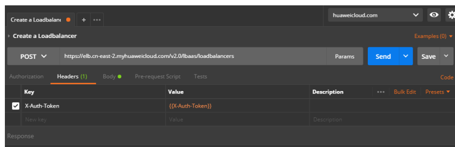
图 10-11 设置请求消息头-添加后端云服务器组
