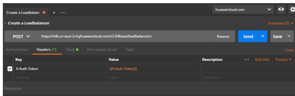
图 10-5 设置请求消息头-创建公网负载均衡器
