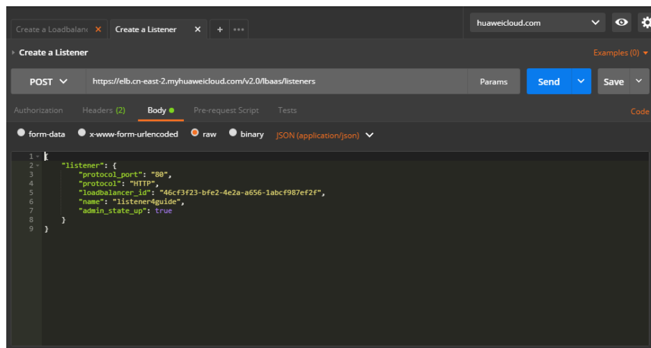
图 10-8 填写请求消息体-创建监听器
