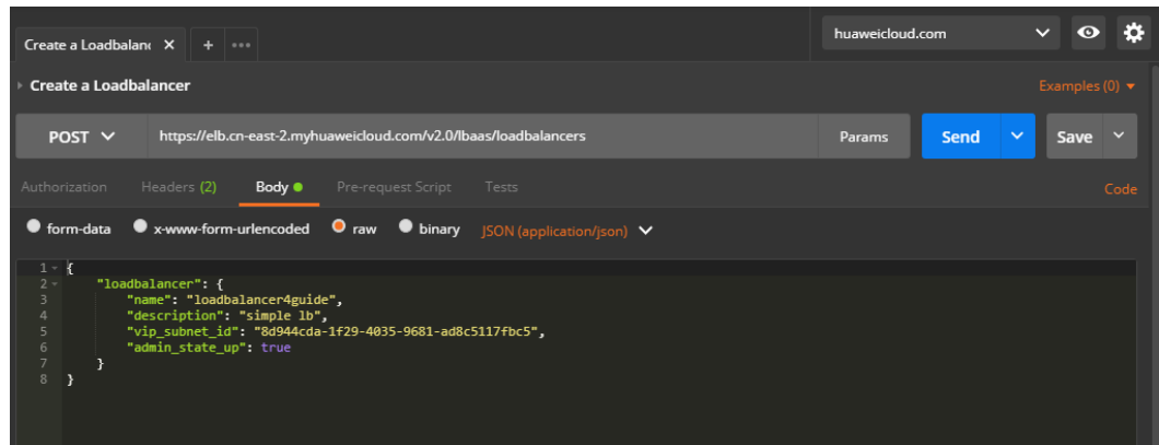
图 10-2 填写请求消息体-创建负载均衡器
