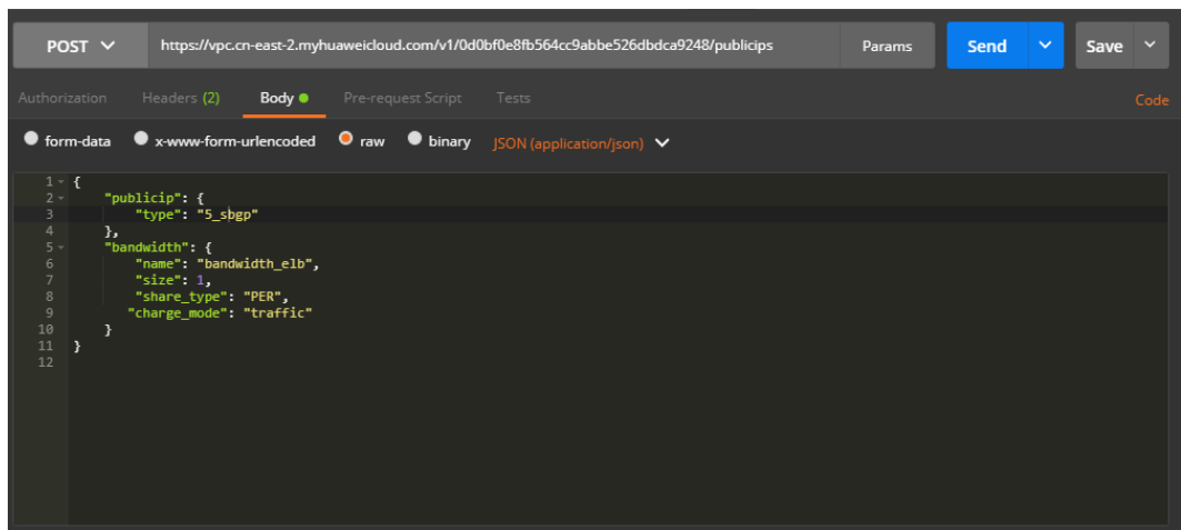
图 10-4 填写请求消息体-创建公网负载均衡器
