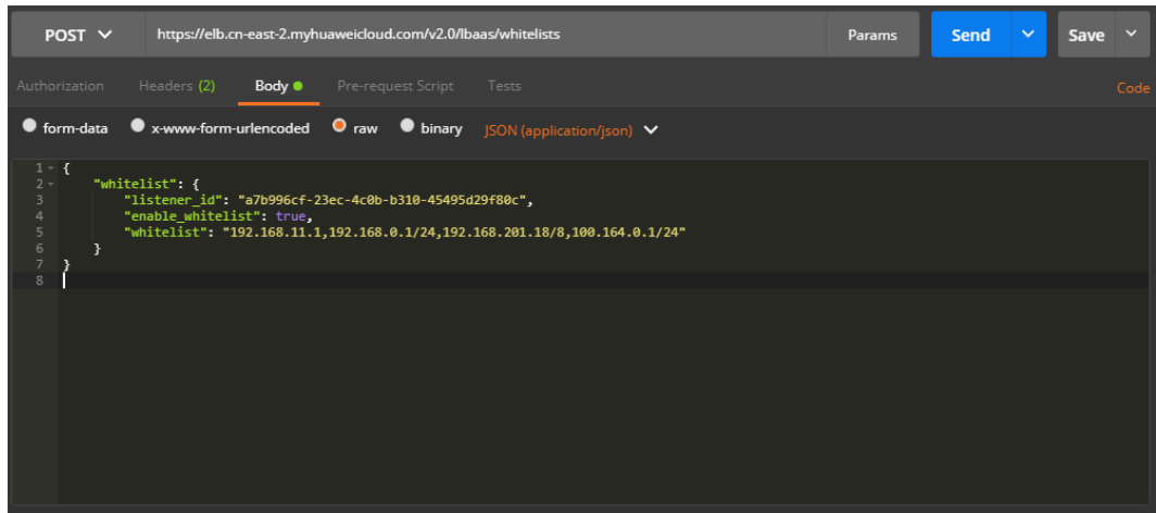
图 10-16 填写请求消息体-创建白名单
