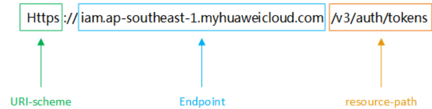
图 3-1 URI 示意图
