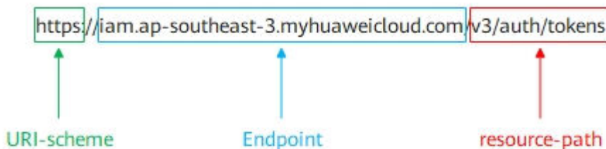
图 3-1 URI 示意图
