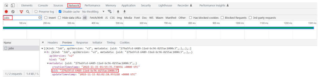
图 8-7 获取 job_id
