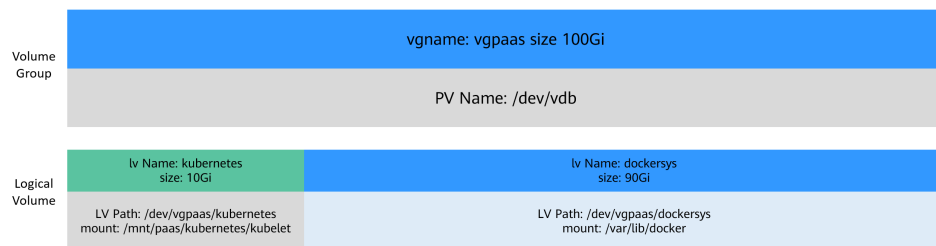
图 8-14 OverlayFS 类型容器引擎空间分配
