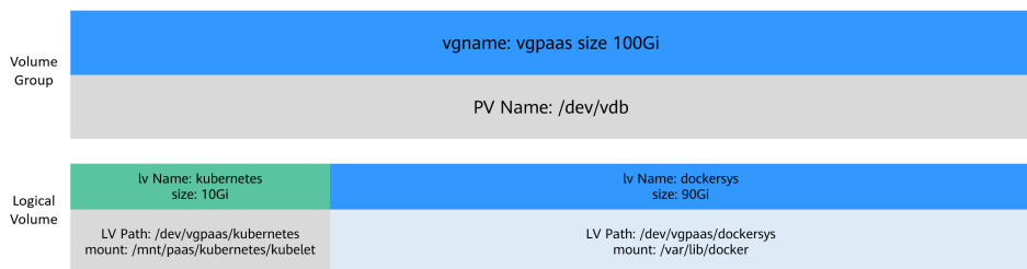
图 8-15 OverlayFS 类型容器引擎空间分配
