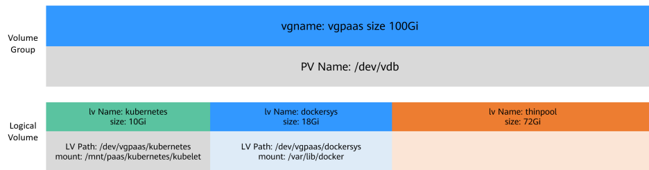
图 8-13 Device Mapper 类型容器引擎空间分配
