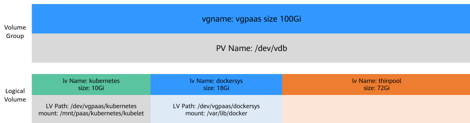
图 8-14 Device Mapper 类型容器引擎空间分配
