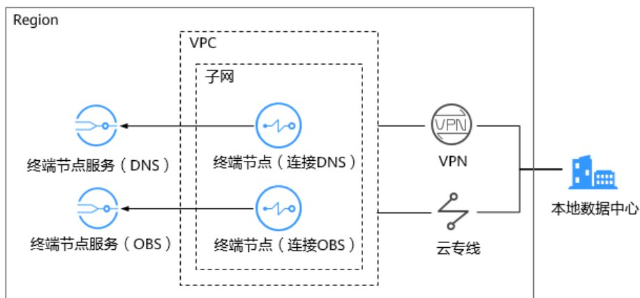
图 2-6 本地数据中心访问 OBS（内网）
