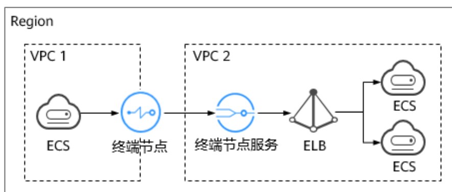
图 1-3 跨 VPC 连接场景示意图
