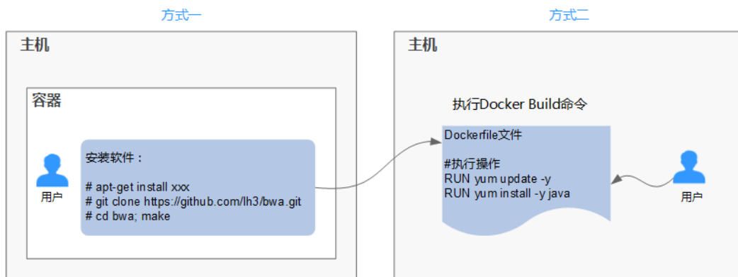
图 9-3 使用 Dockerfile 方式构建
